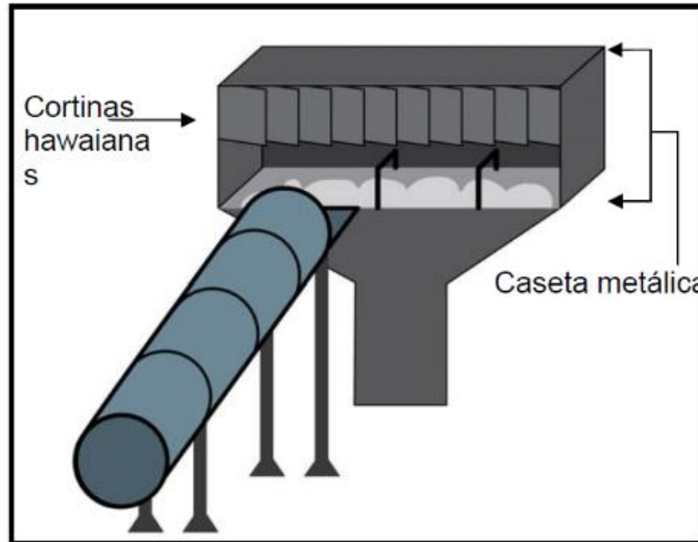
Figura 4. Tolva Secundaria
