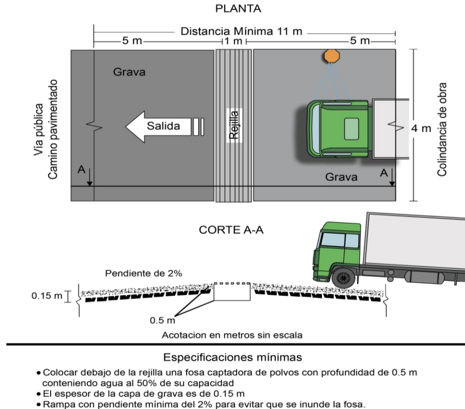
Figura 1 Esquema del Dispositivo de control de salida.
