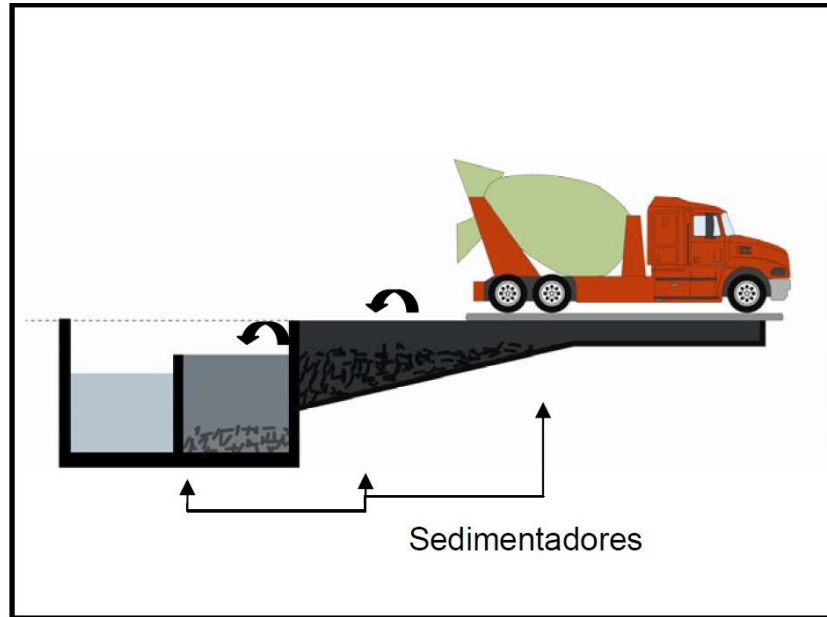
Figura 2. Fosas de lavado y decantación Fuente: NADF-021-AMBT-2011,
