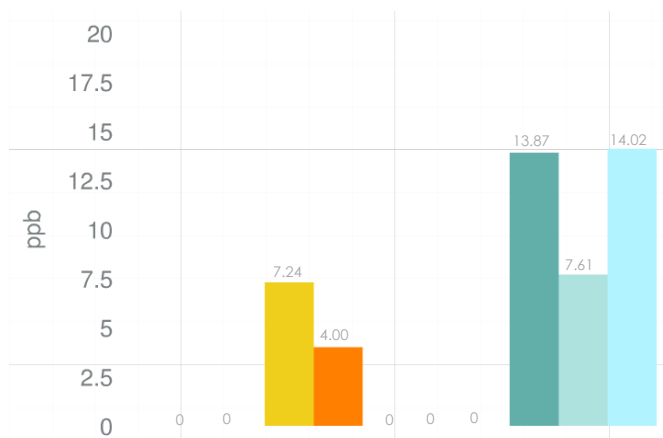
Figura 18: Promedios de concentración de bióxido de nitrógeno por zona en el Área Metropolitana de Monterrey en el mes de Abril de 2016.
