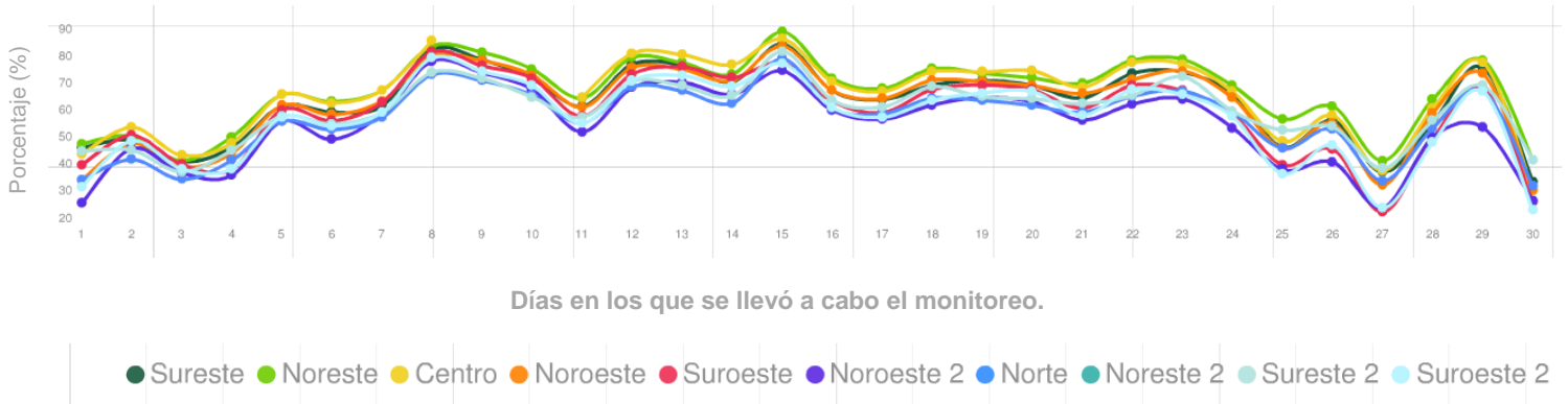
Figura 5: Humedad relativa diaria por zona en el Área Metropolitana de Monterrey, Abril 2016.
