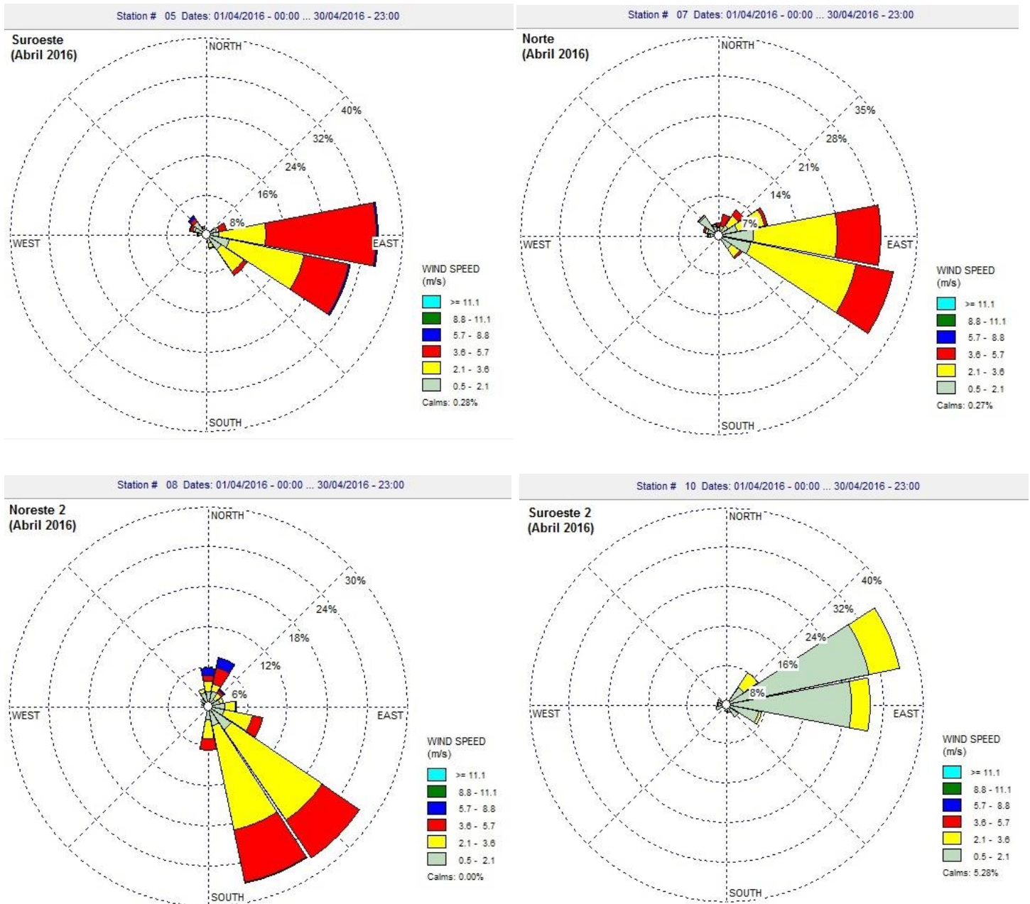
Figura 11: Velocidad del viento por zona en el Área Metropolitana de Nuevo León.
