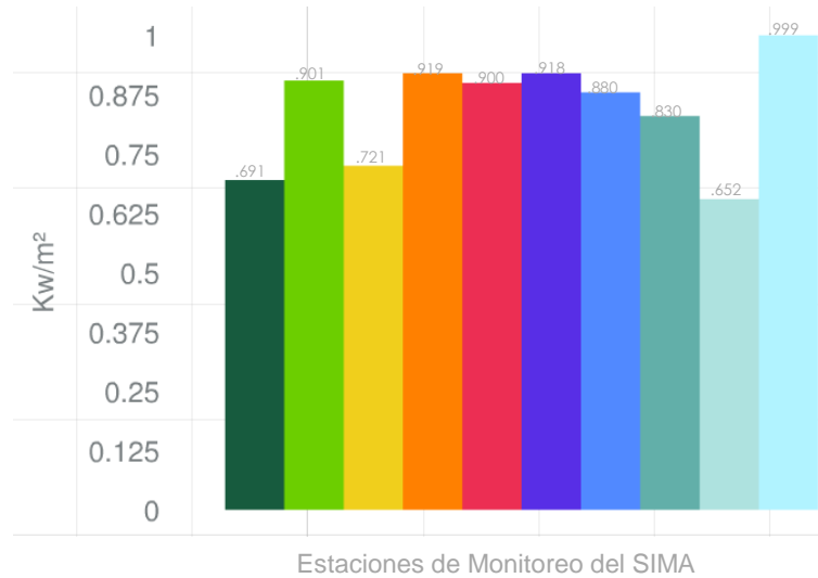
Figura 10: Radiación solar máxima por zona en el Área Metropolitana de Monterrey en el mes de Abril de 2016.
