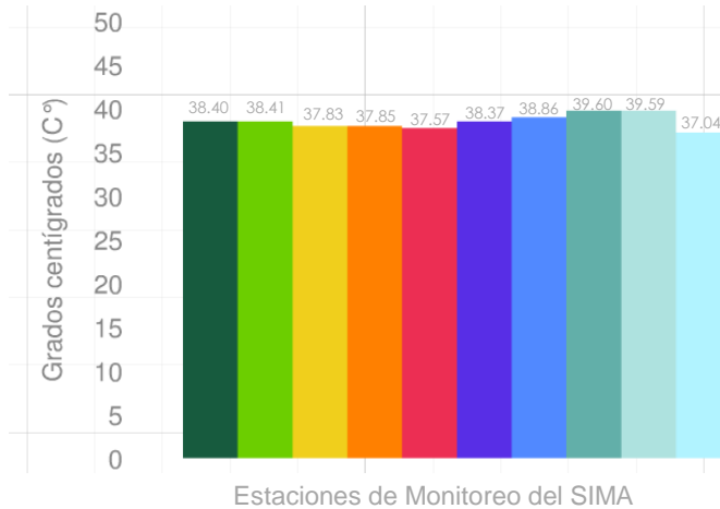
Figura 3: Temperatura máxima alcanzada por zona en el Área Metropolitana de Monterrey en el mes de Abril 2016
