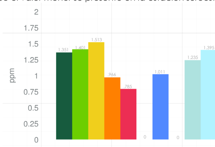
Figura 14: Promedios de concentración de monóxido de carbono por zona en el Área Metropolitana de Monterrey en el mes de Abril de 2016.
