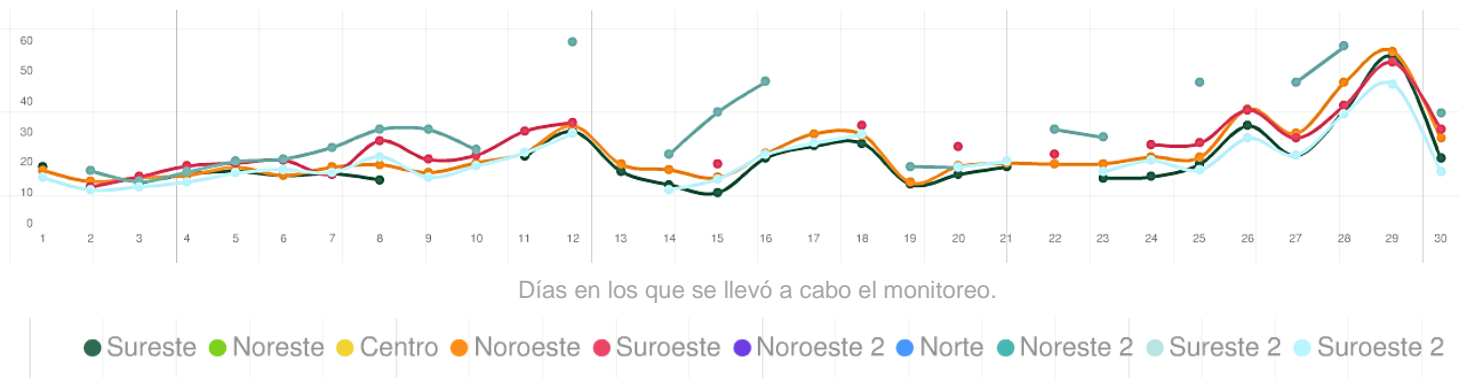
Figura 23: Concentración promedio diaria de PM 2.5 ) por zona en el Área Metropolitana de Nuevo León.
