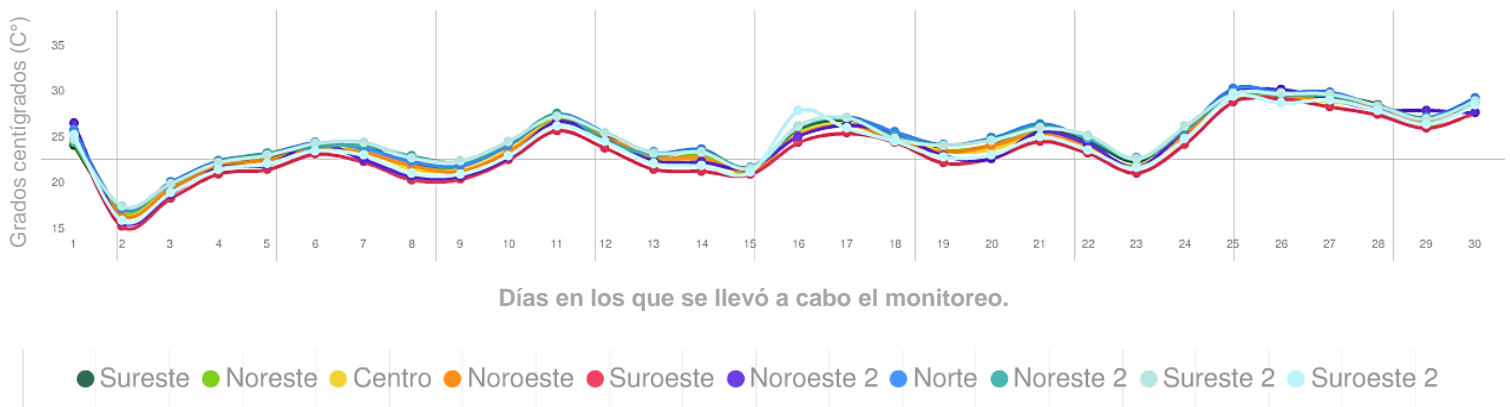
Figura 2: Temperatura promedio diaria por zona en el Área Metropolitana de Monterrey, Abril 2016.
