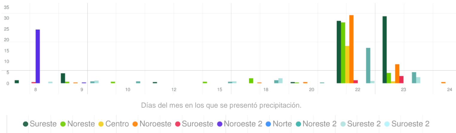
Figura 7: Precipitación pluvial acumulada por zona en el Área Metropolitana de Monterrey en el mes de Abril de 2016.
