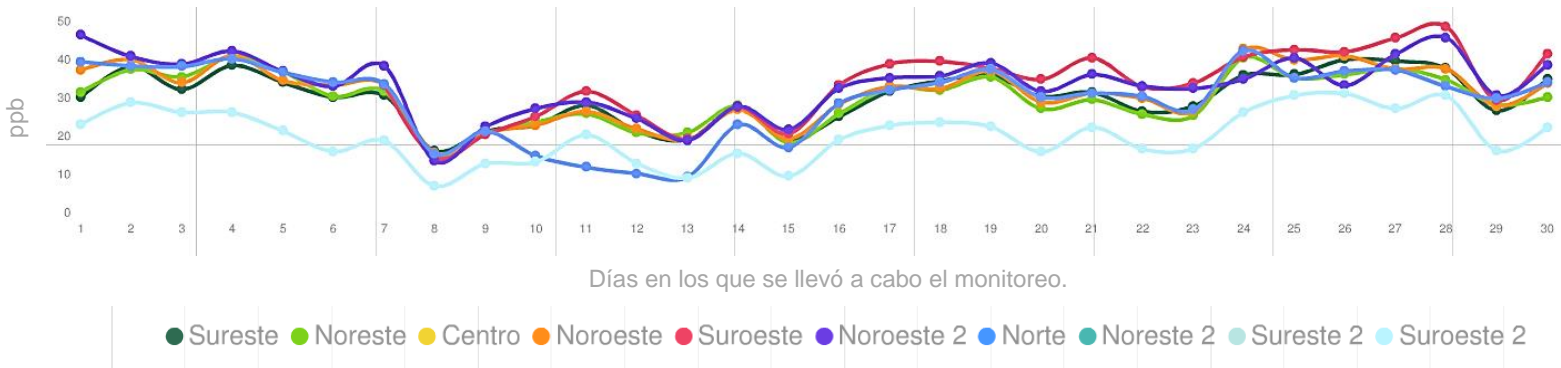
Figura 19: Concentración promedio diaria de ozono (O 3 ) por zona en el Área Metropolitana de Nuevo León.
