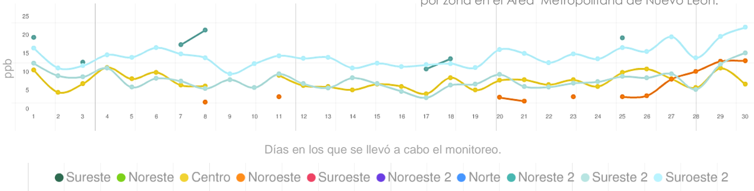
Figura 17: Concentración promedio diaria de bióxido de nitrógeno (NO 2 ) por zona en el Área Metropolitana de Nuevo León.
