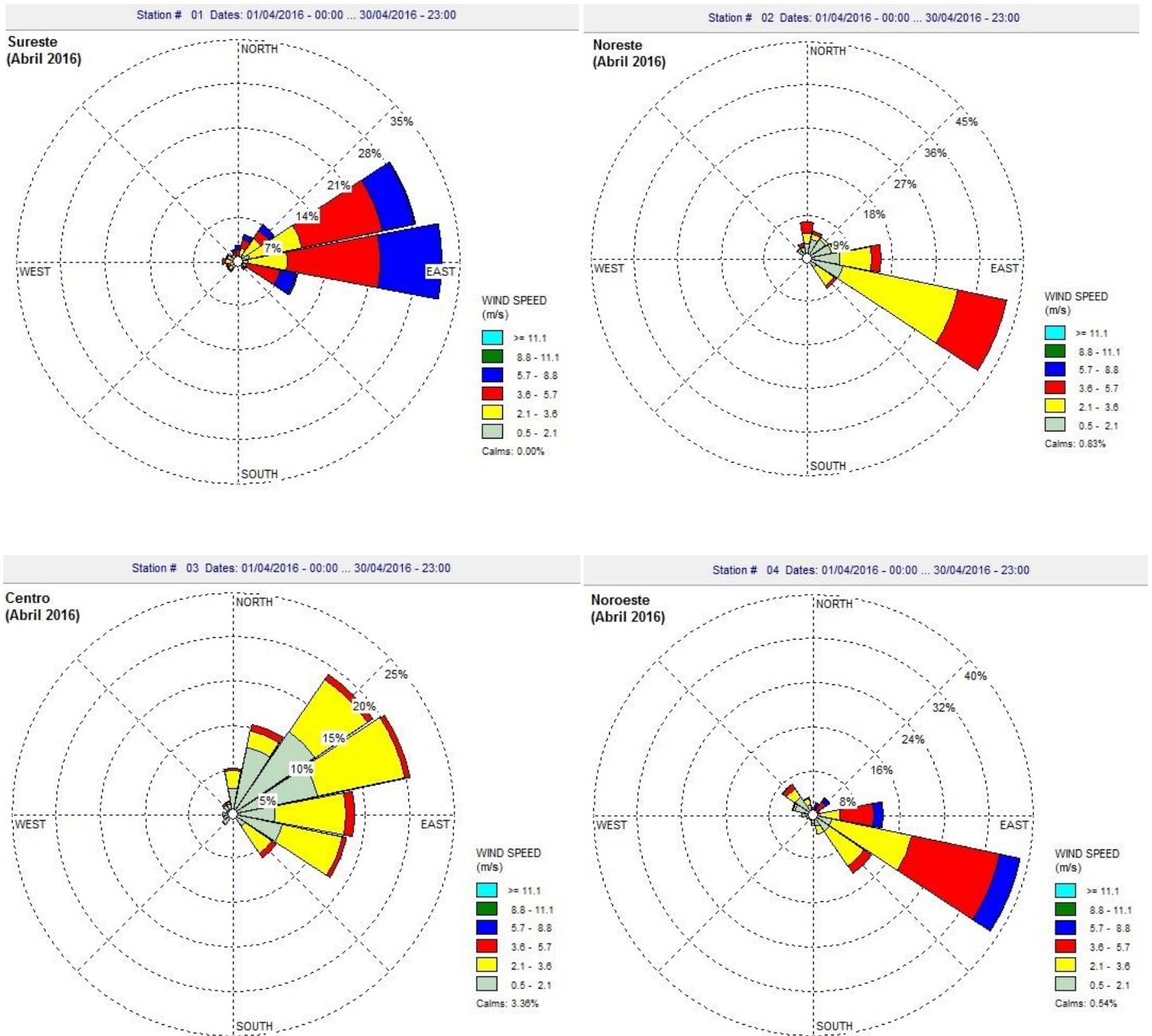
Figura 11: Velocidad del viento por zona en el Área Metropolitana de Nuevo León.
