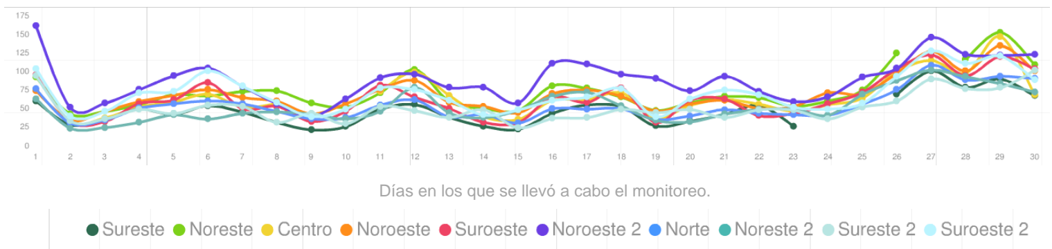
Figura 21: Concentración promedio diaria de ozono (PM 10 ) por zona en el Área Metropolitana de Nuevo León.
