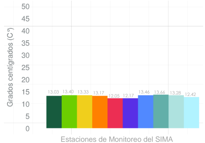
Figura 4: Temperatura mínima alcanzada por zona en el Área Metropolitana de Monterrey en el mes de Abril 2016
