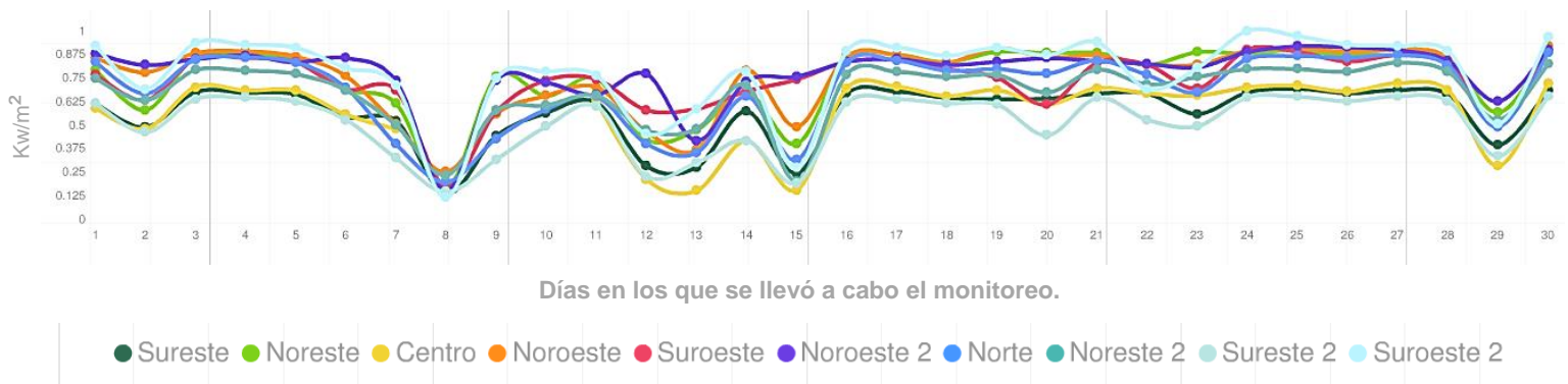
Figura 9: Radiación solar máxima diaria por zona en el Área Metropolitana de Monterrey en el mes de Abril de 2016.
