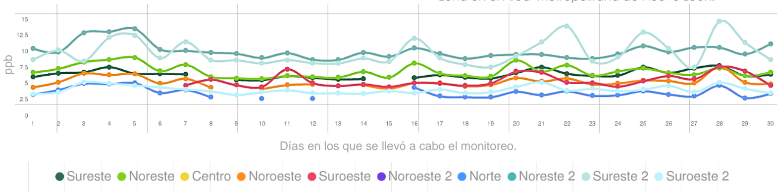
Figura 15: Concentración promedio diaria de bióxido de azufre (SO 2 ) por zona en el Área Metropolitana de Nuevo León.
