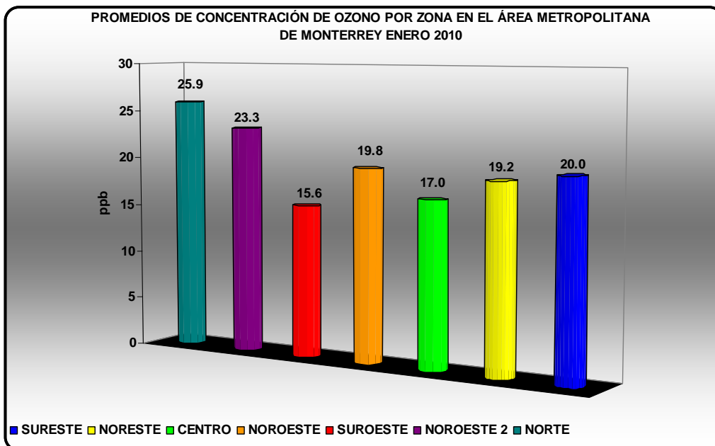
Figura 18: Promedio de concentración de Ozono por zona en el AMM
