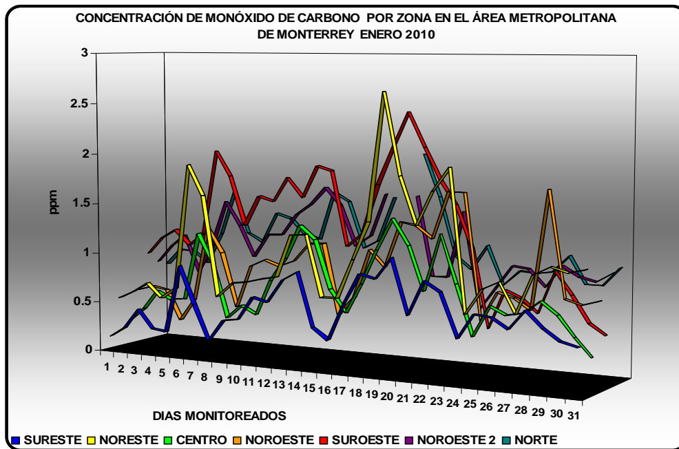
Figura 11: Concentración de Monóxido de Carbono por Zona en el AMM
