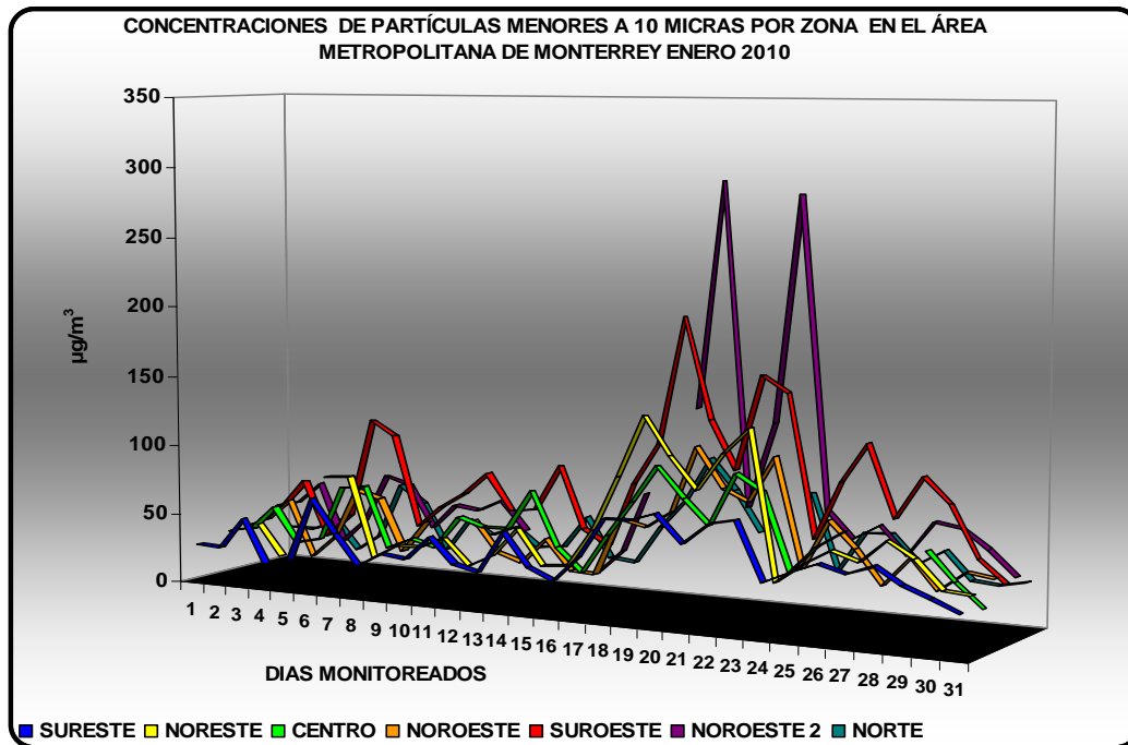
Figura 19: Promedio de concentración diaria de PM 10 por zona en el AMM
