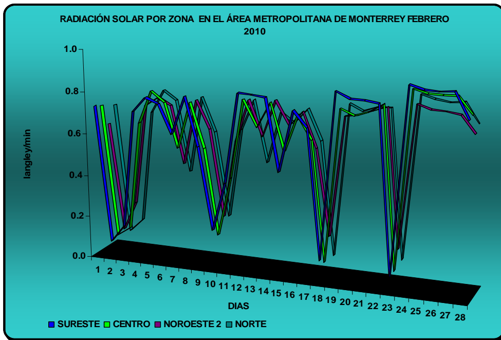
Figura 8: Radiación solar por zona en el AMM
