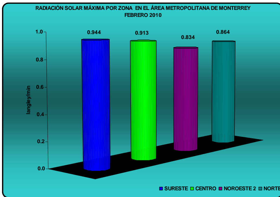
Figura 9: Radiación solar máxima por zona en el AMM
