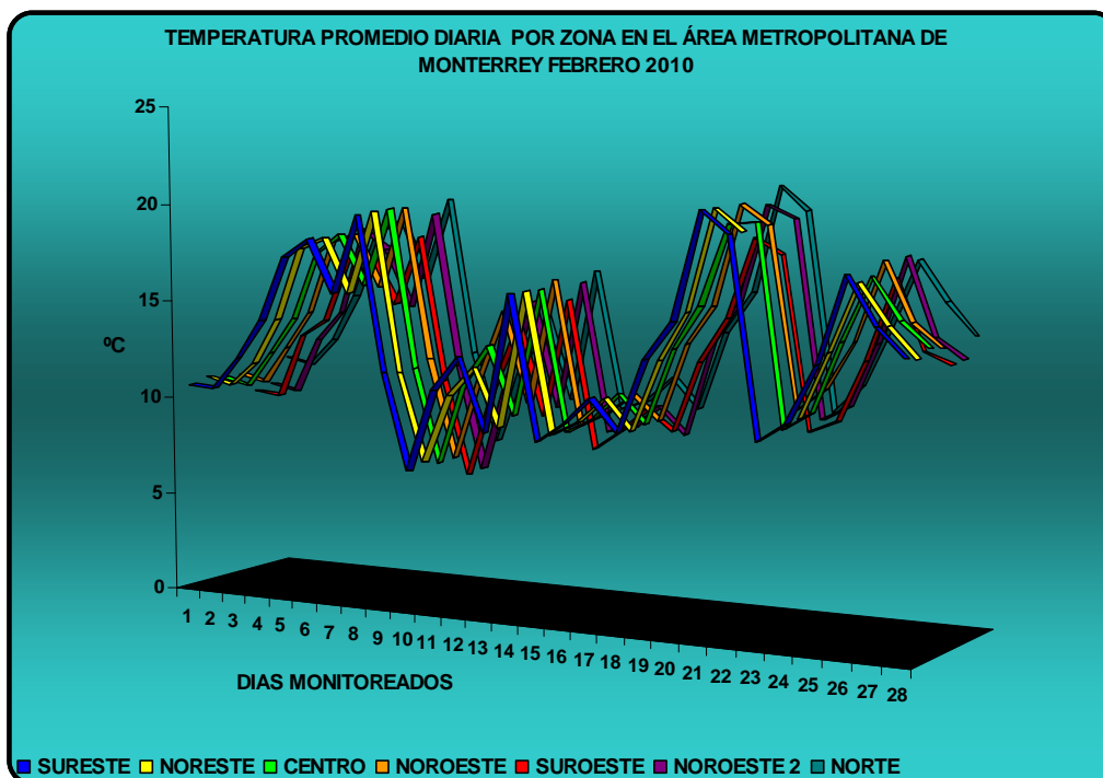
Figura 1: Temperatura Promedio Diaria por zona en el AMM
