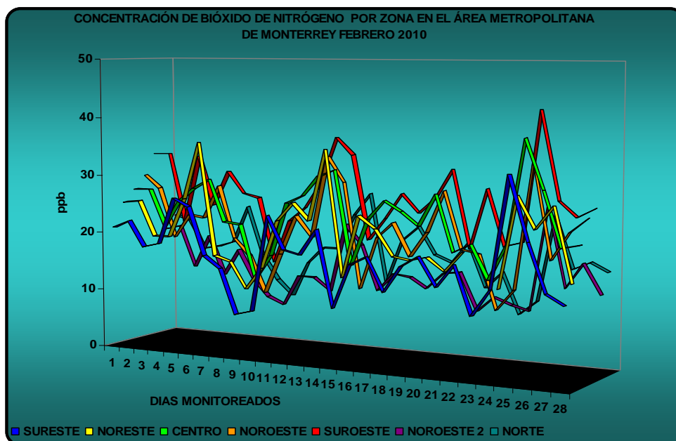
Figura 15: Concentración diaria de Bióxido de Nitrógeno por zona en el AMM
