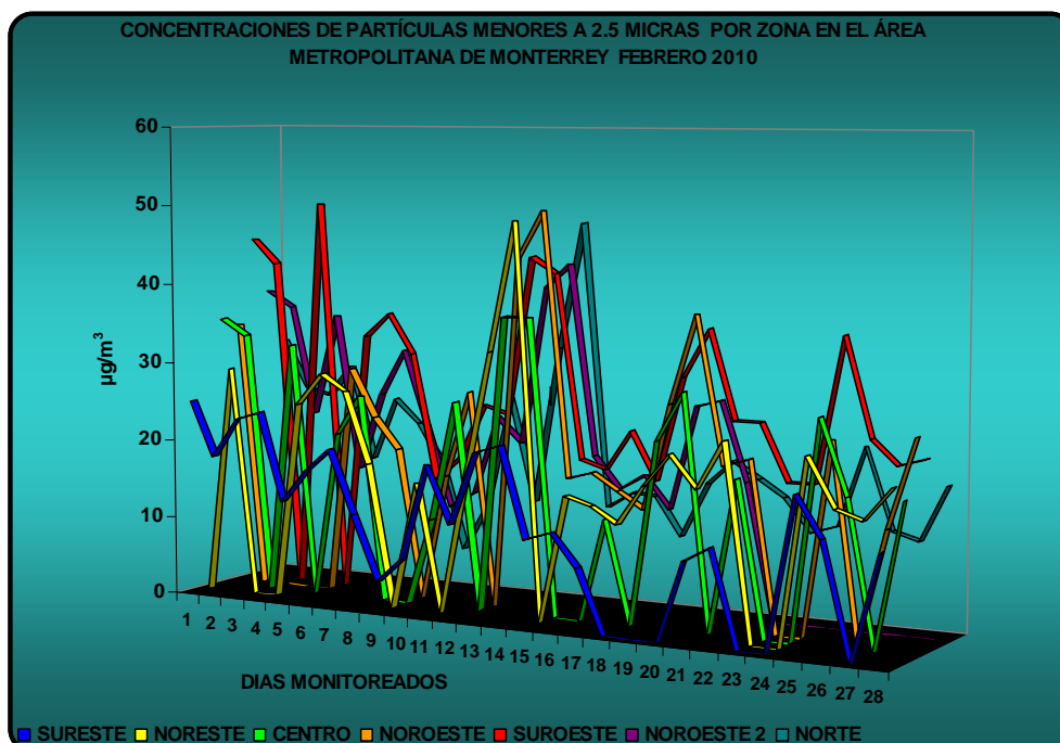
Figura 21: Promedio de concentración diaria de PM 2.5 por zona en el AMM
