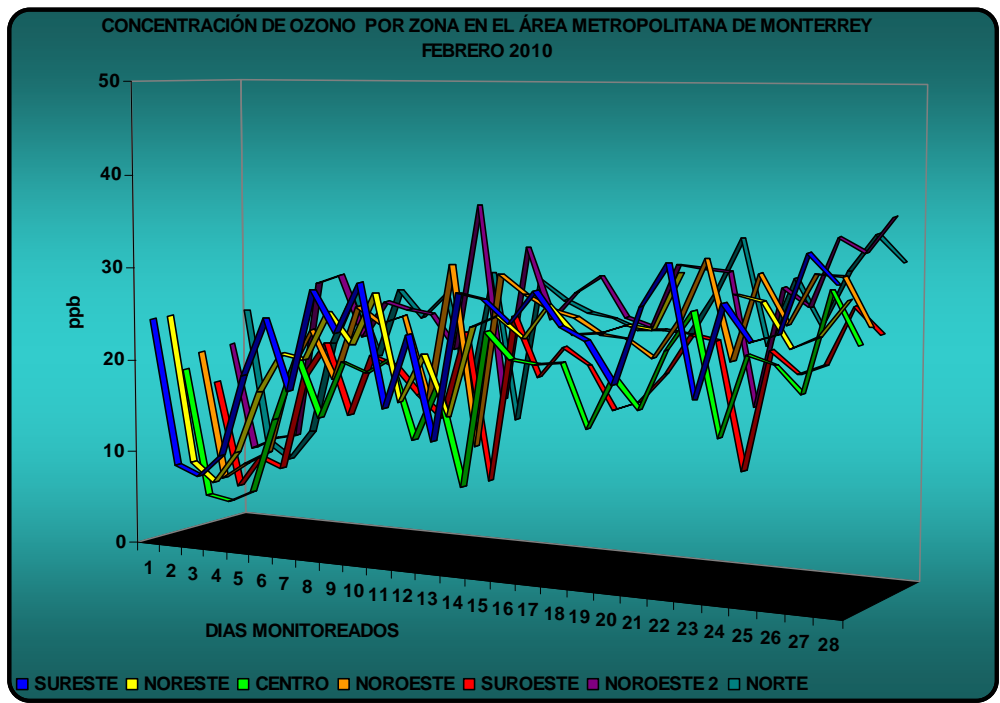
Figura 17: Promedio de concentración diaria de Ozono por zona en el AMM
