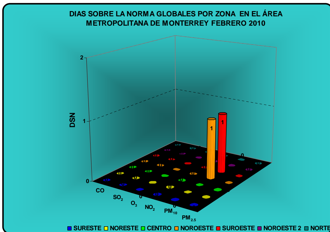
Figura 23: Días sobre la Norma globales por zona en el AMM
