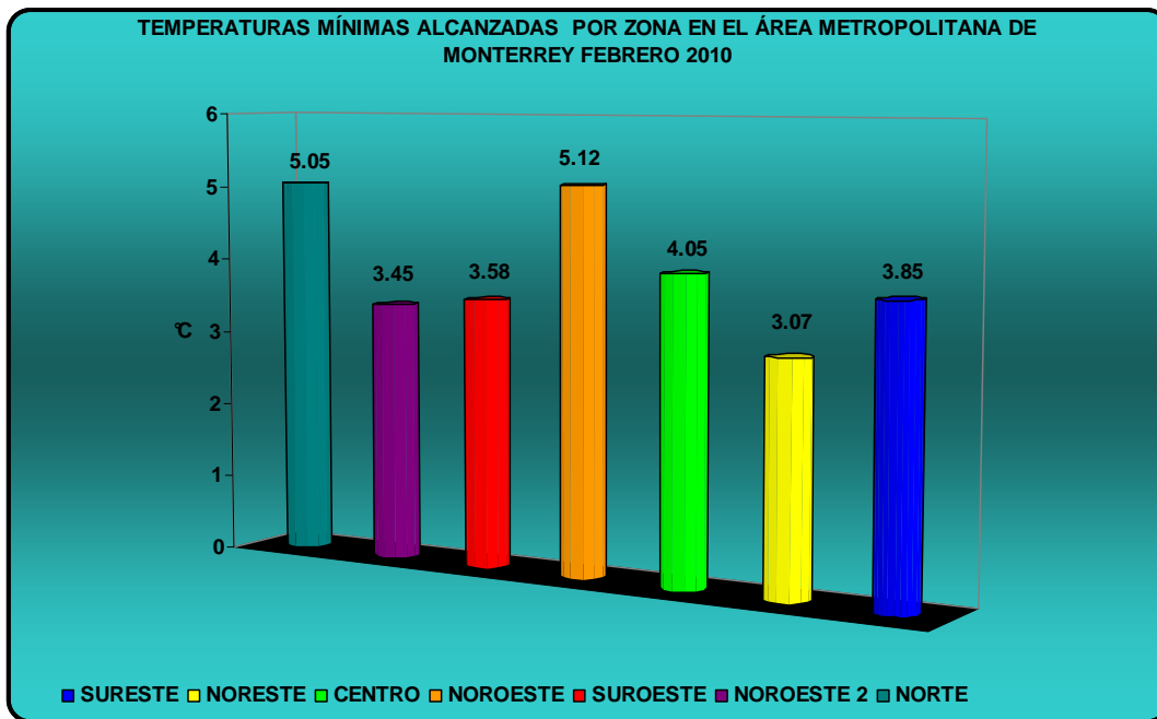
Figura 3: Temperatura Mínima por zona en el AMM
