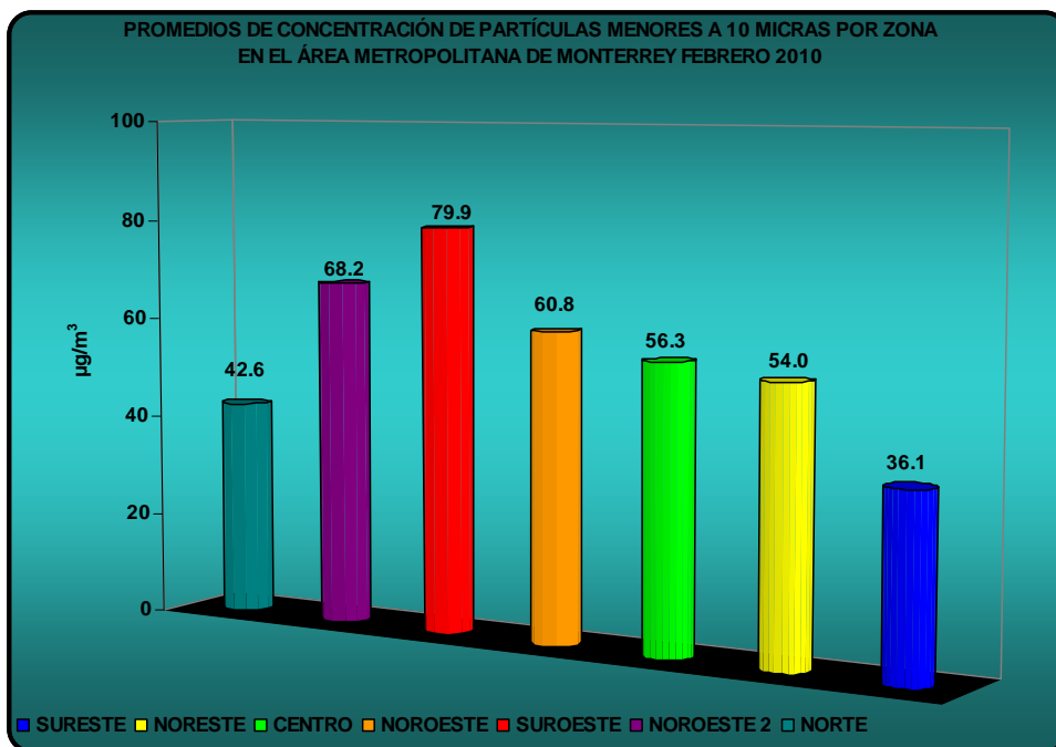
Figura 20: Promedio de concentración de partículas menores a 10 micras por zona en el AMM
