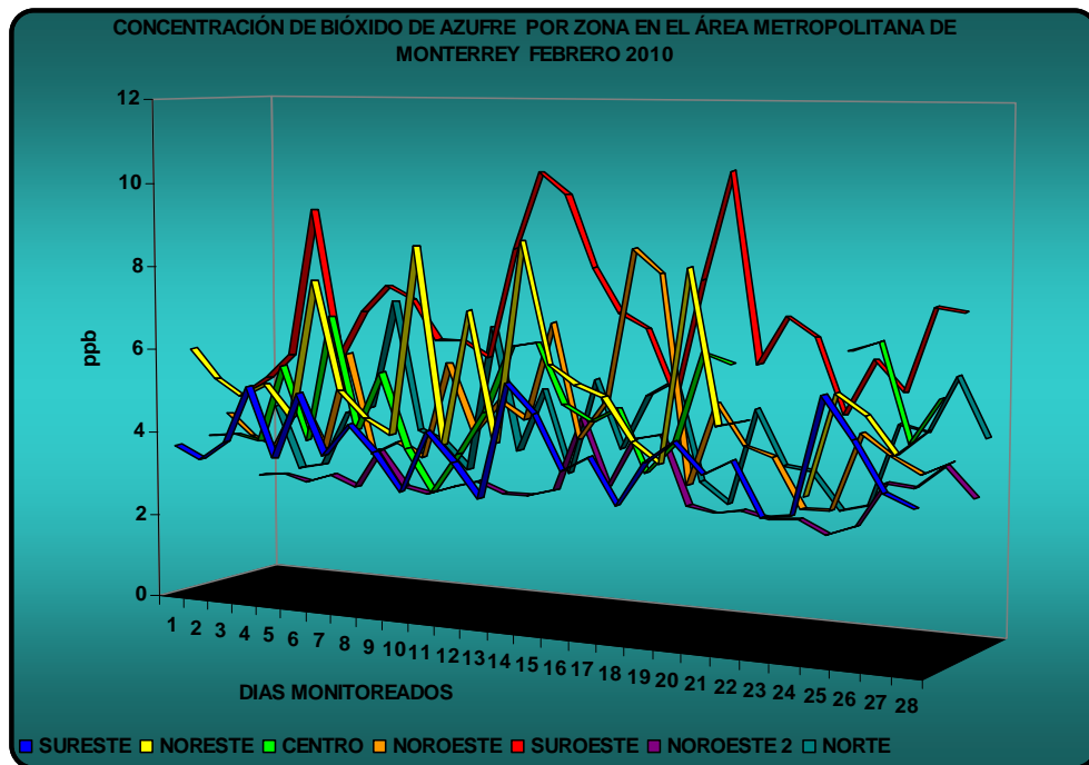
Figura 13: Concentración diaria de Bióxido de Azufre en el AMM
