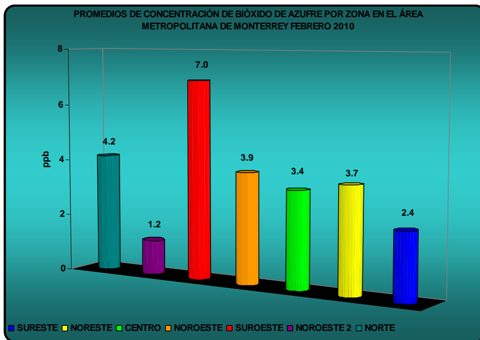
Figura 14: Promedio de concentración de Bióxido de Azufre por zona en el AMM
