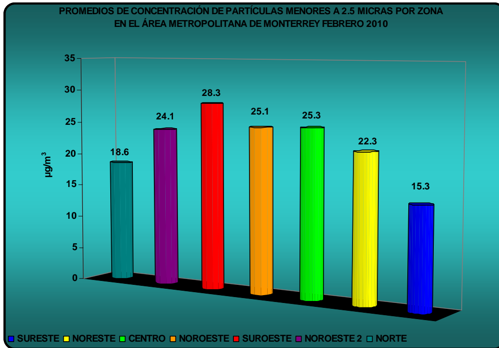
Figura 22: Promedio de concentración de partículas menores a 2.5 micras por zona en el AMM
