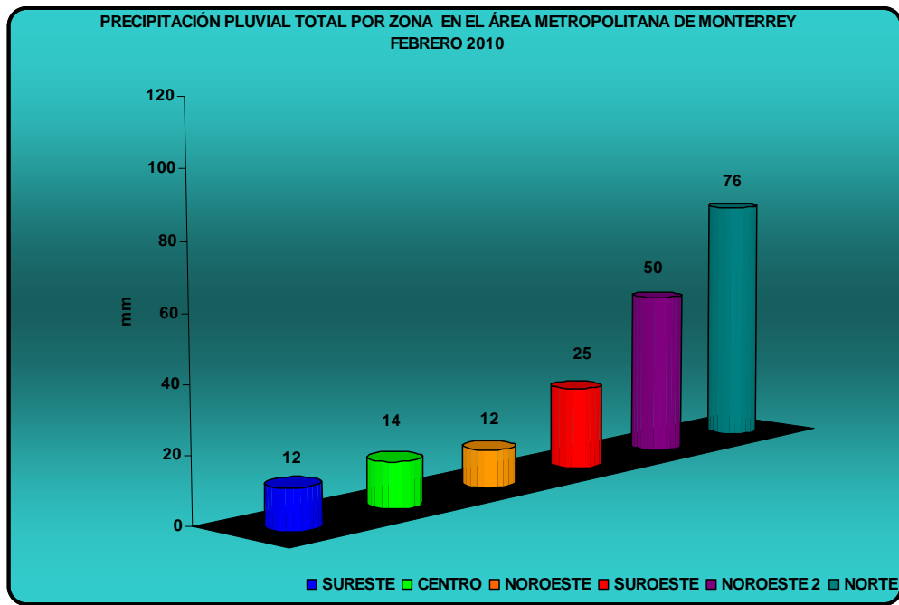
Figura 7: Precipitación pluvial total por zona en el AMM
