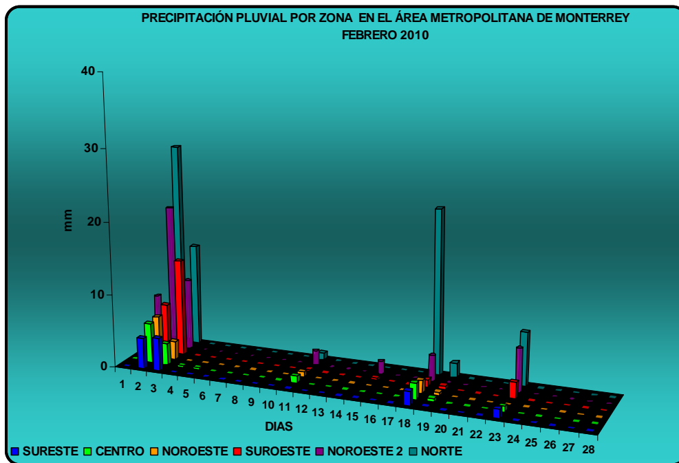
Figura 6: Precipitación pluvial por zona en el AMM
