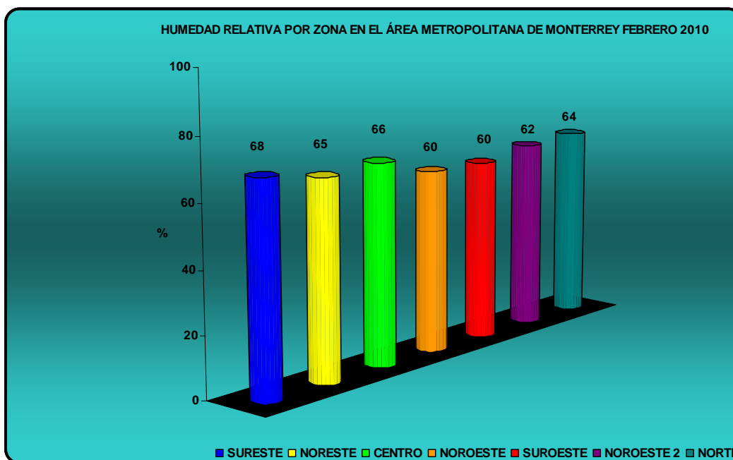
Figura 5: Humedad relativa promedio por zona en el AMM
