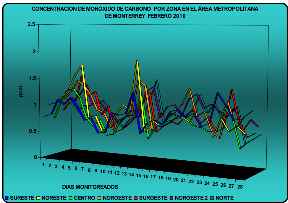
Figura 11: Concentración de Monóxido de Carbono por Zona en el AMM
