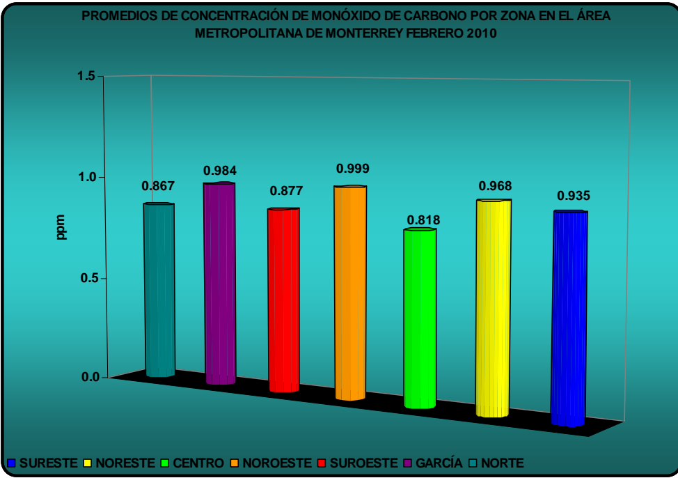
Figura 12: Promedios de concentración de Monóxido de Carbono por zona en el AMM
