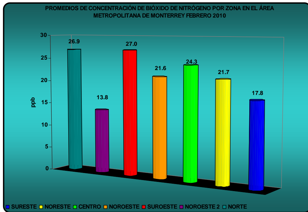
Figura 16: Promedio de concentración de Bióxido de Nitrógeno por zona en el AMM
