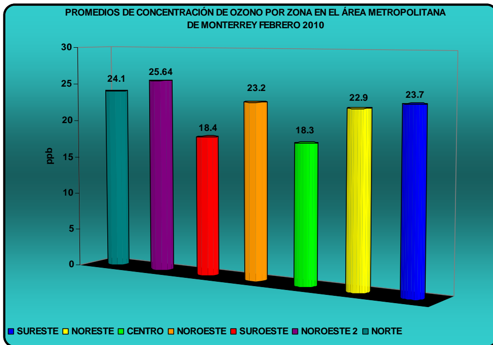
Figura 18: Promedio de concentración de Ozono por zona en el AMM
