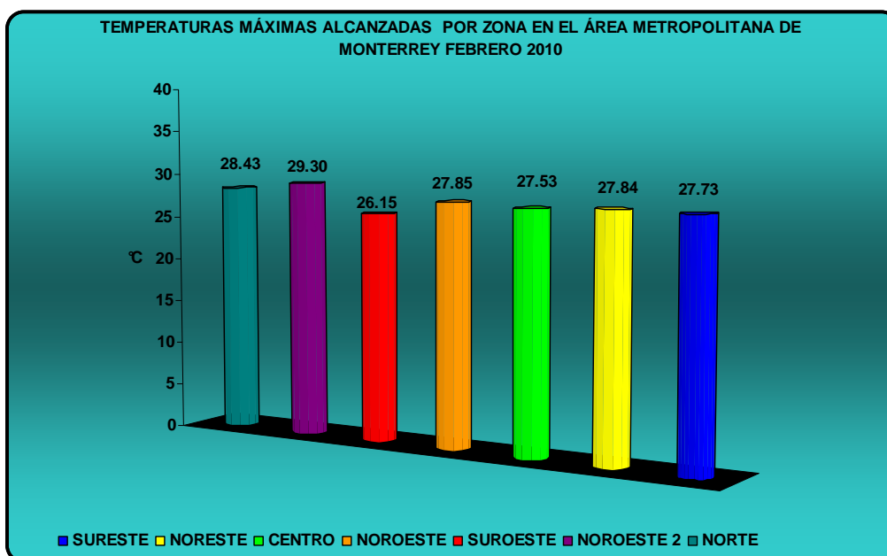
Figura 2: Temperatura Máxima por Zona en el AMM
