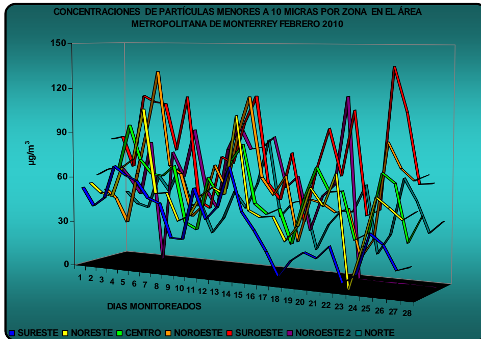
Figura 19: Promedio de concentración diaria de PM 10 por zona en el AMM
