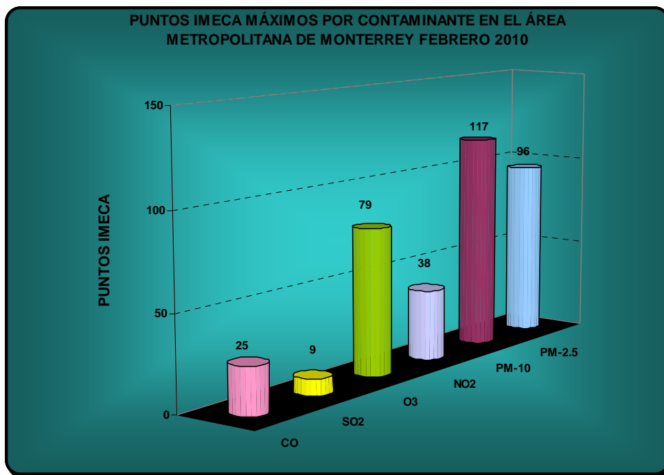
Figura 24: IMECA máximo por contaminante en el AMM
