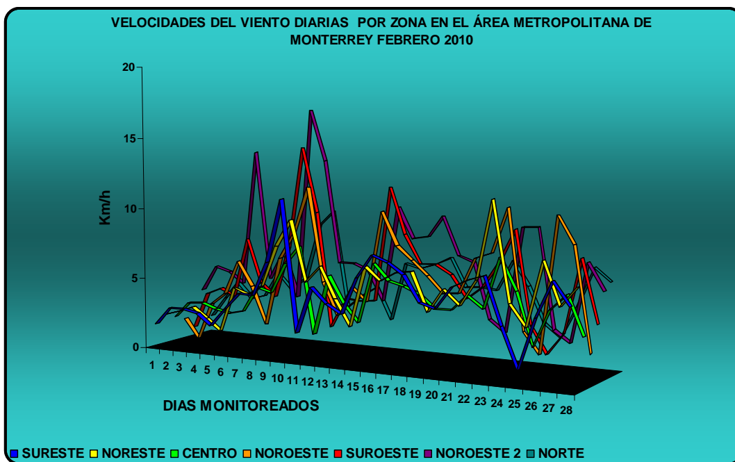
Figura 10: Velocidades del viento Diarias por Zona en el AMM
