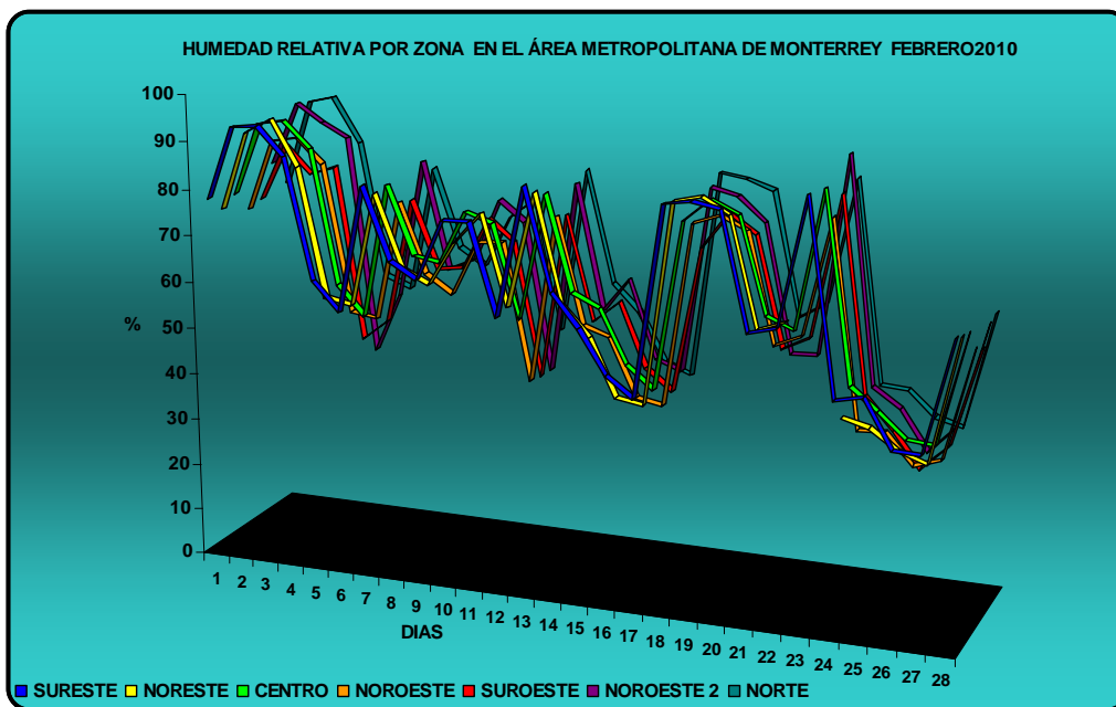
Figura 4: Humedad relativa por zona en el AMM
