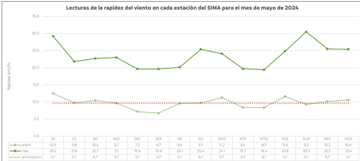
Figura 8. Rapidez del viento para cada estación del SIMA.
