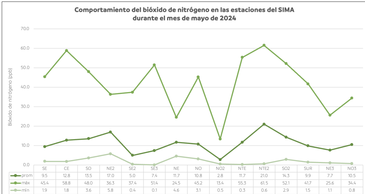
Figura 28. Comportamiento mensual del bióxido de nitrógeno en la ZMM
