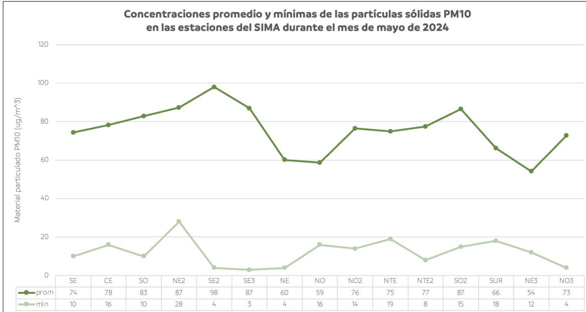
Figura 30. Comportamiento mensual promedio y mínimo de PM 10 en la ZMM.
