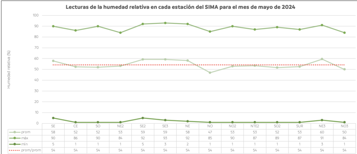
Figura 4. Comportamiento mensual de la humedad relativa en la ZMM.
