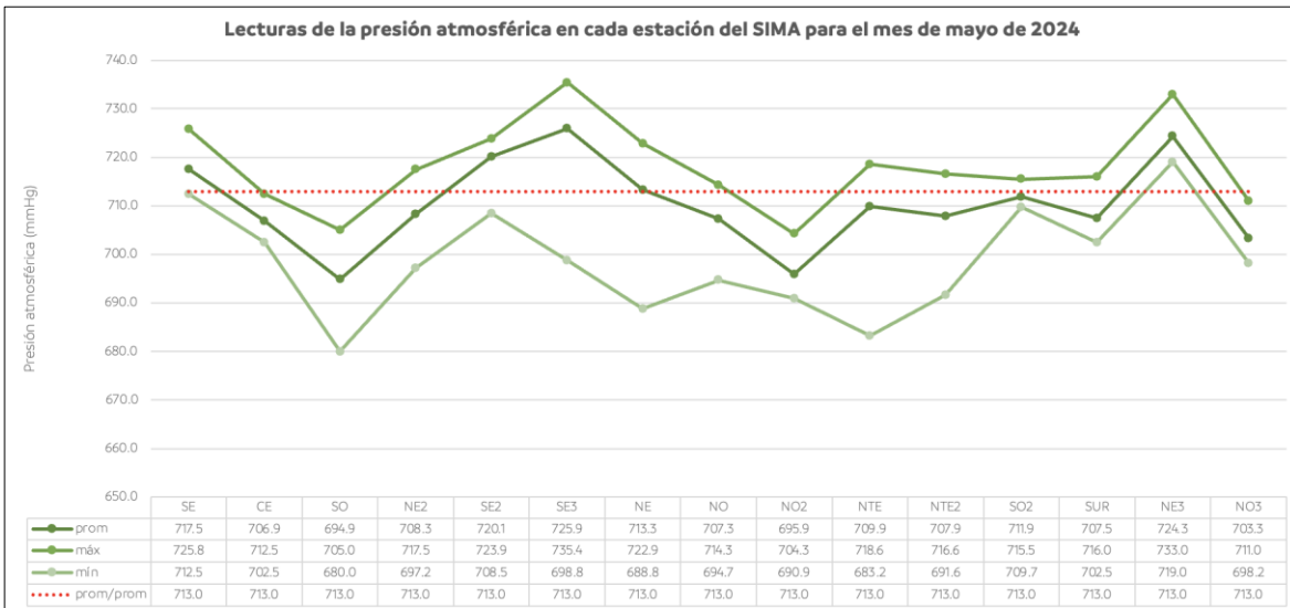
Figura 5. Comportamiento mensual de la presión atmosférica en la ZMM.
