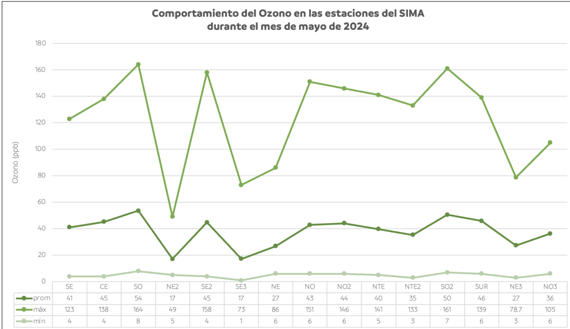
Figura 24. Comportamiento mensual del ozono en la ZMM.
