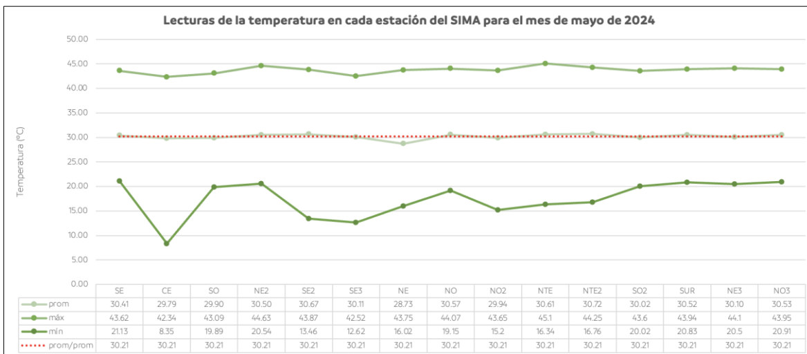
Figura 3. Comportamiento mensual de la temperatura en la ZMM.
