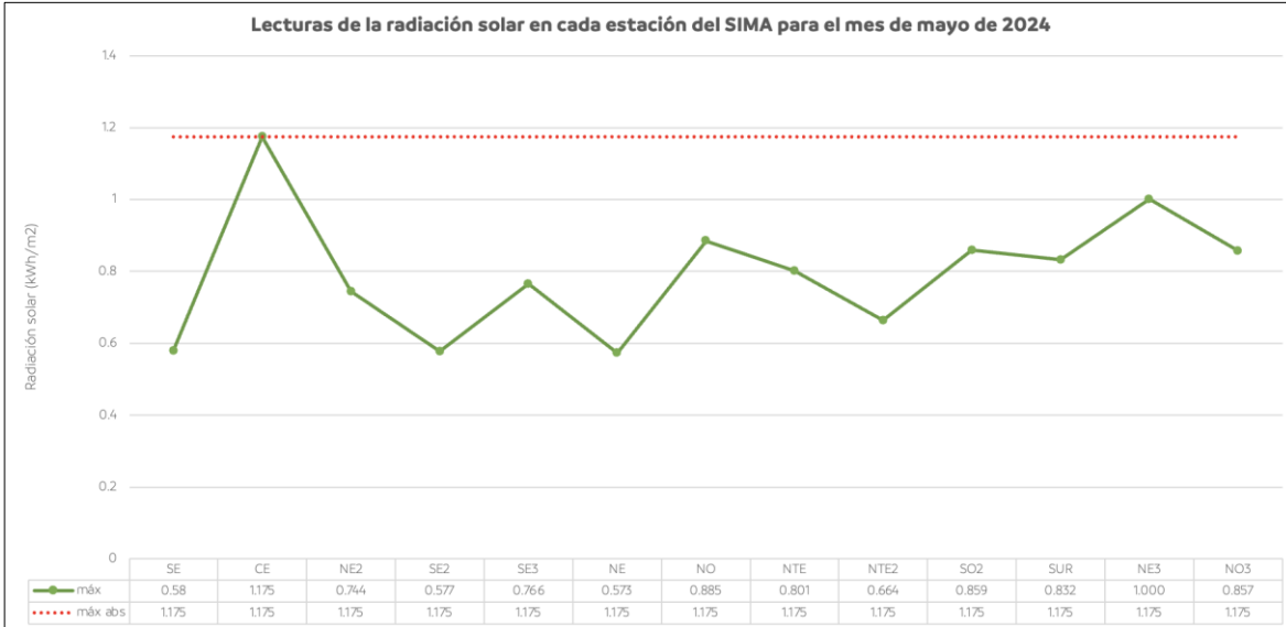
Figura 6. Comportamiento mensual de la radiación solar sobre la ZMM.
