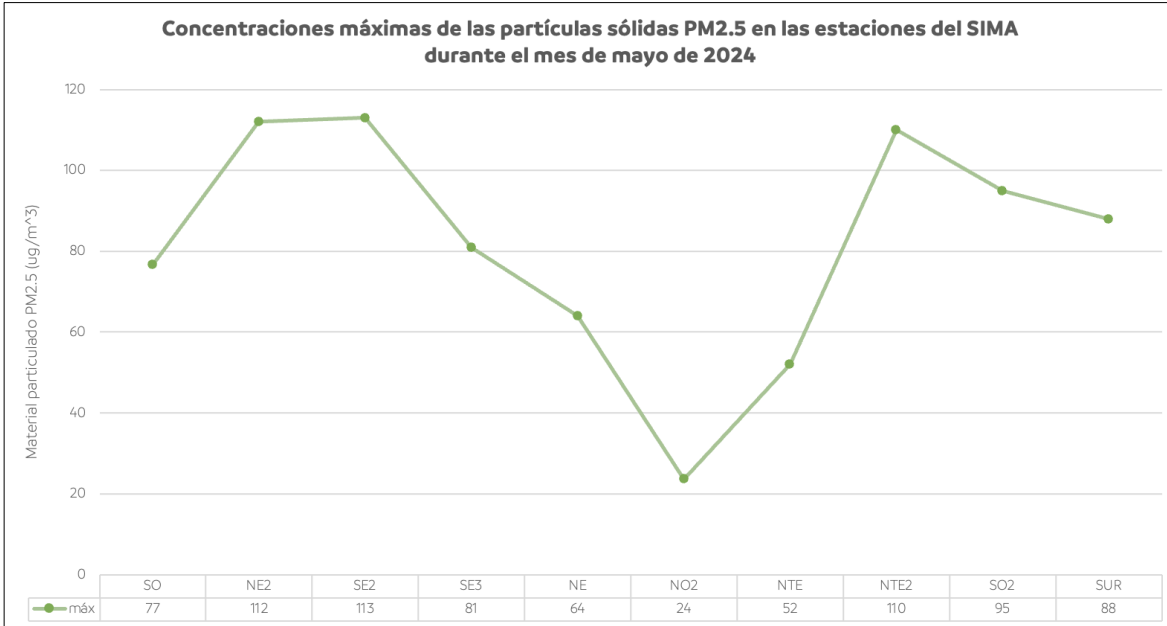
Figura 32. Comportamiento mensual máximo de PM 2.5 en la ZMM.
