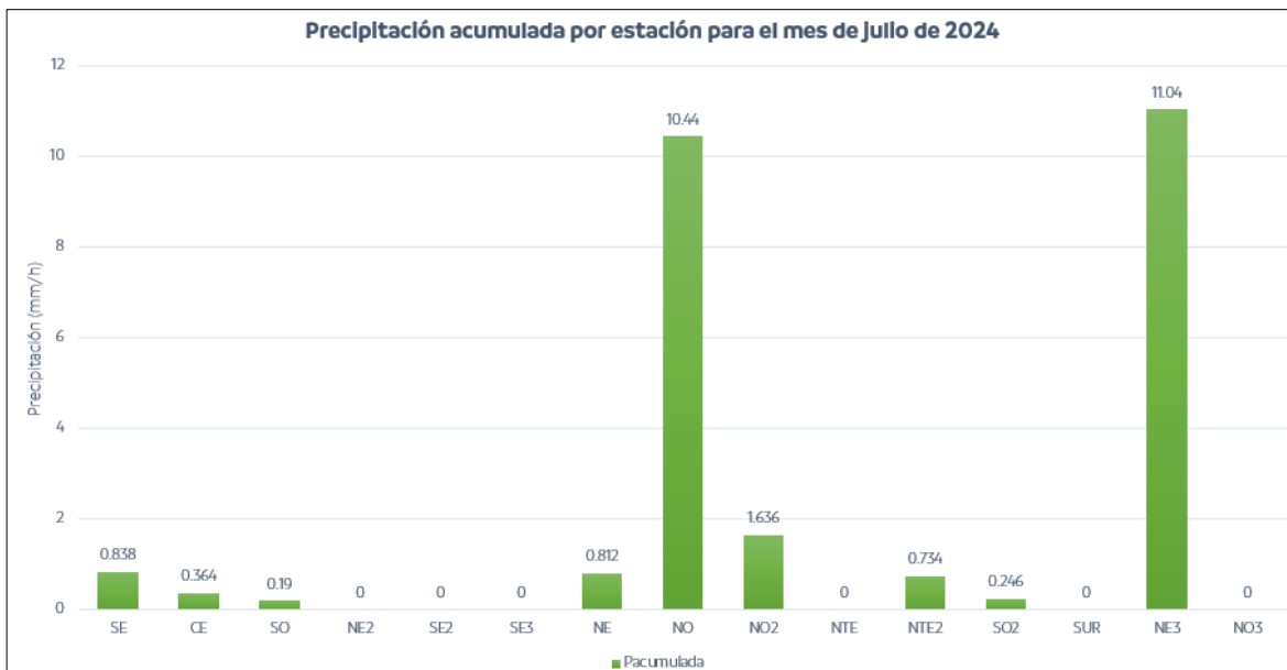
Figura 7. Acumulación de precipitación en estaciones del SIMA.
