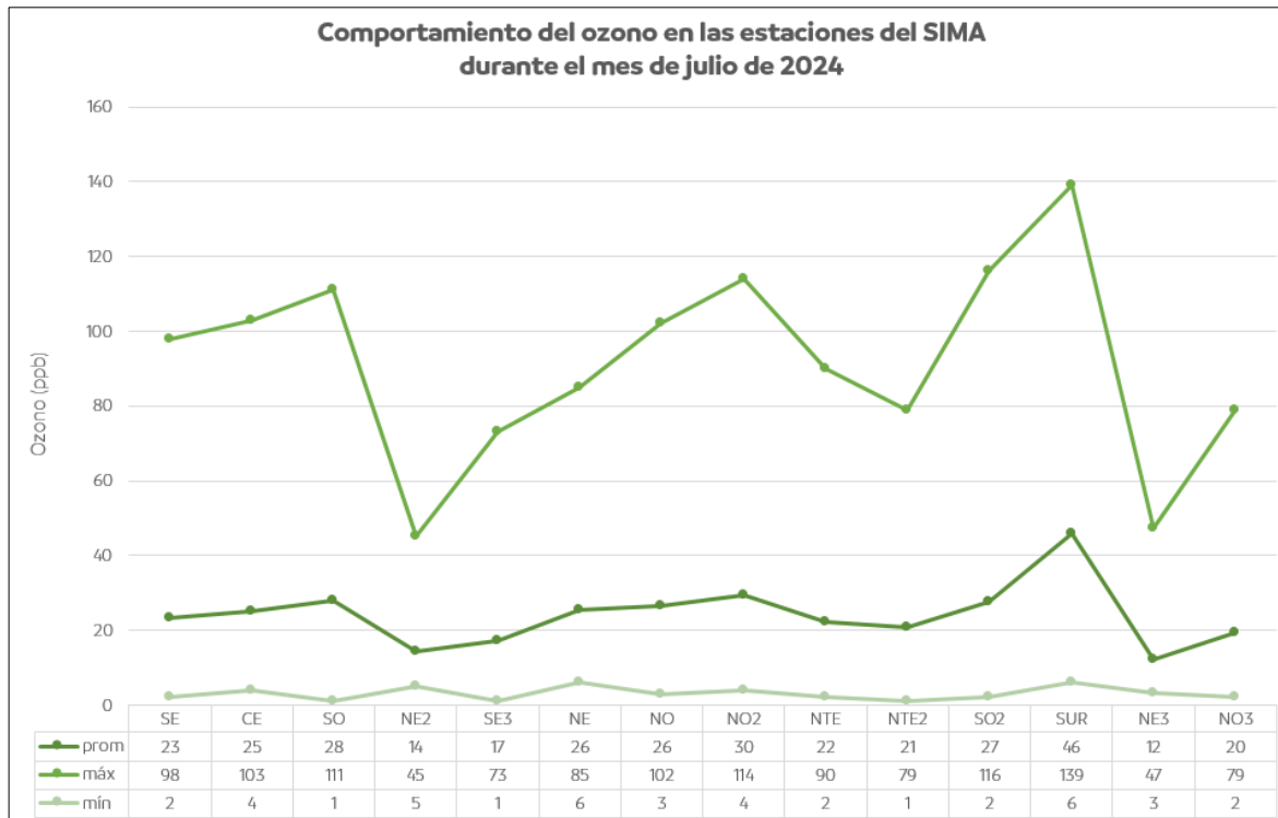
Figura 24. Comportamiento mensual del ozono en la ZMM.
