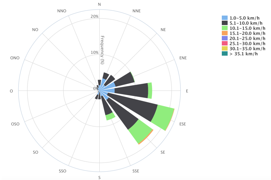
Figura 17. Distribución de la velocidad en la estación SE2.
