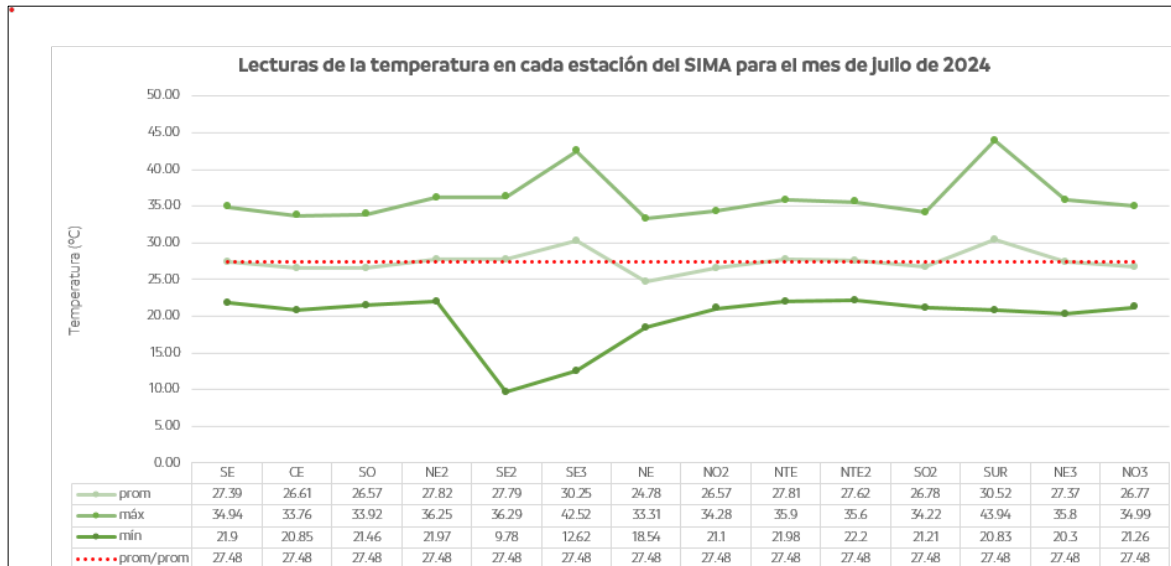
Figura 3. Comportamiento mensual de la temperatura en la ZMM.
