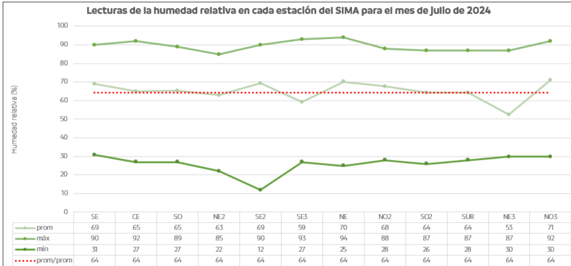
Figura 4. Comportamiento mensual de la humedad relativa en la ZMM.
