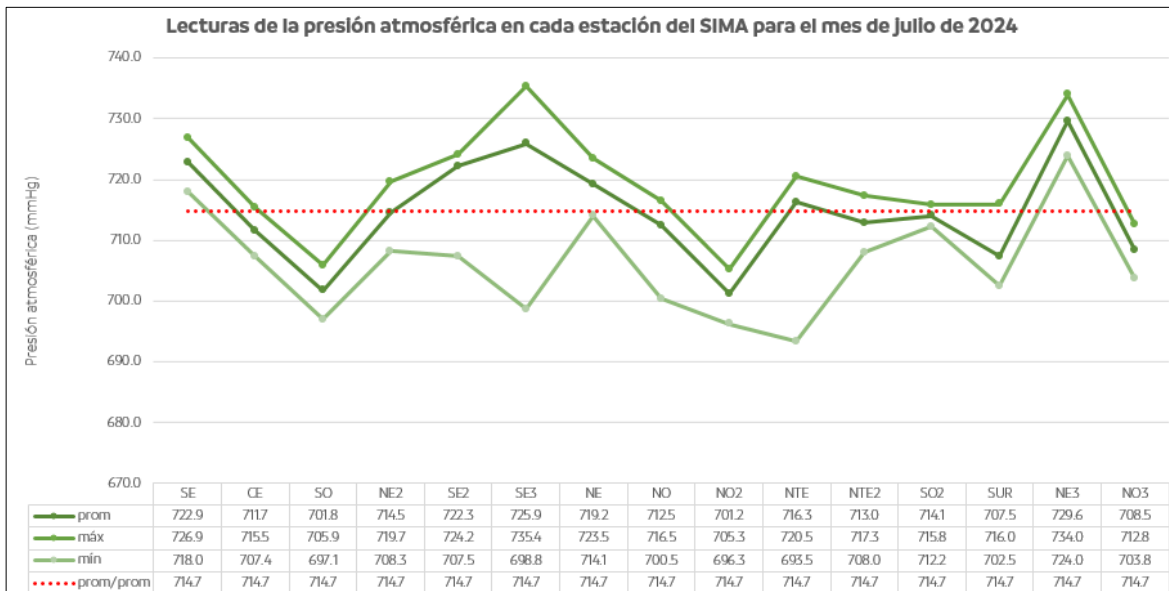
Figura 5. Comportamiento mensual de la presión atmosférica en la ZMM.
