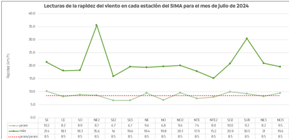
Figura 8. Rapidez del viento para cada estación del SIMA.
