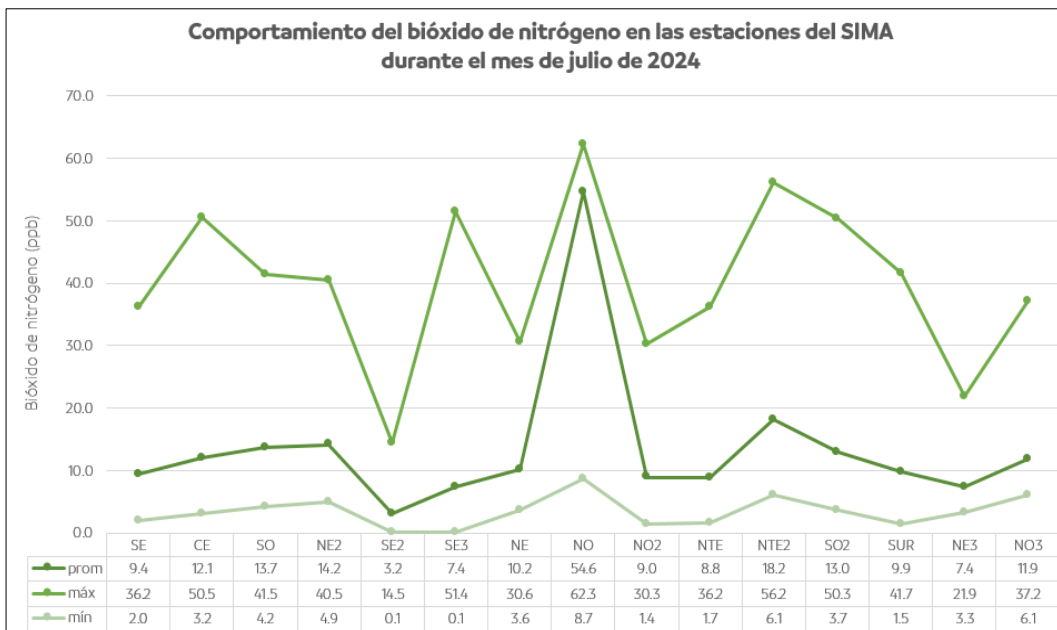
Figura 28. Comportamiento mensual del bióxido de nitrógeno en la ZMM
