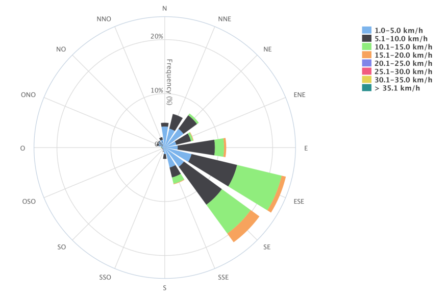
Figura 18. Distribución de la velocidad en la estación SE3.
