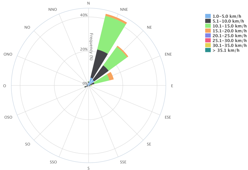
Figura 23. Distribución de la velocidad en la estación NO3.
