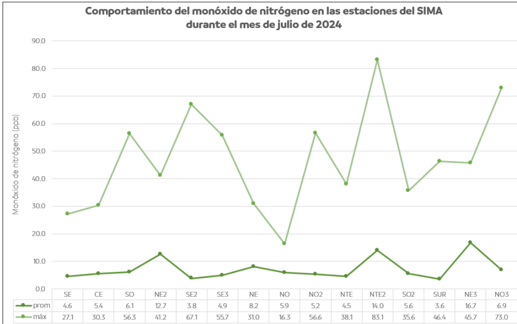
Figura 27. Comportamiento mensual del monóxido de nitrógeno en la ZMM.
