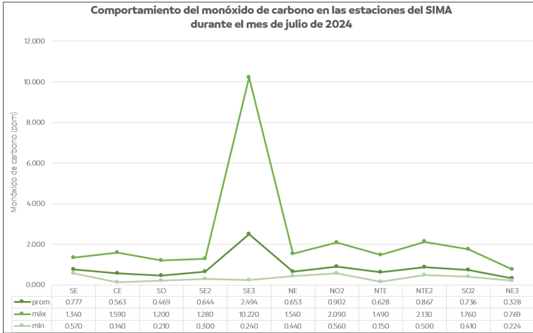
Figura 29. Comportamiento mensual del monóxido de carbono en la ZMM.
