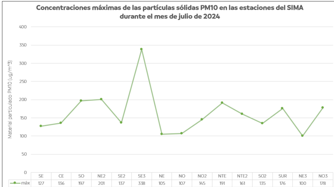
Figura 31. Comportamiento mensual máximo de PM 10 en la ZMM.
