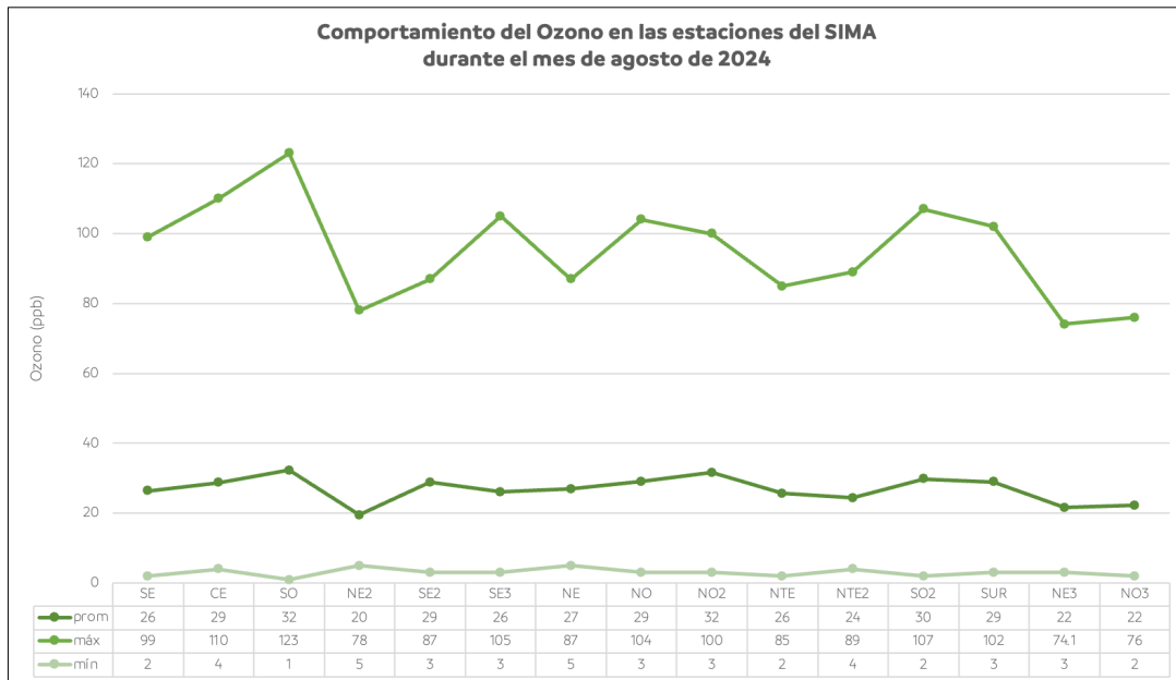
Figura 24. Comportamiento mensual del ozono en la ZMM.
