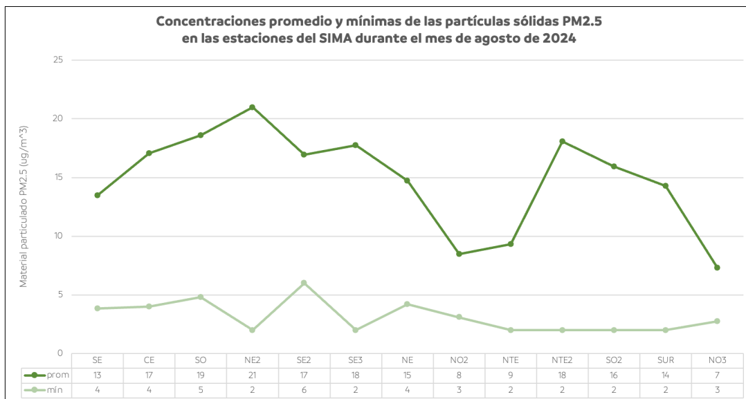
Figura 32. Comportamiento mensual máximo de PM 2.5 en la ZMM.
