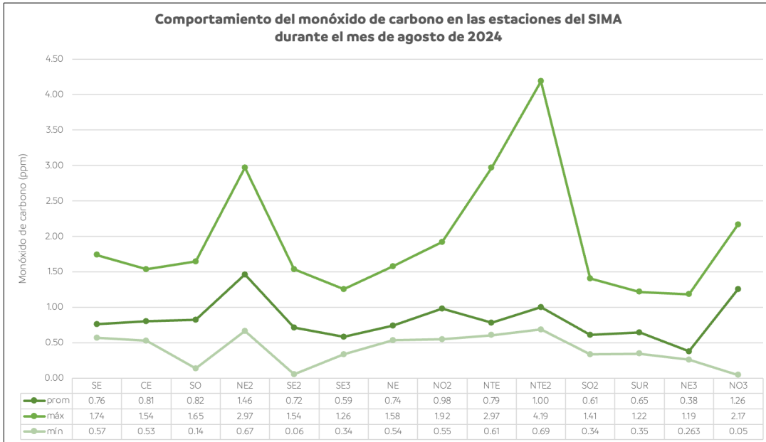
Figura 29. Comportamiento mensual del monóxido de carbono en la ZMM.
