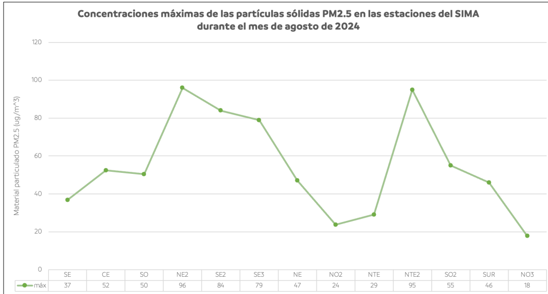
Figura 33. Comportamiento mensual promedio y mínimo de PM 2.5 en la ZMM.
