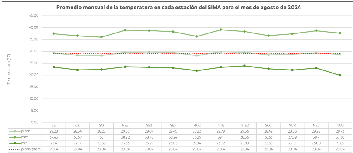
Figura 3. Comportamiento mensual de la temperatura en la ZMM.
