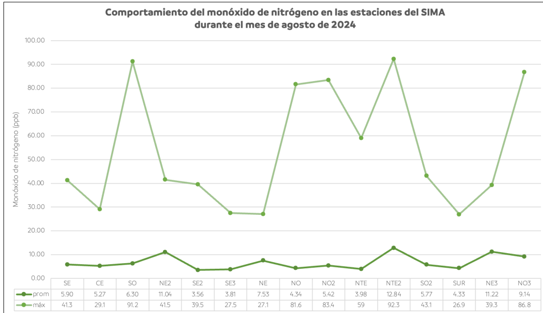
Figura 27. Comportamiento mensual del monóxido de nitrógeno en la ZMM.
