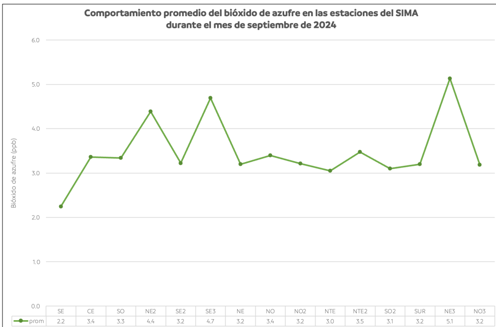
Figura 26. Comportamiento mensual promedio del bióxido de azufre en la ZMM.
