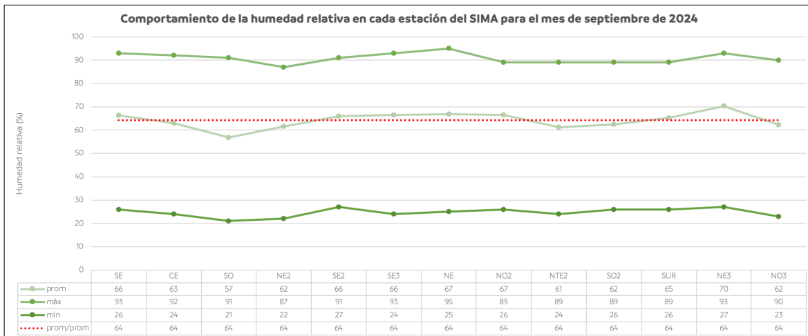
Figura 4. Comportamiento mensual de la humedad relativa en la ZMM.
