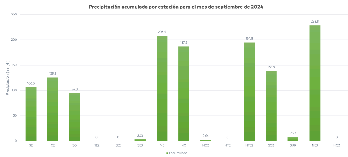
Figura 7. Acumulación de precipitación en estaciones del SIMA.
