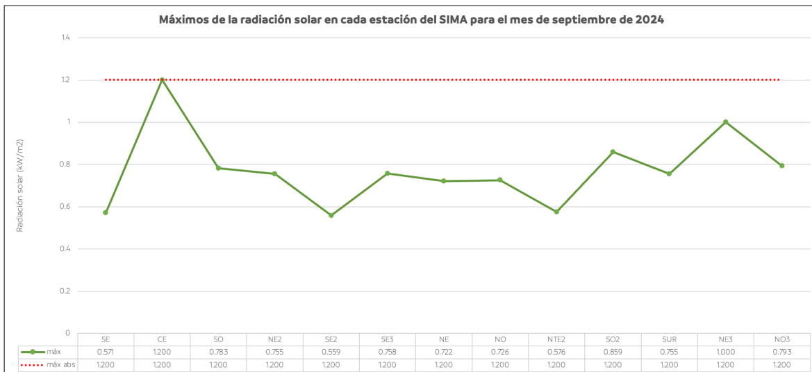
Figura 6. Comportamiento mensual de la radiación solar sobre la ZMM.
