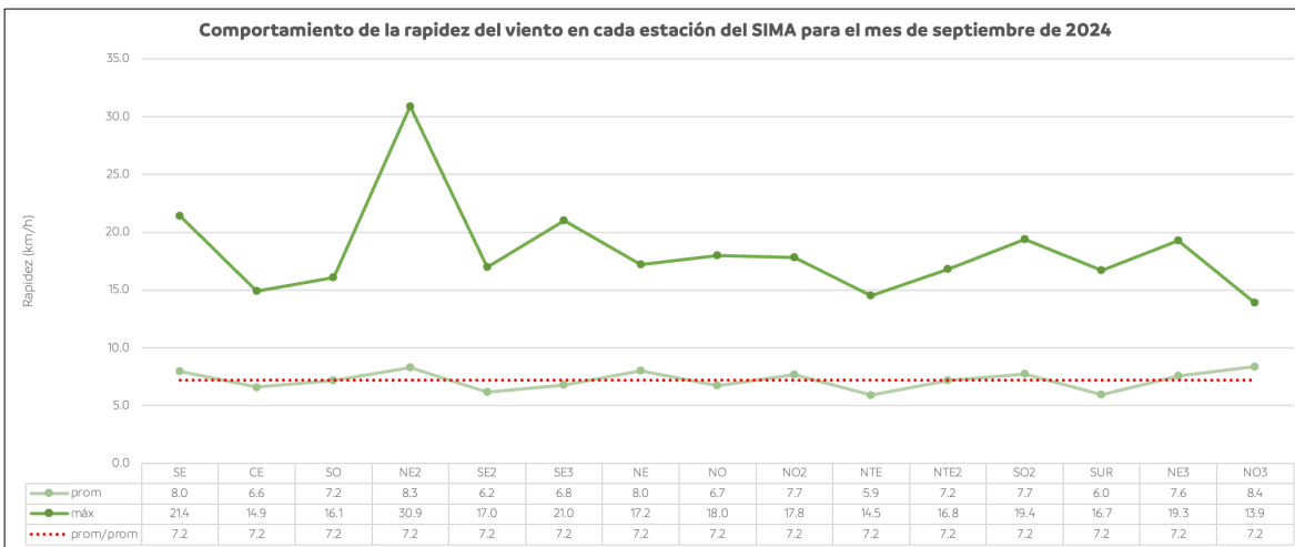
Figura 8. Rapidez del viento para cada estación del SIMA.
