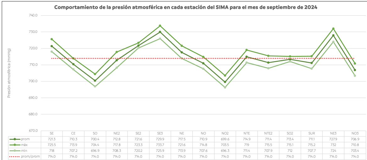
Figura 5. Comportamiento mensual de la presión atmosférica en la ZMM.
