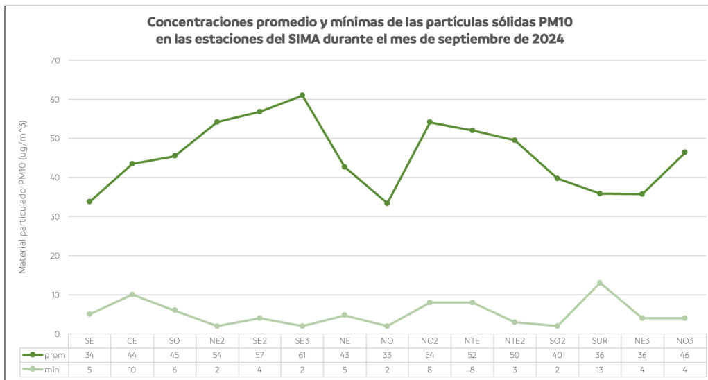
Figura 30. Comportamiento mensual promedio y mínimo de PM 10 en la ZMM.
