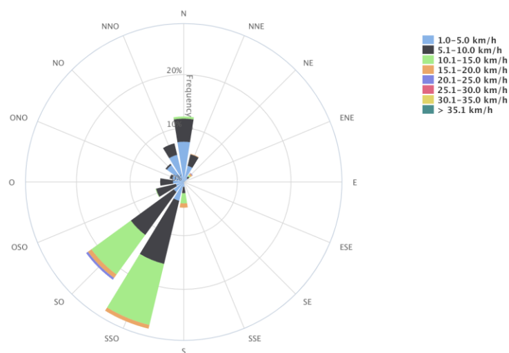
Figura 19. Distribución de la velocidad en la estación SO2.
