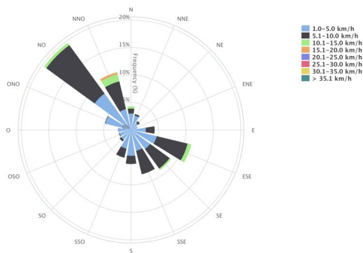
Figura 17. Distribución de la velocidad en la estación SE2.
