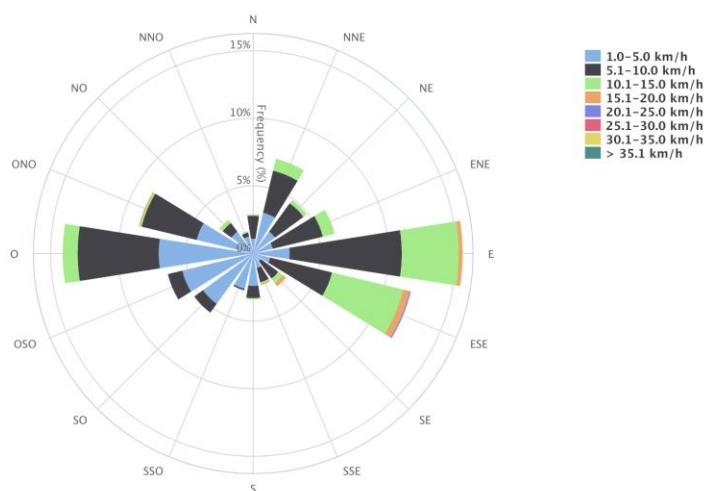
Figura 9. Distribución de la velocidad en la estación SE.
