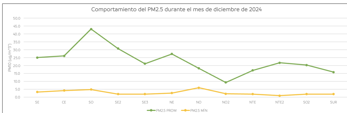
Figura 32. Comportamiento mensual promedio y mínimo de PM 2.5 en la ZMM.
