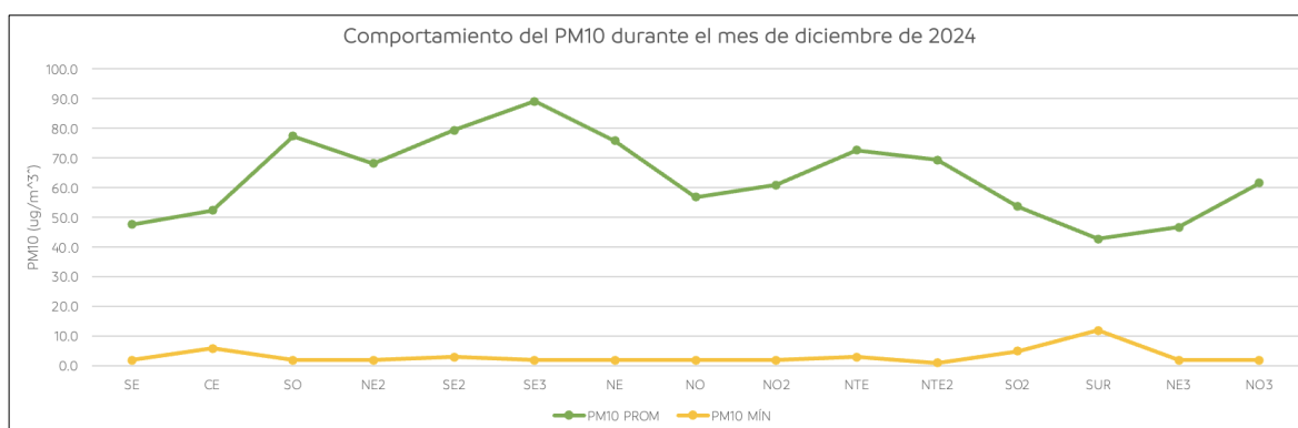
Figura 30. Comportamiento mensual promedio y mínimo de PM 10 en la ZMM.
