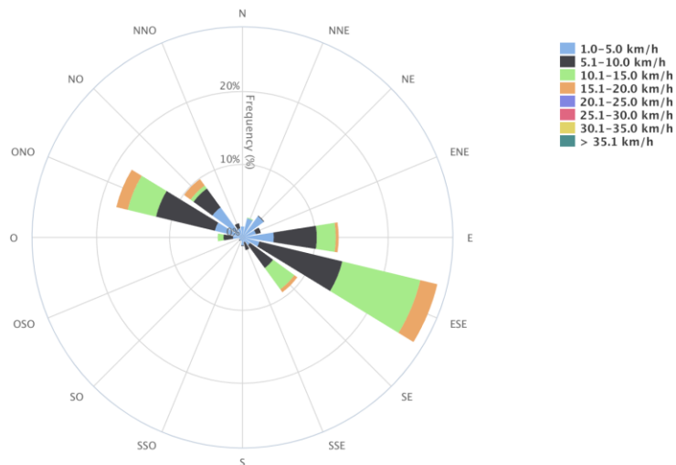
Figura 14. Distribución de la velocidad en la estación NO2.
