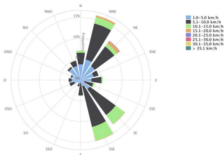
Figura 10. Distribución de la velocidad en la estación NE.
