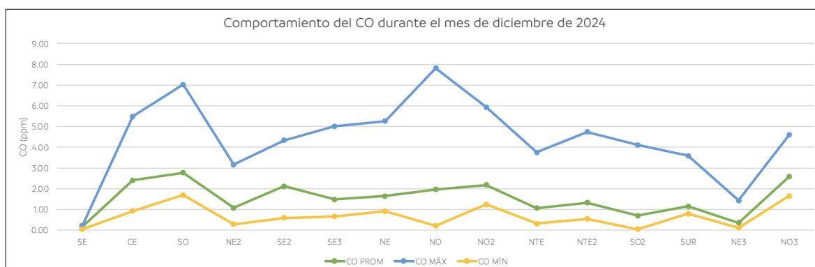
Figura 29. Comportamiento mensual del monóxido de carbono en la ZMM.
