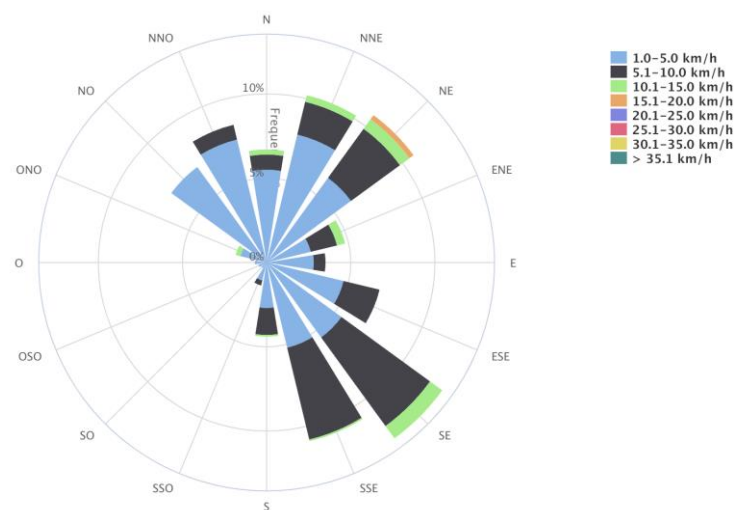
Figura 15. Distribución de la velocidad en la estación NTE.
