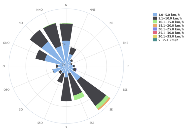
Figura 20. Distribución de la velocidad en la estación SUR.
