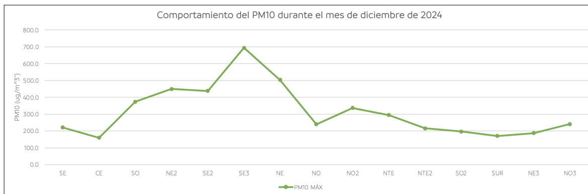
Figura 31. Comportamiento mensual máximo de PM 10 en la ZMM.
