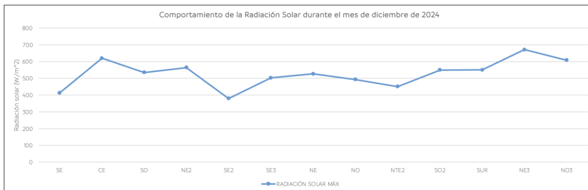
Figura 6. Comportamiento mensual de la radiación solar sobre la ZMM.
