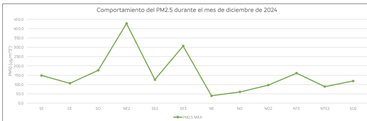
Figura 33. Comportamiento mensual máximo de PM 2.5 en la ZMM.
