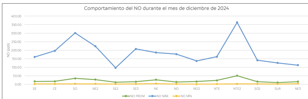
Figura 27. Comportamiento mensual del monóxido de nitrógeno en la ZMM.
