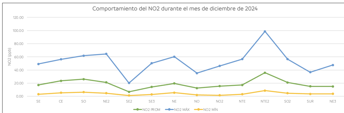
Figura 28. Comportamiento mensual del bióxido de nitrógeno en la ZMM
