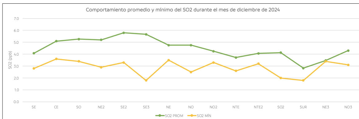
Figura 26. Comportamiento mensual promedio del bióxido de azufre en la ZMM.
