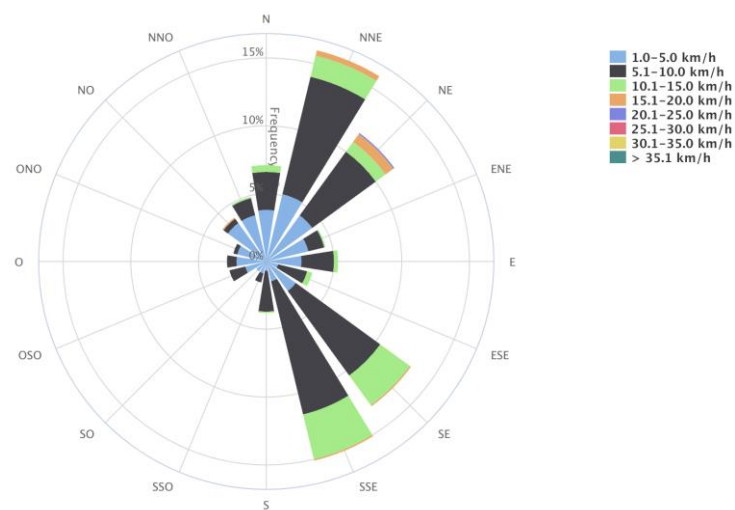
Figura 11. Distribución de la velocidad en la estación CE.
