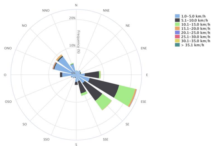
Figura 13. Distribución de la velocidad en la estación SO.
