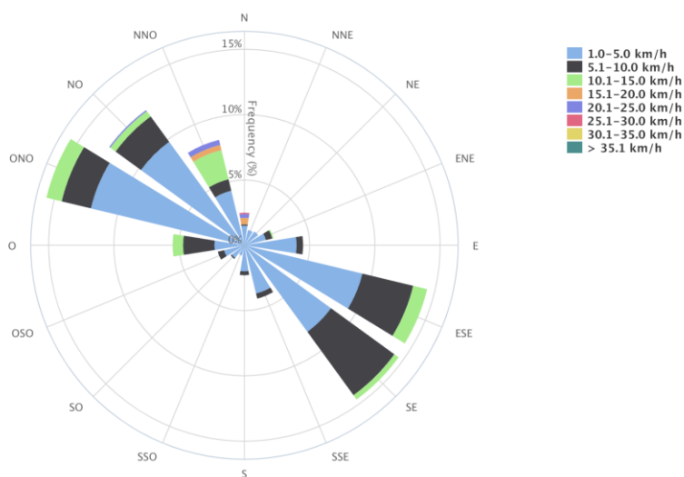
Figura 22. Distribución de la velocidad en la estación NE3.
