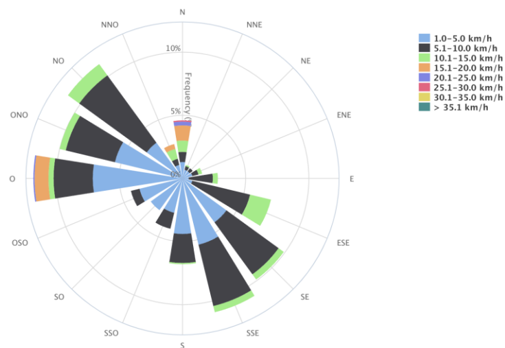
Figura 12. Distribución de la velocidad en la estación NO.
