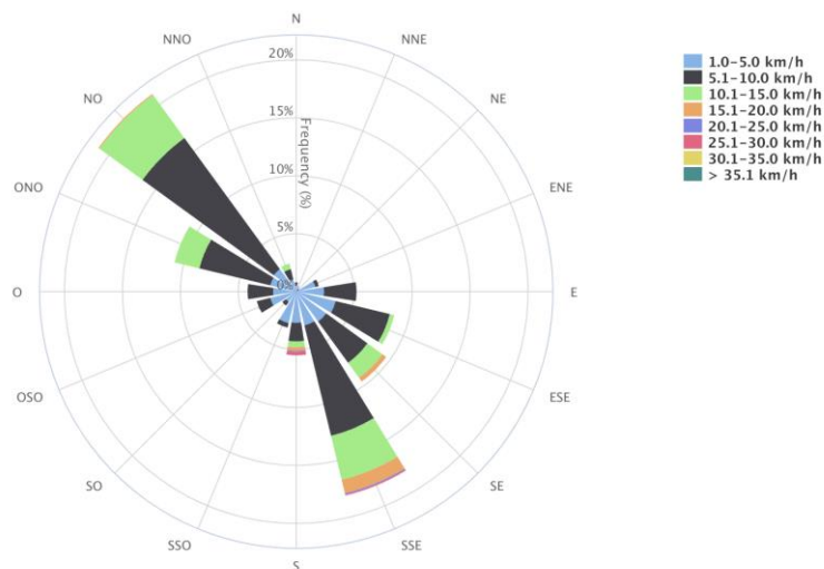
Figura 16. Distribución de la velocidad en la estación NE2.
