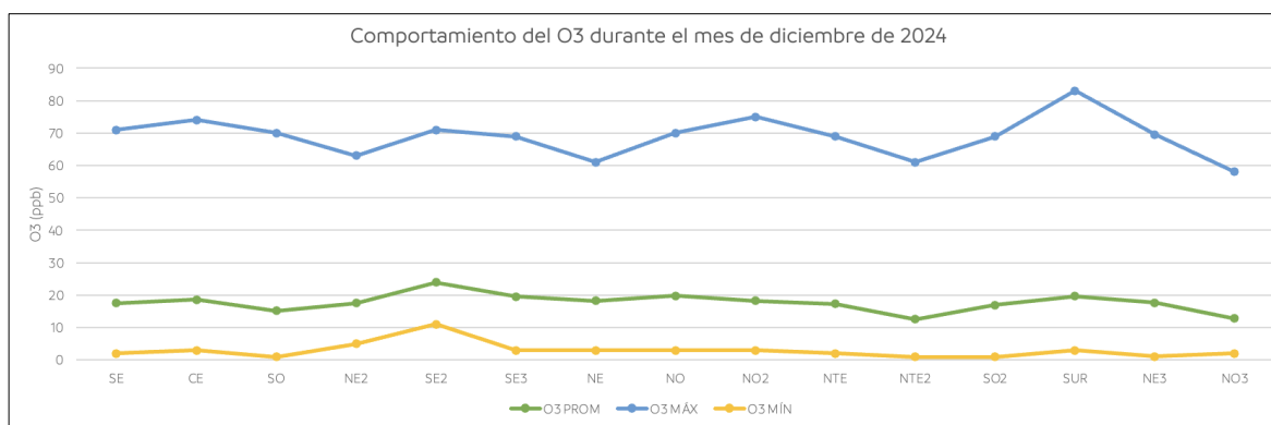
Figura 24. Comportamiento mensual del ozono en la ZMM.
