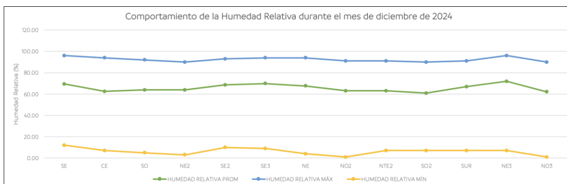
Figura 4. Comportamiento mensual de la humedad relativa en la ZMM.
