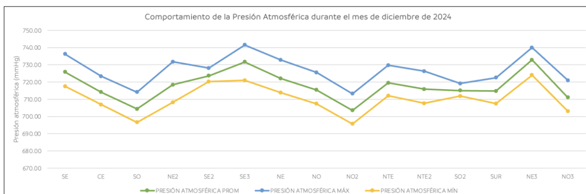
Figura 5. Comportamiento mensual de la presión atmosférica en la ZMM.
