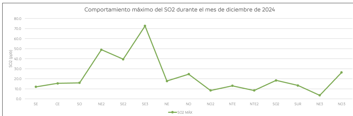
Figura 25. Comportamiento mensual de los máximos del bióxido de azufre en la ZMM.
