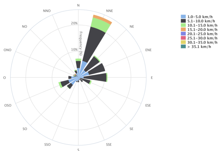
Figura 21. Distribución de la velocidad en la estación NTE2.
