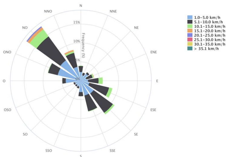
Figura 18. Distribución de la velocidad en la estación SE3.
