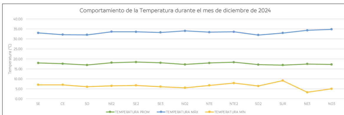
Figura 3. Comportamiento mensual de la temperatura en la ZMM.
