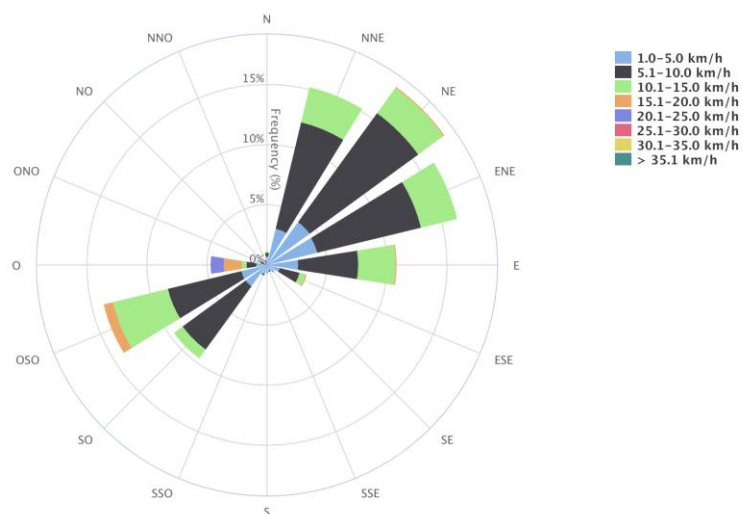
Figura 23. Distribución de la velocidad en la estación NO3.
