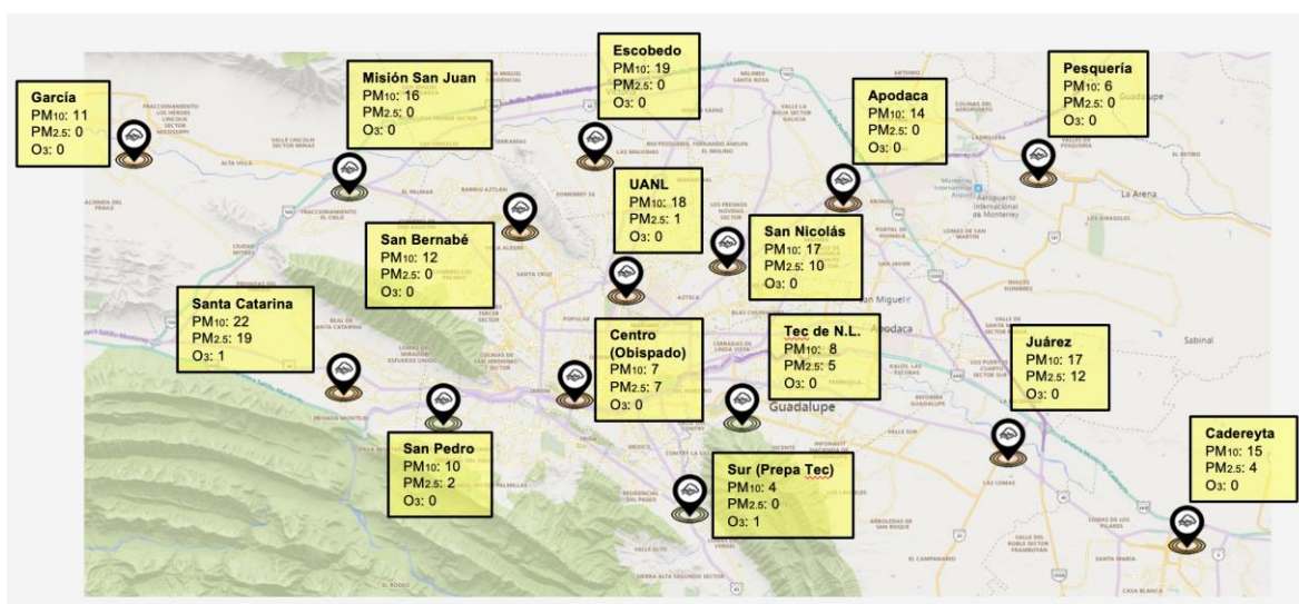
Figura 34. Días superiores al límite normado por estación, por contaminante criterio, del SIMA.
