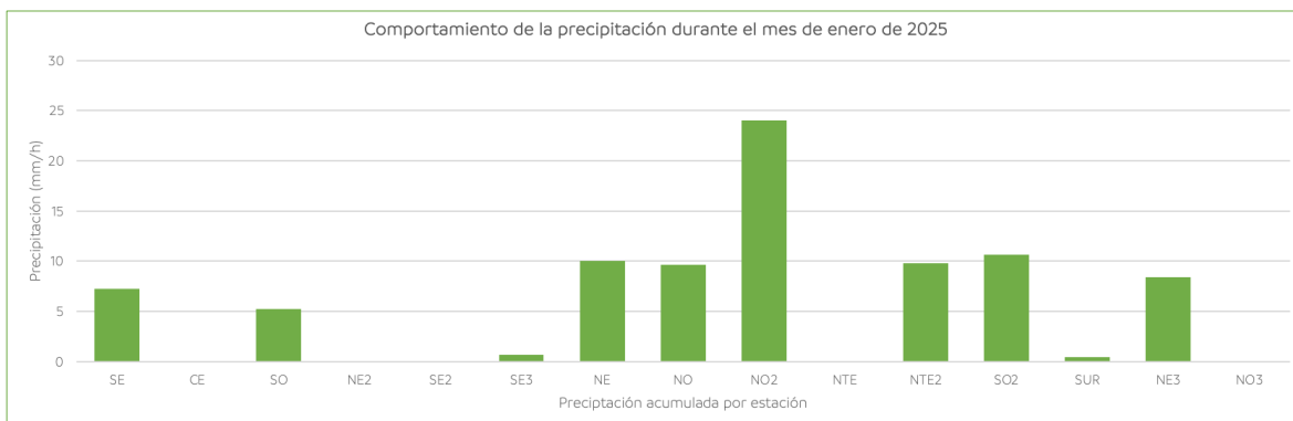
Figura 7. Acumulación de precipitación en estaciones del SIMA.
