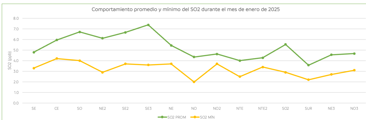
Figura 26. Comportamiento mensual promedio y mínimo del bióxido de azufre en la ZMM.
