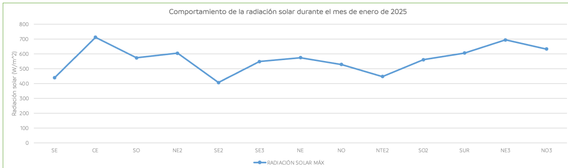
Figura 6. Comportamiento mensual de la radiación solar sobre la ZMM.
