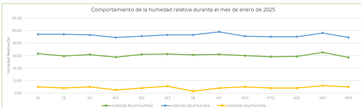
Figura 4. Comportamiento mensual de la humedad relativa en la ZMM.
