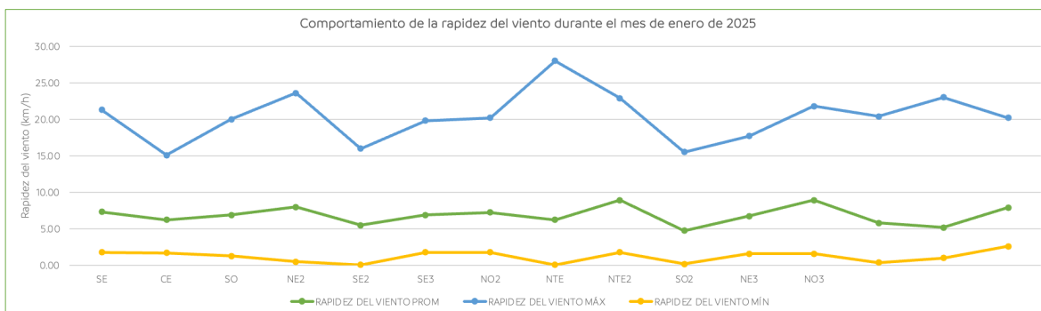
Figura 8. Rapidez del viento para cada estación del SIMA.
