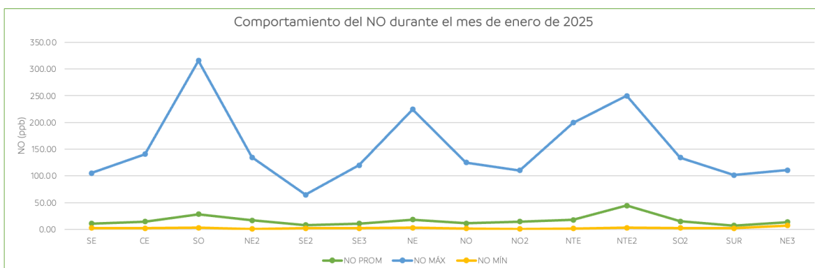
Figura 27. Comportamiento mensual del monóxido de nitrógeno en la ZMM.
