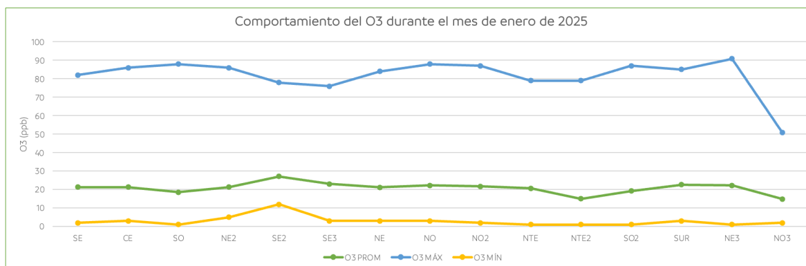
Figura 24. Comportamiento mensual del ozono en la ZMM.
