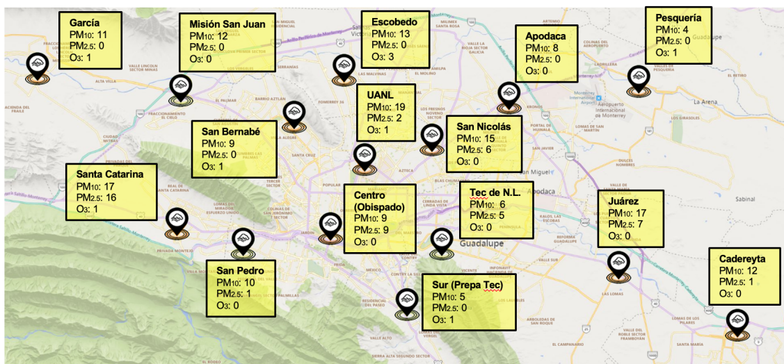
Figura 34. Días superiores al límite normado por estación del SIMA.
