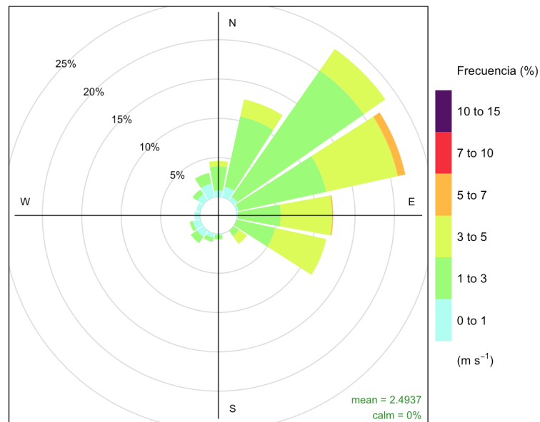
Figura 9. Distribución de la velocidad en la estación CE.
