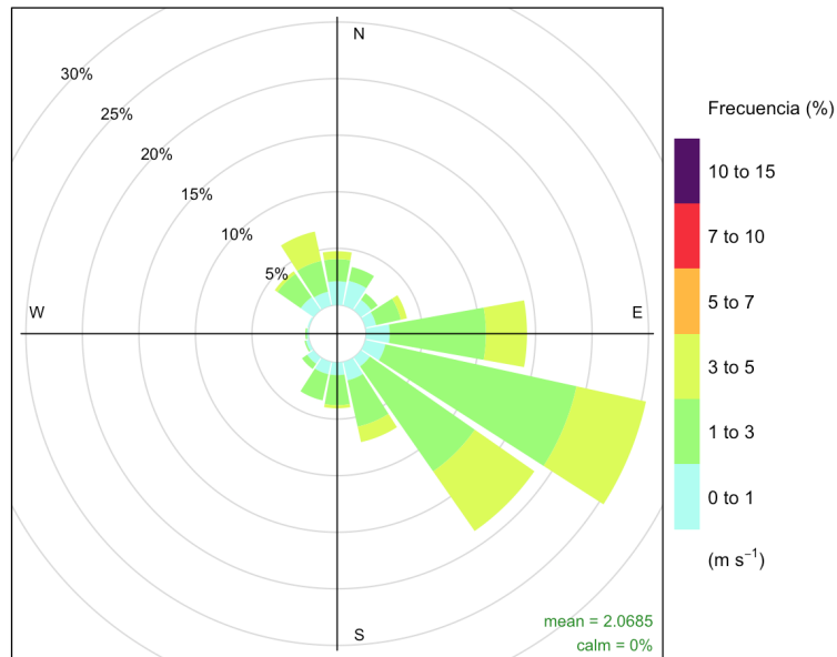
Figura 19. Distribución de la velocidad en la estación SE2.
