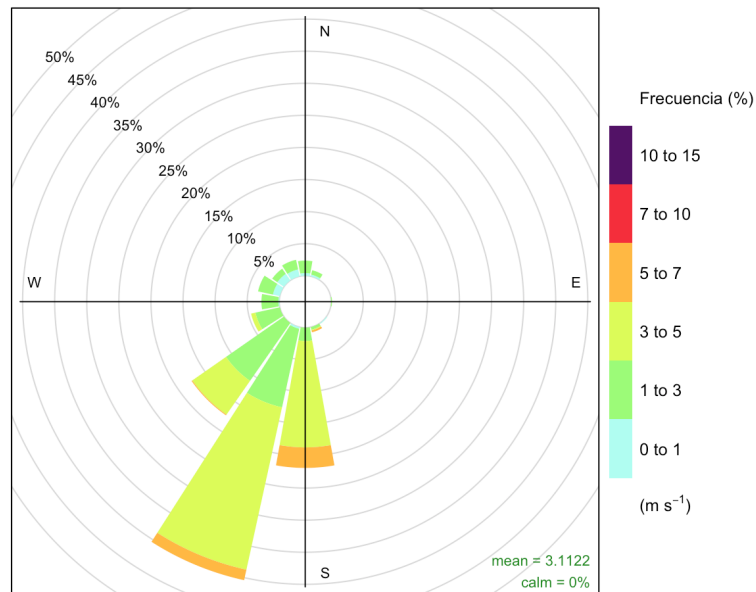
Figura 21. Distribución de la velocidad en la estación SO2.
