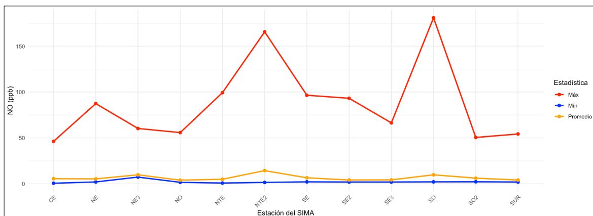
Figura 25. Comportamiento mensual del monóxido de nitrógeno en la ZMM. Las estaciones NO2, NO3 y NE2 no registraron datos.
