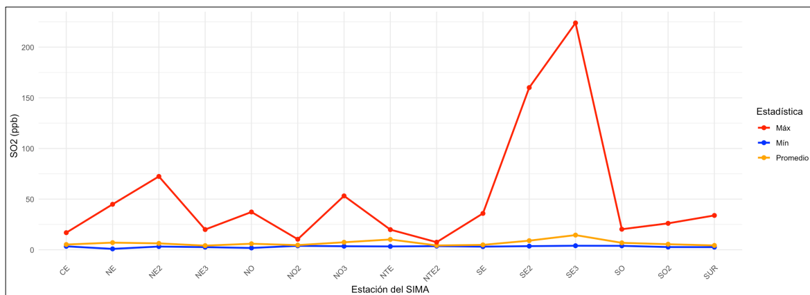
Figura 24. Comportamiento mensual del bióxido de azufre en la ZMM.
