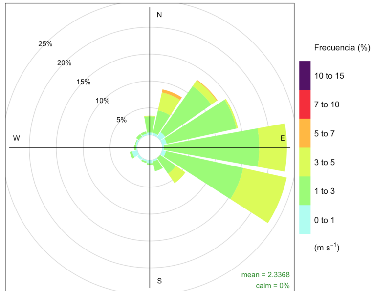
Figura 17. Distribución de la velocidad en la estación NTE2.
