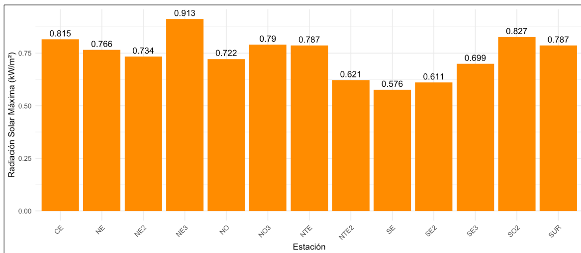
Figura 6. Comportamiento mensual de la radiación solar sobre la ZMM. Los sensores de las estaciones SO y NO2 no cumplieron con los criterios de calidad.
