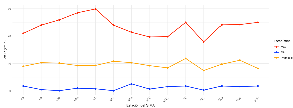
Figura 8. Rapidez del viento para cada estación del SIMA. El instrumento de medición de la estación SO no cumplió con los criterios de calidad.
