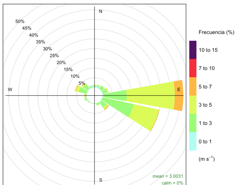
Figura 14. Distribución de la velocidad en la estación NO2.
