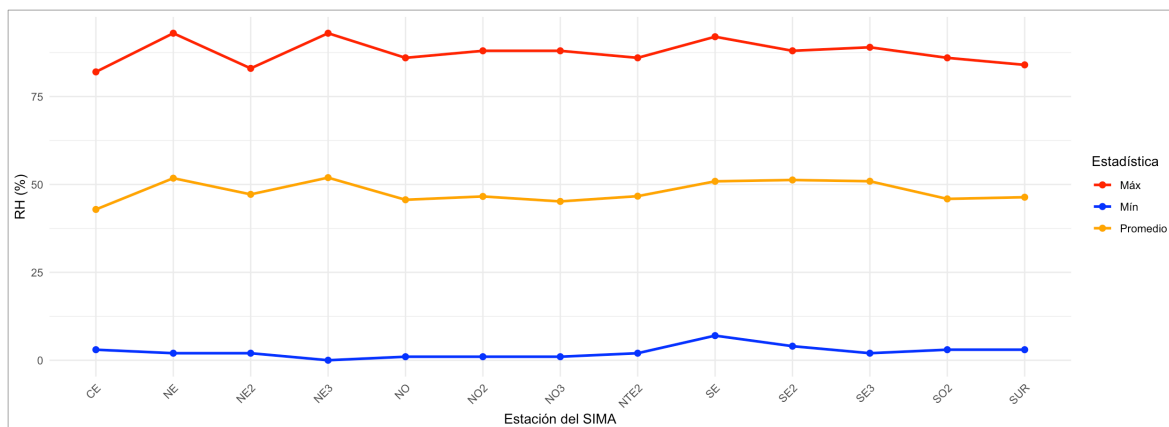
Figura 4. Comportamiento mensual de la humedad relativa en la ZMM. Los sensores de las estaciones NTE y SO estuvieron fuera de operaciones.
