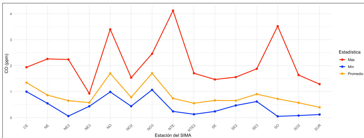
Figura 27. Comportamiento mensual del monóxido de carbono en la ZMM.
