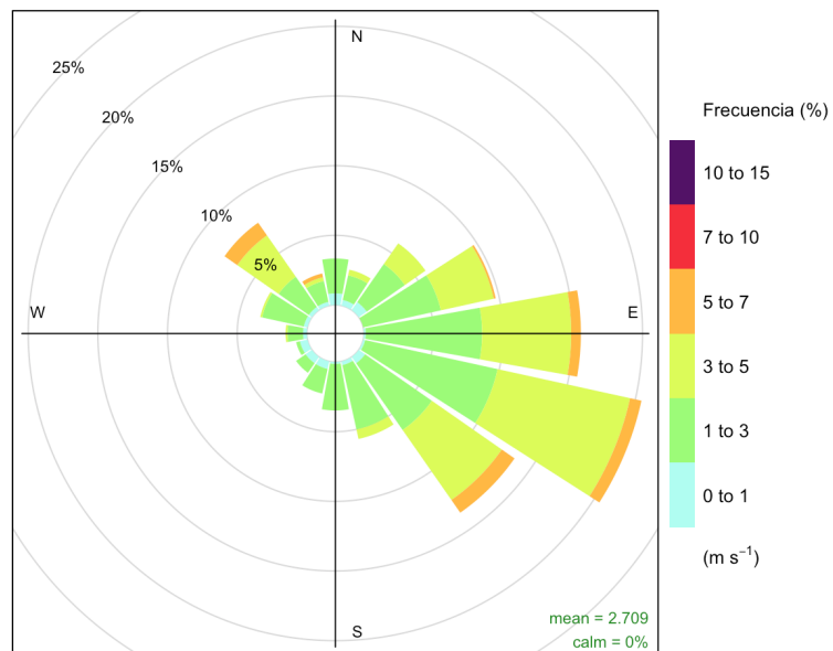
Figura 20. Distribución de la velocidad en la estación SE3.
