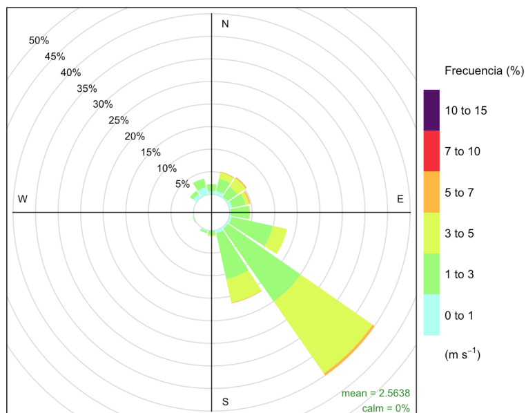
Figura 16. Distribución de la velocidad en la estación NTE.
