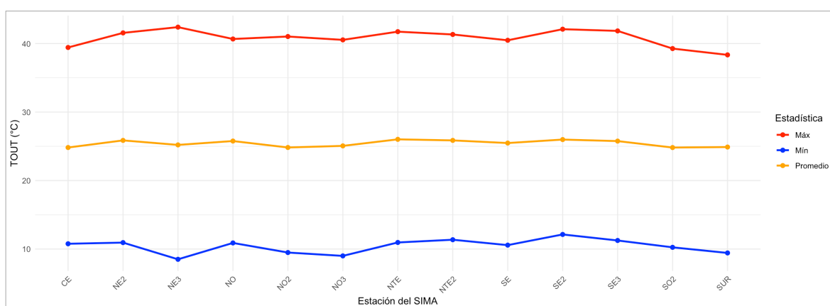
Figura 3. Comportamiento mensual de la temperatura en la ZMM. Los sensores de las estaciones NE y SO estuvieron fuera de operaciones.
