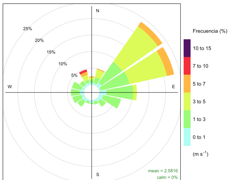
Figura 13. Distribución de la velocidad en la estación NO.
