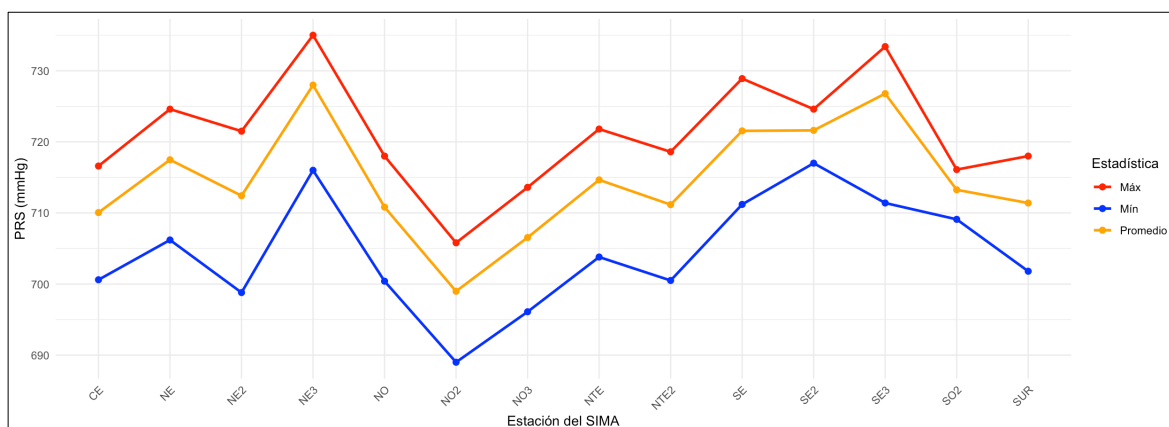
Figura 5. Comportamiento mensual de la presión atmosférica en la ZMM. El sensor de la estación SO no cumplió con los criterios de calidad.
