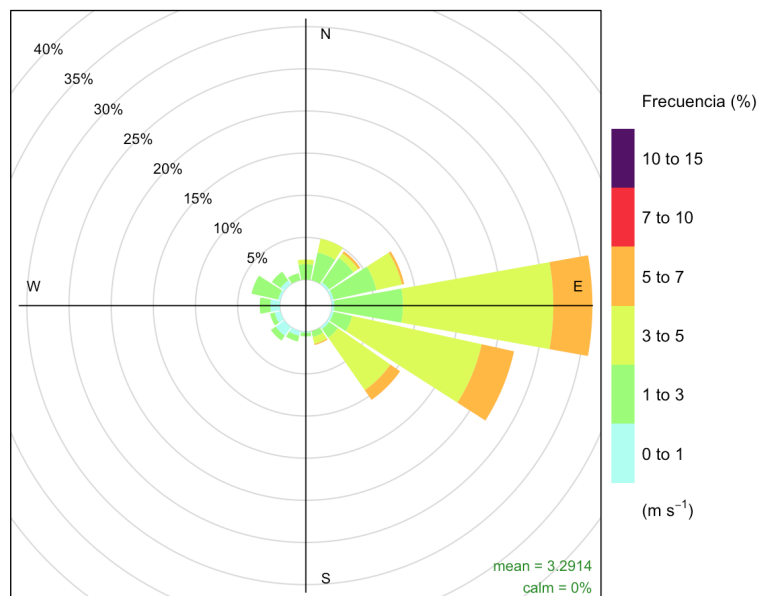
Figura 18. Distribución de la velocidad en la estación SE.
