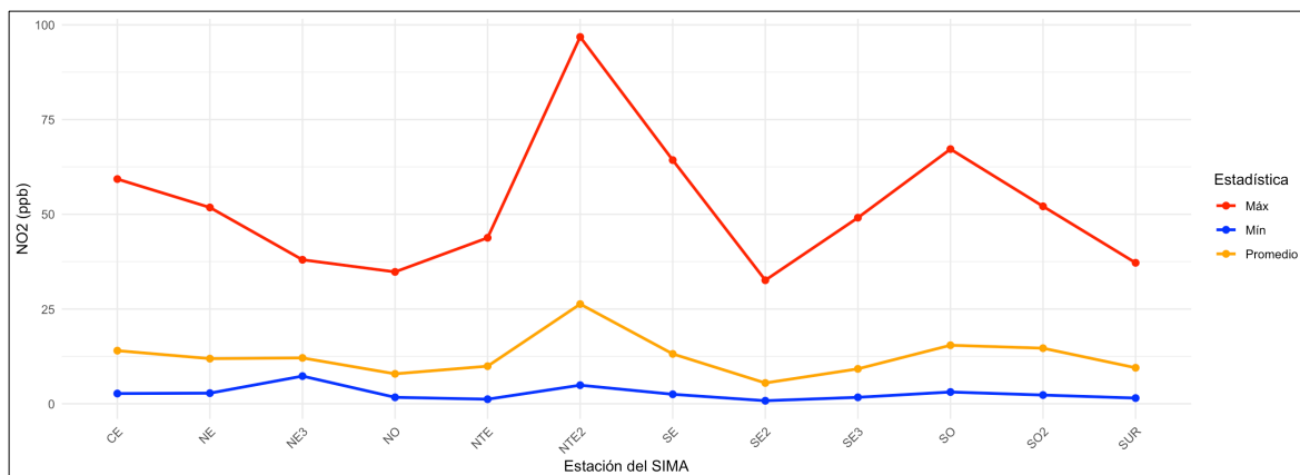
Figura 26. Comportamiento mensual del bióxido de nitrógeno en la ZMM. Las estaciones NO2, NO3 y NE2 no registraron datos.
