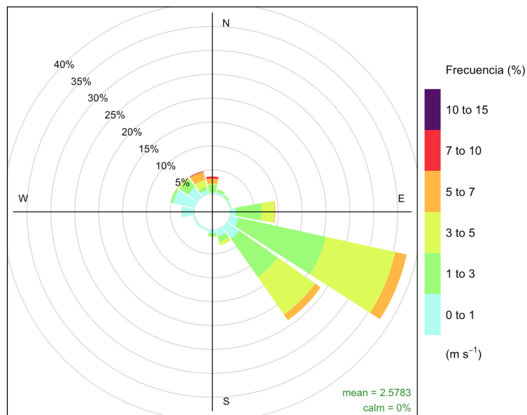
Figura 12. Distribución de la velocidad en la estación NE3.
