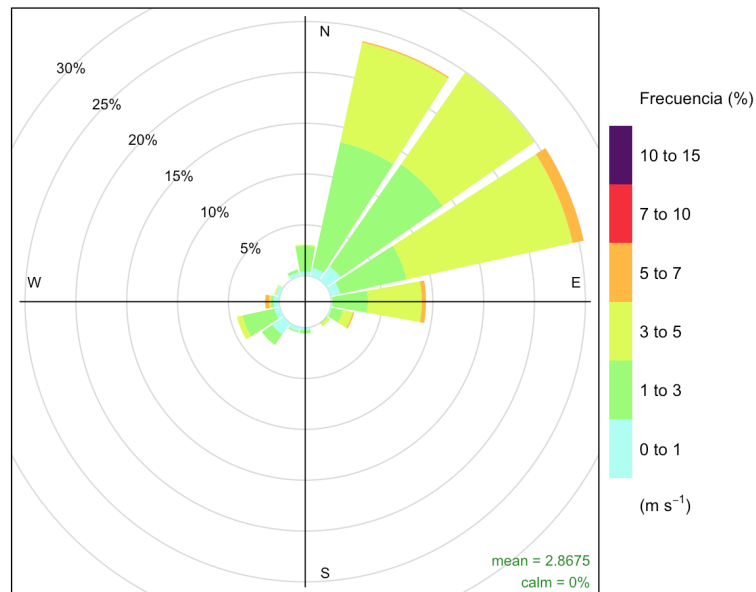
Figura 15. Distribución de la velocidad en la estación NO3.
