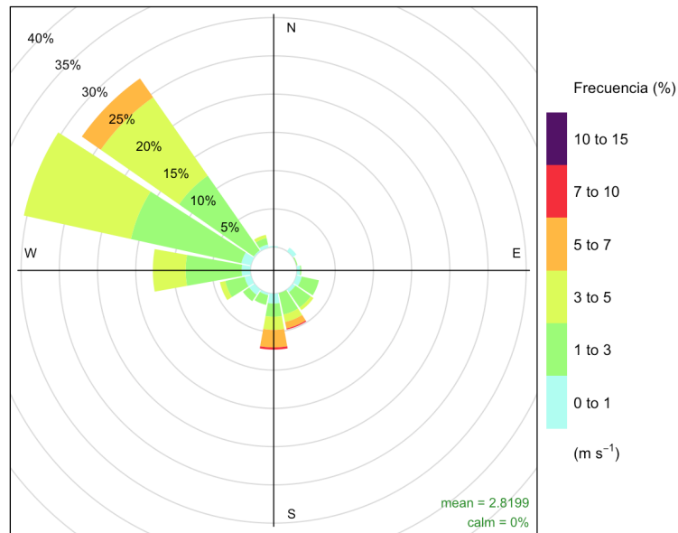
Figura 11. Distribución de la velocidad en la estación NE2.
