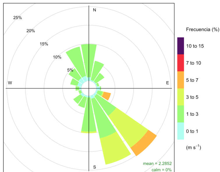
Figura 22. Distribución de la velocidad en la estación SUR.
