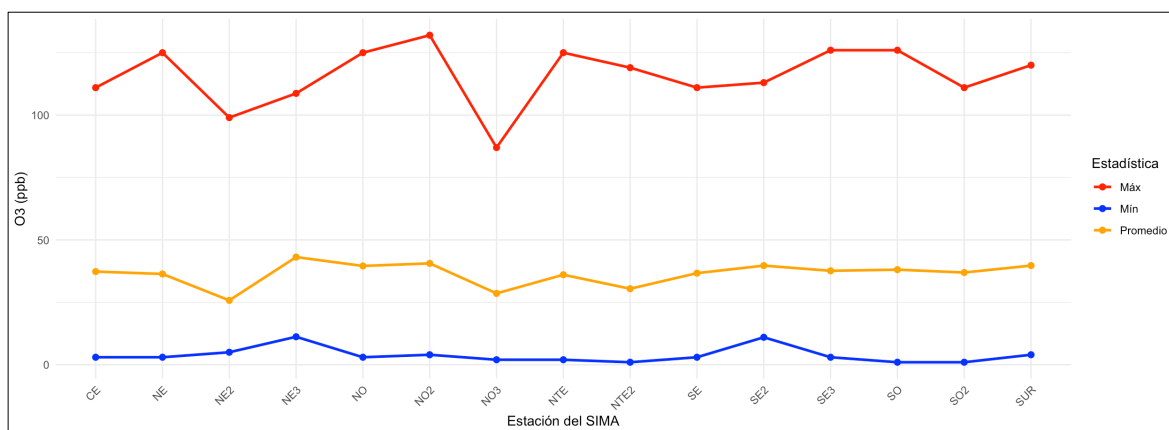
Figura 23. Comportamiento mensual del ozono en la ZMM.
