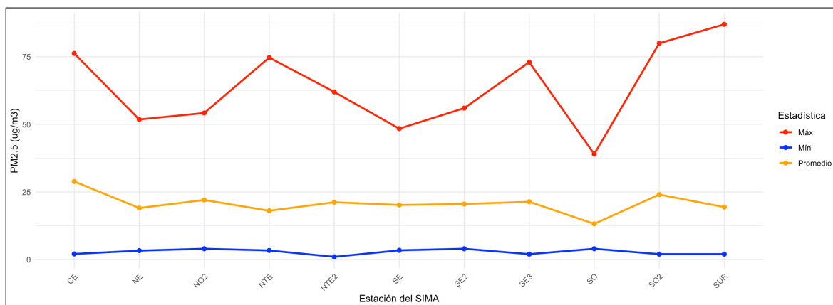
Figura 29. Comportamiento mensual de PM_{2.5} en la ZMM. Las estaciones NE2, NO, NO3 y NE3 no registraron datos.
