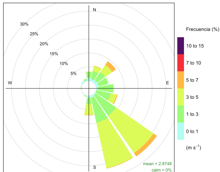
Figura 10. Distribución de la velocidad en la estación NE.
