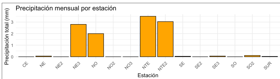
Figura 7. Acumulación de precipitación en estaciones del SIMA. Las estaciones que no indican un registro de lluvia, no aparecen con una barra en color naranja.
