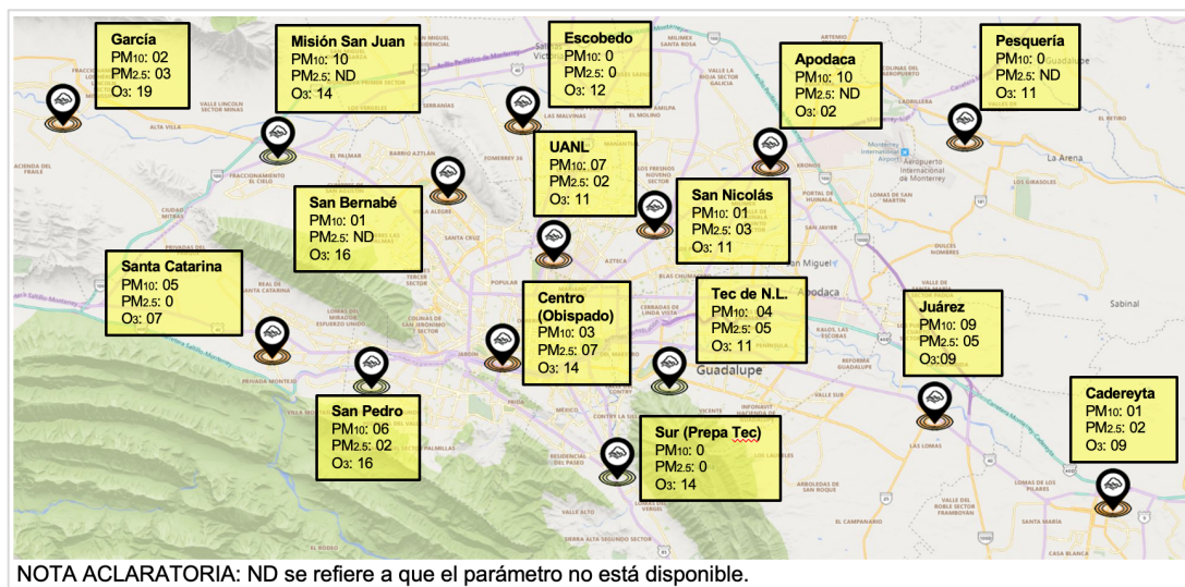
Figura 31. Días superiores al límite normado por estación del SIMA.
