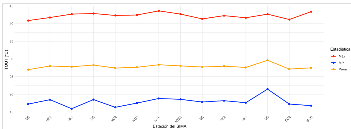
Figura 3. Comportamiento mensual de la temperatura en la ZMM. El sensor de la estación NE estuvo fuera de operación.
