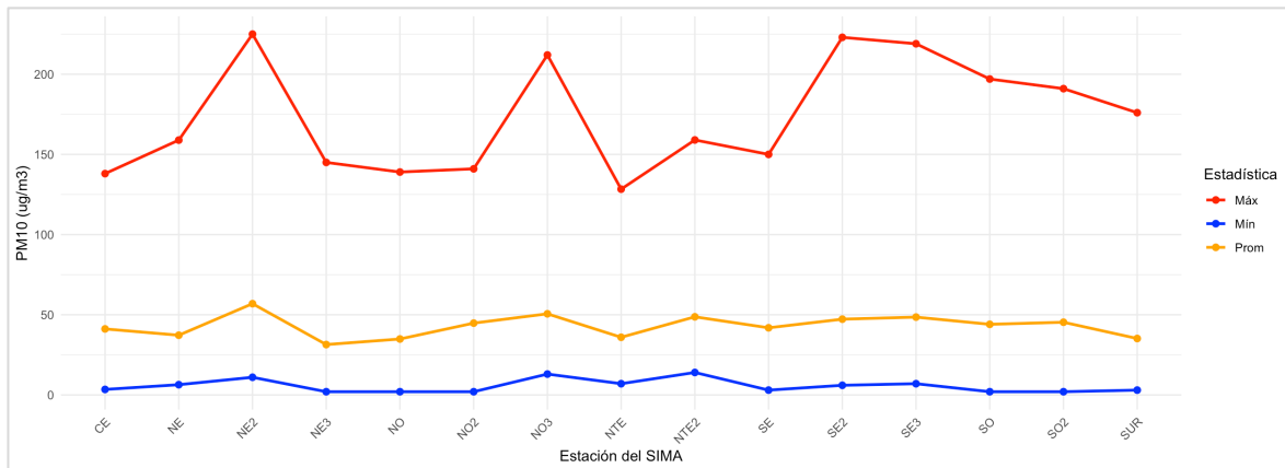
Figura 29. Comportamiento mensual de PM 10 en la ZMM.
