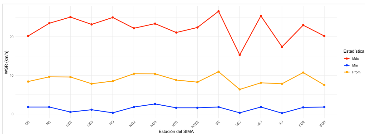
Figura 8. Rapidez del viento para cada estación del SIMA.
