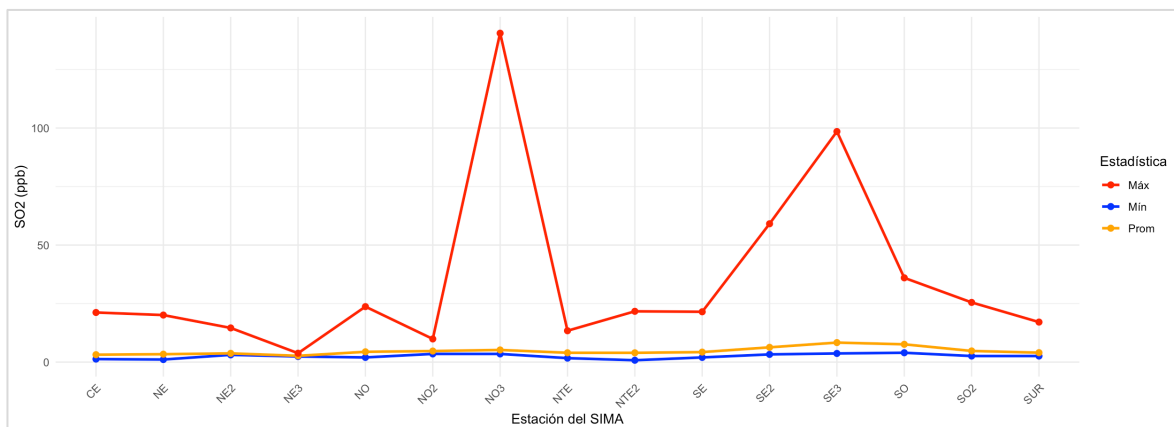
Figura 25. Comportamiento mensual del bióxido de azufre en la ZMM.
