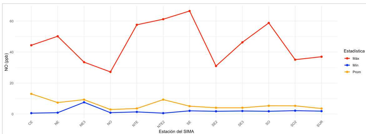
Figura 26. Comportamiento mensual del monóxido de nitrógeno en la ZMM. Las estaciones NO2, NO3 y NE2 no registraron datos.
