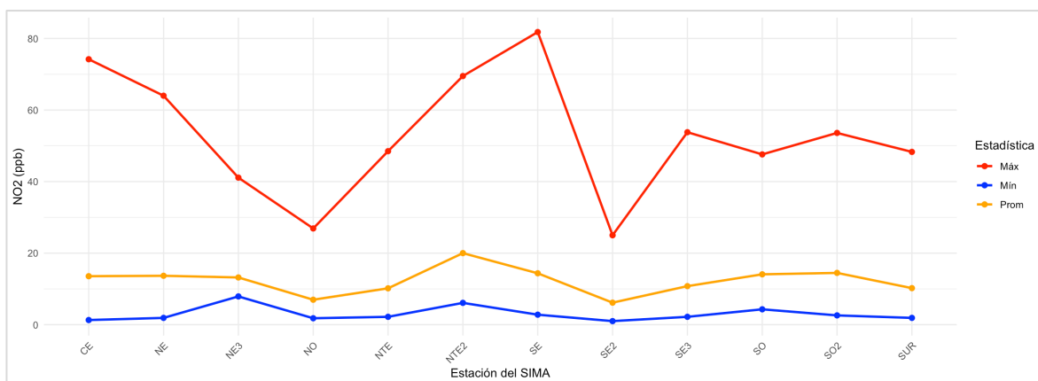
Figura 27. Comportamiento mensual del bióxido de nitrógeno en la ZMM. Las estaciones NO2, NO3 y NE2 no registraron datos.
