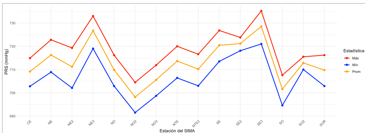
Figura 5. Comportamiento mensual de la presión atmosférica en la ZMM.
