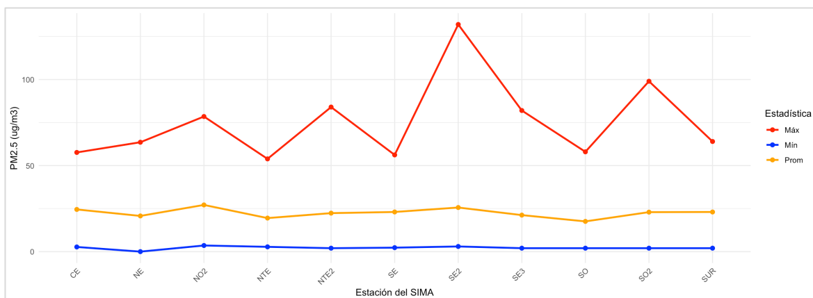
Figura 30. Comportamiento mensual de PM 2.5 en la ZMM. Las estaciones NE2, NO, NO3 y NE3 no registraron datos.
