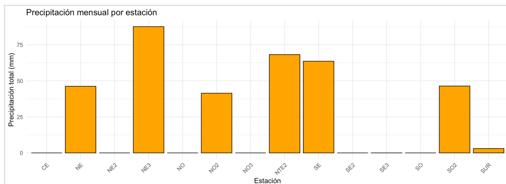
Figura 6. Acumulación de precipitación en estaciones del SIMA. Las estaciones que no indican un registro de lluvia, no aparecen con una barra en color naranja.
