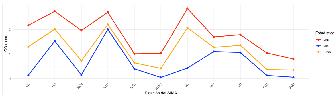
Figura 28. Comportamiento mensual del monóxido de carbono en la ZMM. Las estaciones NE, NE2 y NE3 no fueron reportadas debido a que no superaron criterios de calidad. La estación SE2 no reportó datos.
