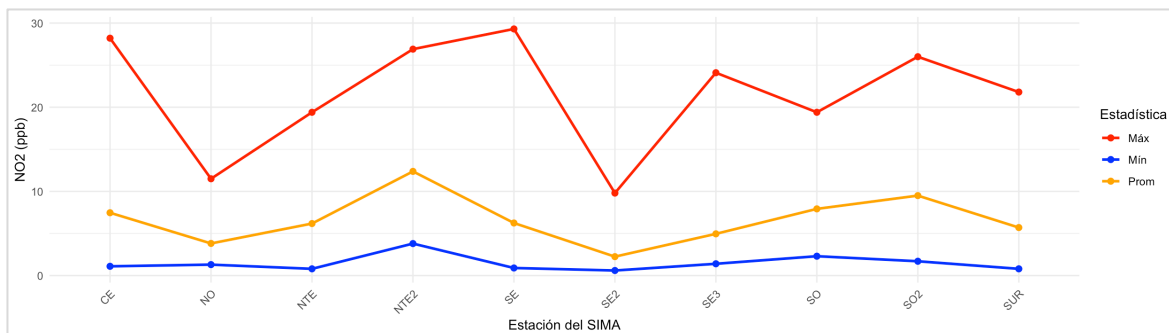
Figura 27. Comportamiento mensual del bióxido de nitrógeno en la ZMM. Las estaciones NO2, NO3, NE y NE3 no fueron reportadas debido a que no superaron criterios de calidad. La estación NE2 no reportó datos.
