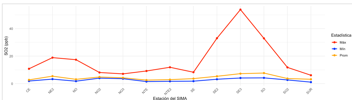
Figura 25. Comportamiento mensual del bióxido de azufre en la ZMM. Las estaciones NE y NE3 no fueron reportadas debido a que no superaron criterios de calidad.
