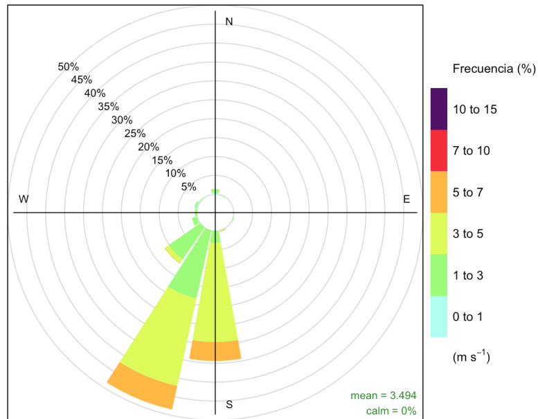
Figura 22. Distribución de la velocidad en la estación SO2.
