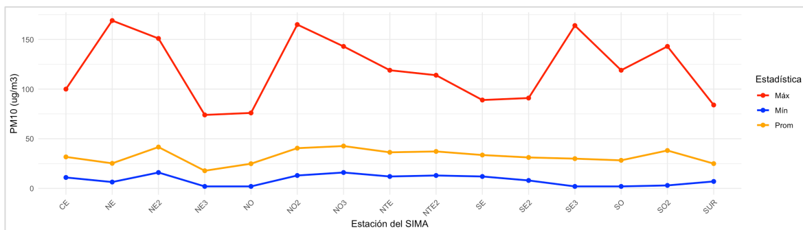
Figura 29. Comportamiento mensual de PM 10 en la ZMM.
