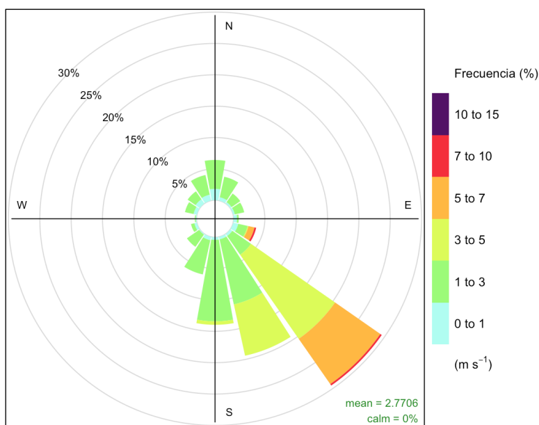
Figura 23. Distribución de la velocidad en la estación SUR.
