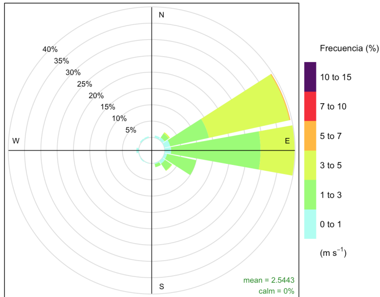
Figura 21. Distribución de la velocidad en la estación SO.
