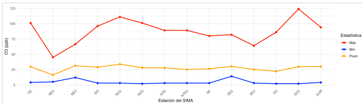
Figura 24. Comportamiento mensual del ozono en la ZMM. La estación NE no fue reportada debido a que no superó criterios de calidad.
