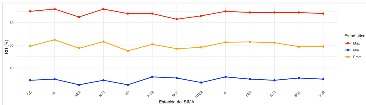
Figura 4. Comportamiento mensual de la humedad relativa en la ZMM. Los sensores de las estaciones NTE y SO estuvieron fuera de operaciones.
