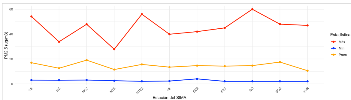
Figura 30. Comportamiento mensual de PM 2.5 en la ZMM. Las estaciones NE2, NE3, NO y NO3 no registraron datos.
