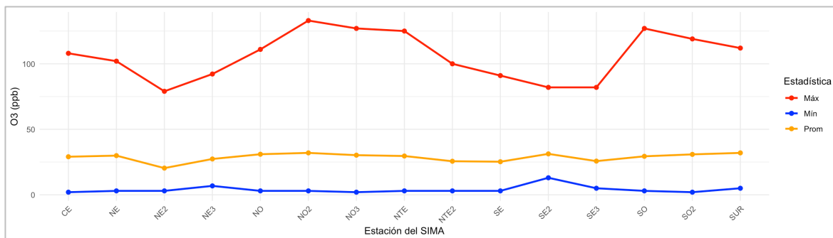
Figura 24. Comportamiento mensual del ozono en la ZMM.
