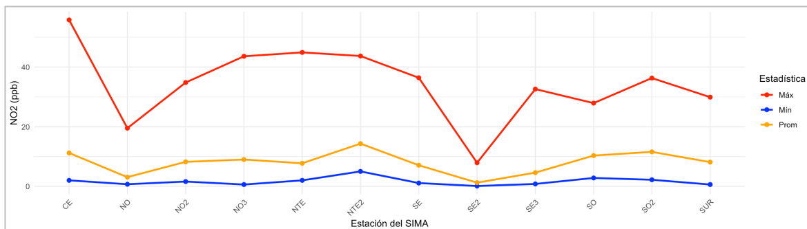
Figura 27. Comportamiento mensual del bióxido de nitrógeno en la ZMM. Las estaciones NE y NE3 no fueron reportadas debido a que no superaron criterios de calidad. La estación NE2 no reportó datos.
