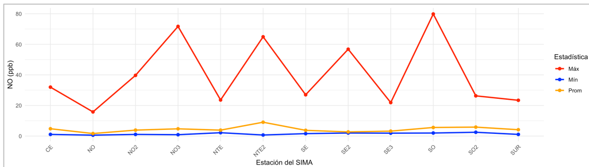
Figura 26. Comportamiento mensual del monóxido de nitrógeno en la ZMM. Las estaciones NE y NE3 no fueron reportadas debido a que no superaron criterios de calidad. La estación NE2 no reportó datos.
