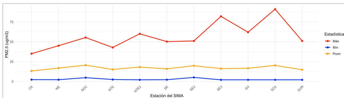
Figura 30. Comportamiento mensual de PM 2.5 en la ZMM. La estación NO3 no fue reportada debido a que no superaro criterios de calidad. Las estaciones NE2, NE3 y NO no registraron datos.
