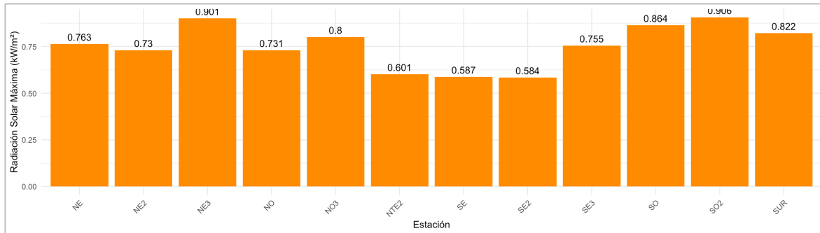
Figura 7. Comportamiento mensual de la radiación solar sobre la ZMM. Los sensores de las estaciones CE, NTE y NO2 no cumplieron con los criterios de calidad.
