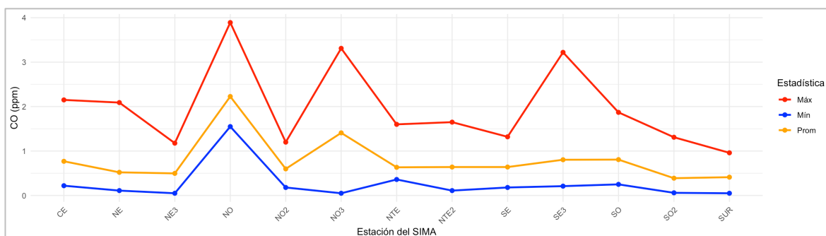
Figura 28. Comportamiento mensual del monóxido de carbono en la ZMM. Las estaciones NE2 y SE2 no fueron reportadas debido a que no superaron criterios de calidad.
