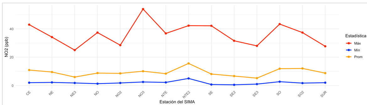
Figura 27. Comportamiento mensual del bióxido de nitrógeno en la ZMM. La estación NE2 no reportó datos.
