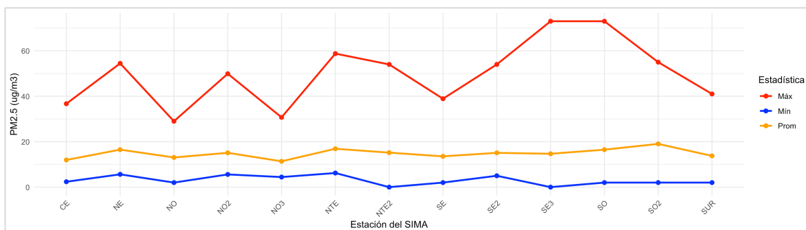
Figura 30. Comportamiento mensual de PM 2.5 en la ZMM. Las estaciones NE2 y NE3 no registraron datos.
