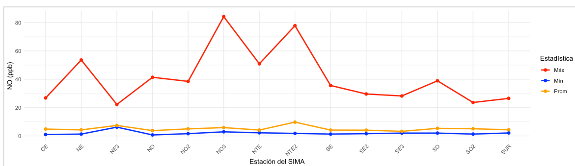
Figura 26. Comportamiento mensual del monóxido de nitrógeno en la ZMM. La estación NE2 no reportó datos.
