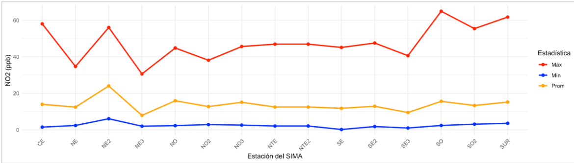
Figura 27. Comportamiento mensual del bióxido de nitrógeno en la ZMM.
