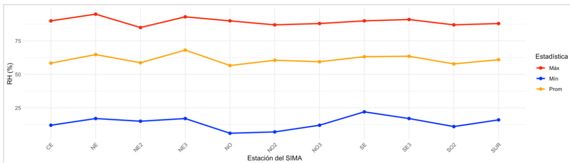
Figura 4. Comportamiento mensual de la humedad relativa en la ZMM. Los sensores de las estaciones NTE, NTE2, SE2 y SO estuvieron fuera de operaciones.
