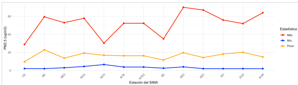
Figura 30. Comportamiento mensual de PM 2.5 en la ZMM. Las estaciones NE2 y NO no registraron datos.
