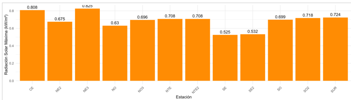
Figura 7. Comportamiento mensual de la radiación solar sobre la ZMM. Los sensores de las estaciones NE, NO2 y SE3 estuvieron fuera de operación.
