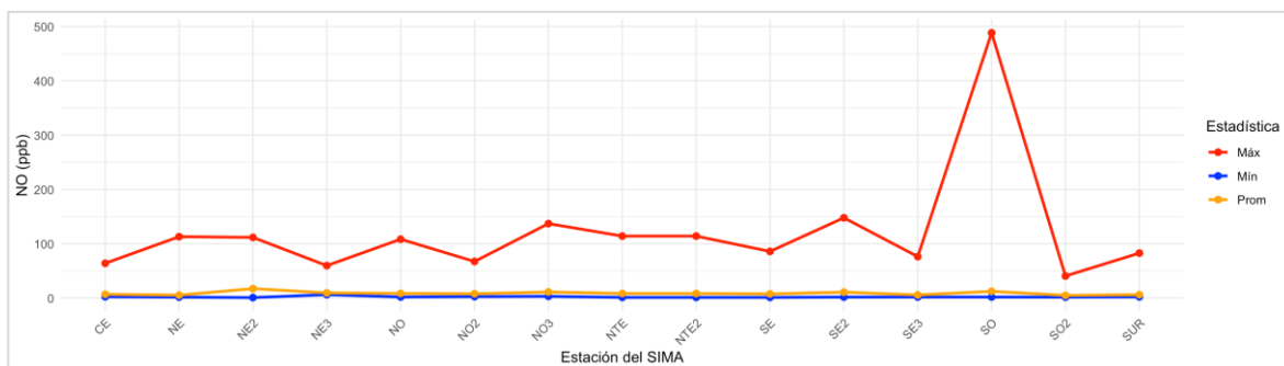
Figura 26. Comportamiento mensual del monóxido de nitrógeno en la ZMM.
