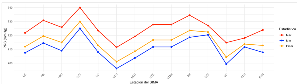
Figura 5. Comportamiento mensual de la presión atmosférica en la ZMM. El sensor de las estación SE3 estuvo fuera de operación.
