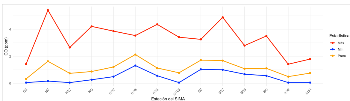
Figura 28. Comportamiento mensual del monóxido de carbono en la ZMM. El analizador de la estación NE3 estuvo fuera de operación.
