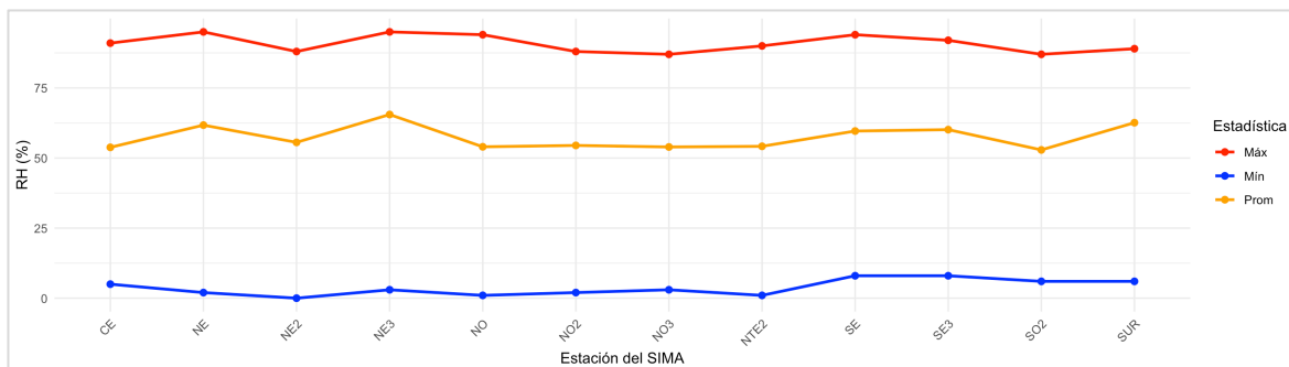
Figura 4. Comportamiento mensual de la humedad relativa en la ZMM. Los sensores de las estaciones NTE, SE2 y SO estuvieron fuera de operaciones.
