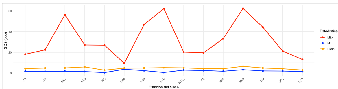
Figura 25. Comportamiento mensual del bióxido de azufre en la ZMM.
