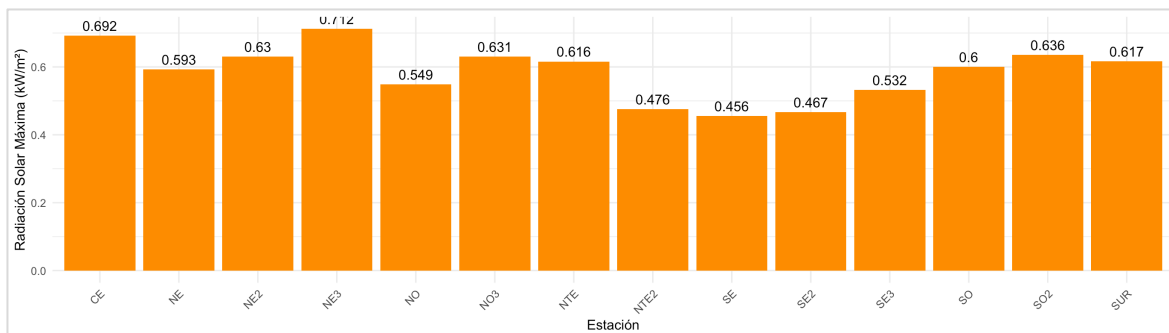
Figura 7. Comportamiento mensual de la radiación solar sobre la ZMM. El sensor de la estación NO2 estuvo fuera de operación.
