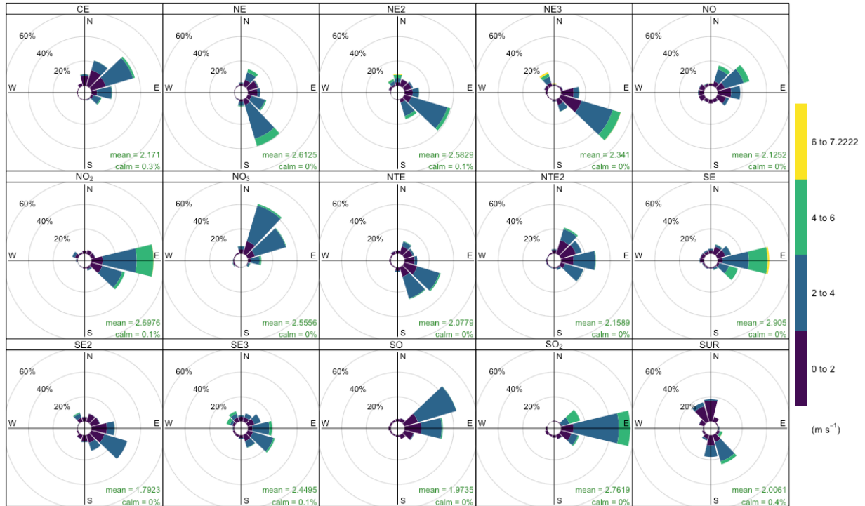
Figura 9. Distribuciones de la velocidad durante el mes de abril en cada estación del SIMA.
