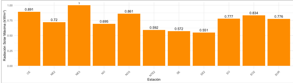
Figura 7. Comportamiento mensual de la radiación solar sobre la ZMM. Los sensores de las estaciones NE, NO2, NTE y SE3 estuvieron fuera de operaciones.
