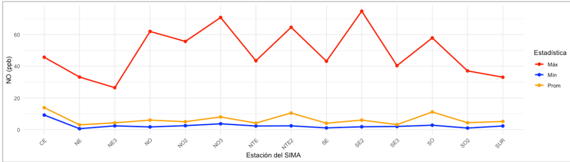
Figura 12. Comportamiento mensual del monóxido de nitrógeno en la ZMM. El analizador de la estación NE2 estuvo fuera de operaciones.
