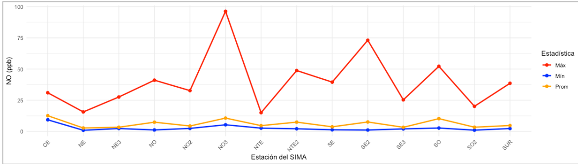
Figura 12. Comportamiento mensual del monóxido de nitrógeno en la ZMM. El analizador de la estación NE2 estuvo fuera de operaciones. El equipo de la estación NE2 estuvo fuera de operación.
