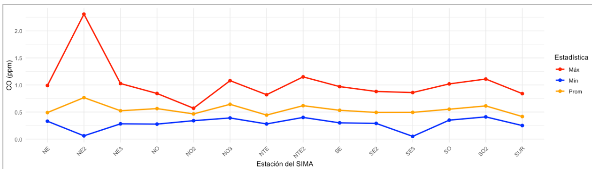
Figura 14. Comportamiento mensual del monóxido de carbono en la ZMM. El equipo de la estación CE estuvo fuera de operación.
