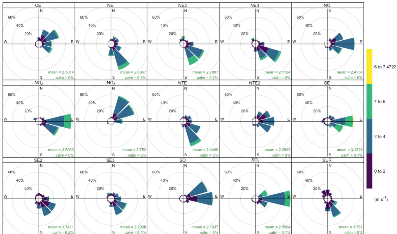
Figura 9. Distribuciones de la velocidad durante el mes de mayo en cada estación del SIMA.
