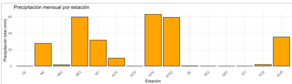
Figura 6. Acumulación de precipitación en las estaciones del SIMA. Las estaciones que no indican un registro de lluvia, no aparecen con una barra en color naranja.
