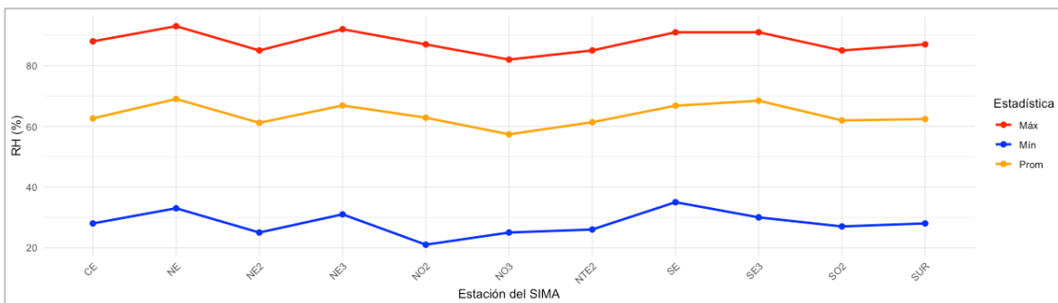
Figura 4. Comportamiento mensual de la humedad relativa en la ZMM. Los sensores de las estaciones NO, NTE, SE2 y SO estuvieron fuera de operaciones.
