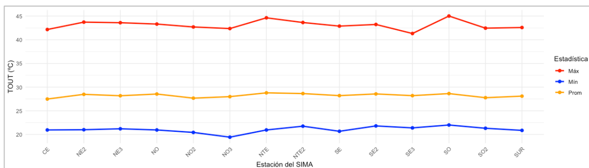
Figura 3. Comportamiento mensual de la temperatura en la ZMM. El sensor de la estación NE estuvo fuera de operaciones.
