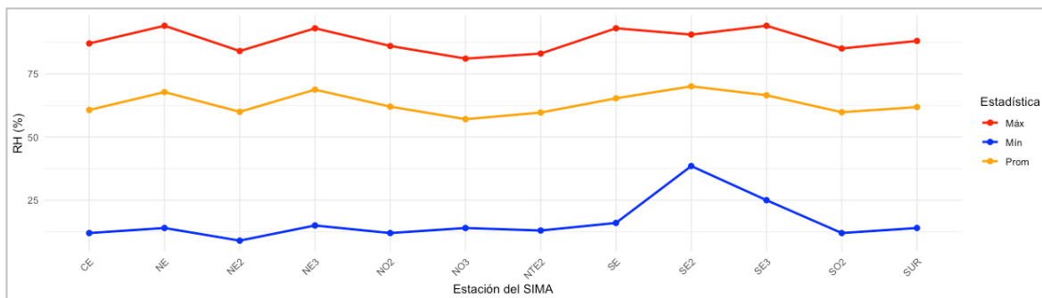
Figura 4. Comportamiento mensual de la humedad relativa en la ZMM. Los sensores de las estaciones NO, NTE y SO estuvieron fuera de operaciones.
