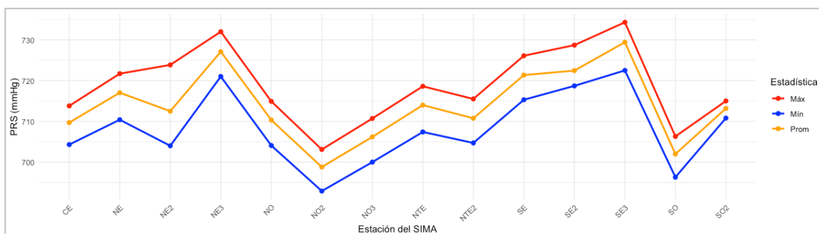
Figura 5. Comportamiento mensual de la presión atmosférica en la ZMM. El sensor de las estación SUR estuvo fuera de operaciones.
