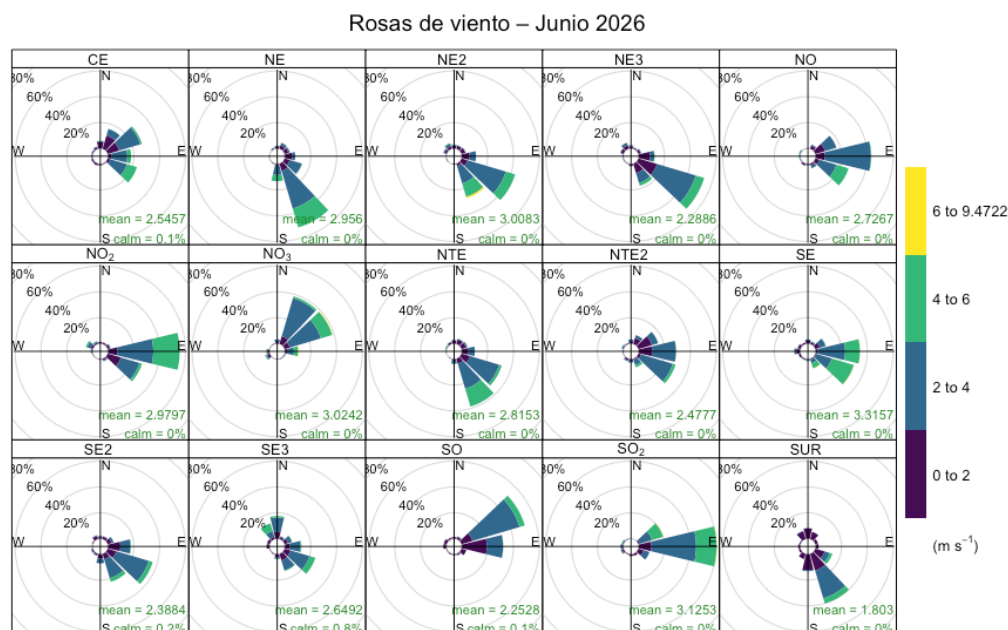
Figura 9. Distribuciones de la velocidad durante el mes de junio en cada estación del SIMA.
