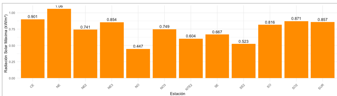
Figura 7. Comportamiento mensual de la radiación solar sobre la ZMM. Los sensores de las estaciones NO2, NTE y SE3 estuvieron fuera de operaciones.
