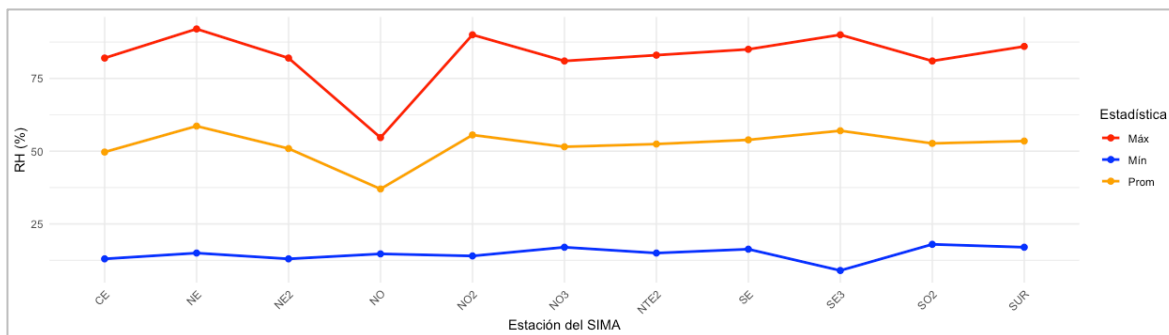
Figura 4. Comportamiento mensual de la humedad relativa en la ZMM. Los sensores de las estaciones NE3, NTE, SE2 y SO estuvieron fuera de operaciones.
