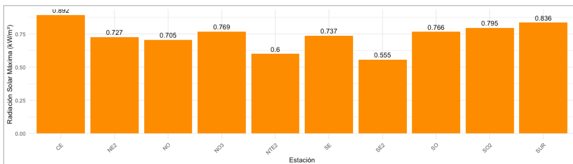
Figura 7. Comportamiento mensual de la radiación solar sobre la ZMM. Los sensores de las estaciones NE, NE3, NO2, NTE y SE3 estuvieron fuera de operaciones.
