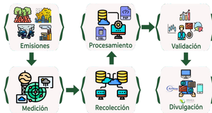
Figura 2. Ciclo de tratamiento de los datos del SIMA.
