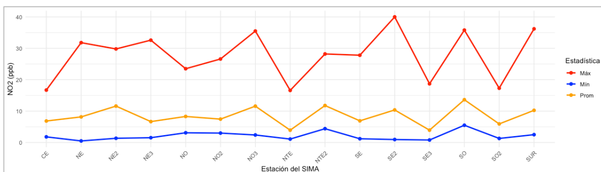
Figura 13. Comportamiento mensual del bióxido de nitrógeno en la ZMM.
