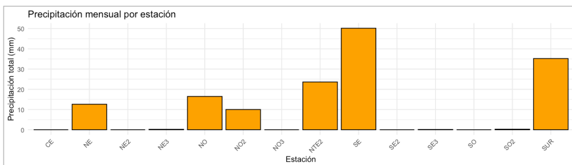
Figura 6. Acumulación de precipitación en las estaciones del SIMA. Las estaciones que no indican un registro de lluvia, no aparecen con una barra en color naranja. La estación NTE no aparece en el gráfico debido a que el sensor estuvo fuera de operación.
