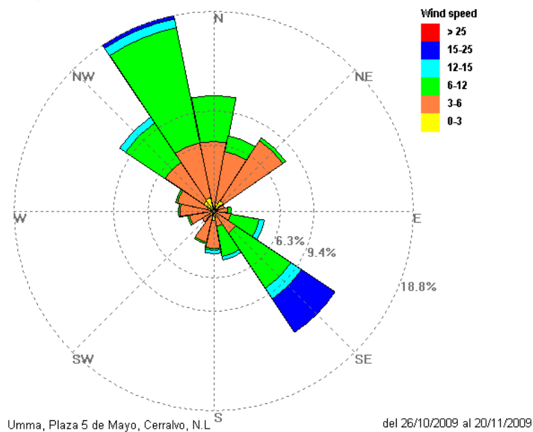
Fig. 2. Análisis de la rosa de vientos durante el monitoreo atmosférico en el municipio de Cerralvo, N.L.
