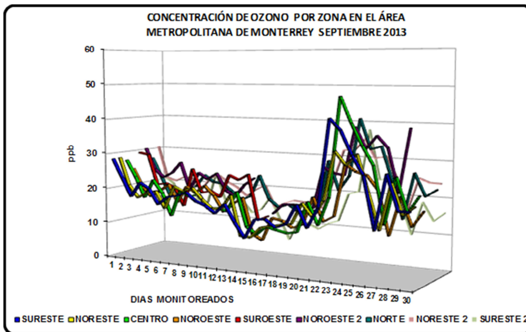
Figura 17: Promedio de concentración diaria de Ozono por zona en el AMM
