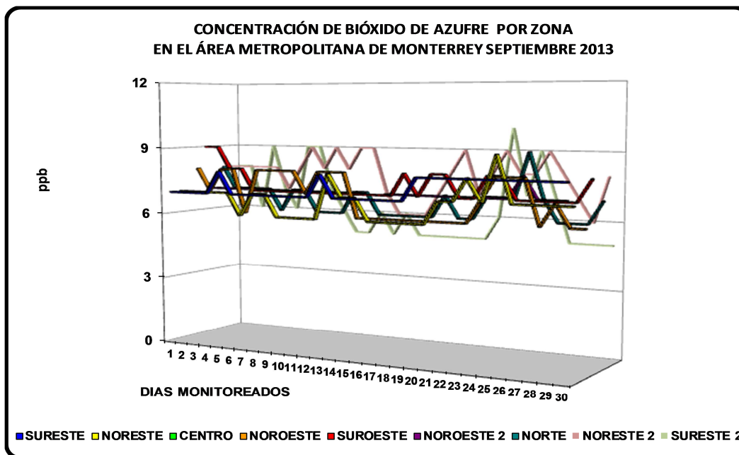
Figura 13: Concentración diaria de Bióxido de Azufre en el AMM
