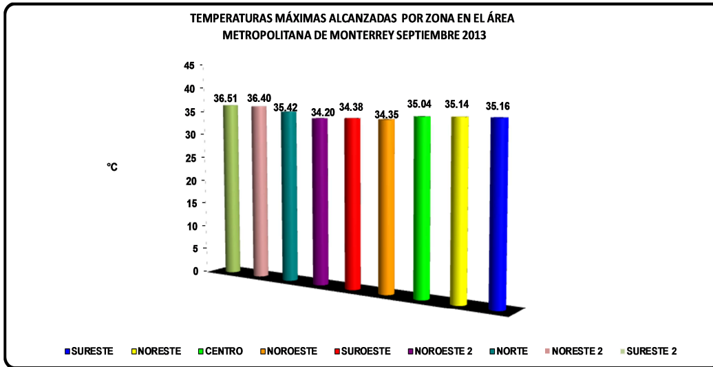
Figura 2: Temperatura Máxima por Zona en el AMM
