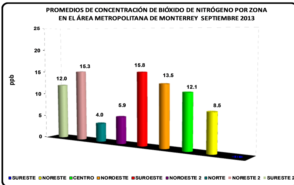
Figura 16: Promedio de concentración de Bióxido de Nitrógeno por zona en el AMM
