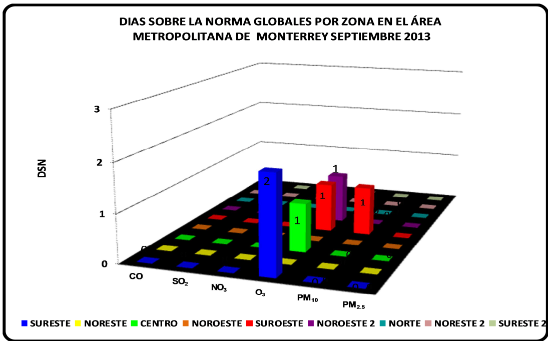
Figura 21: Días sobre la Norma globales por zona en el AMM
