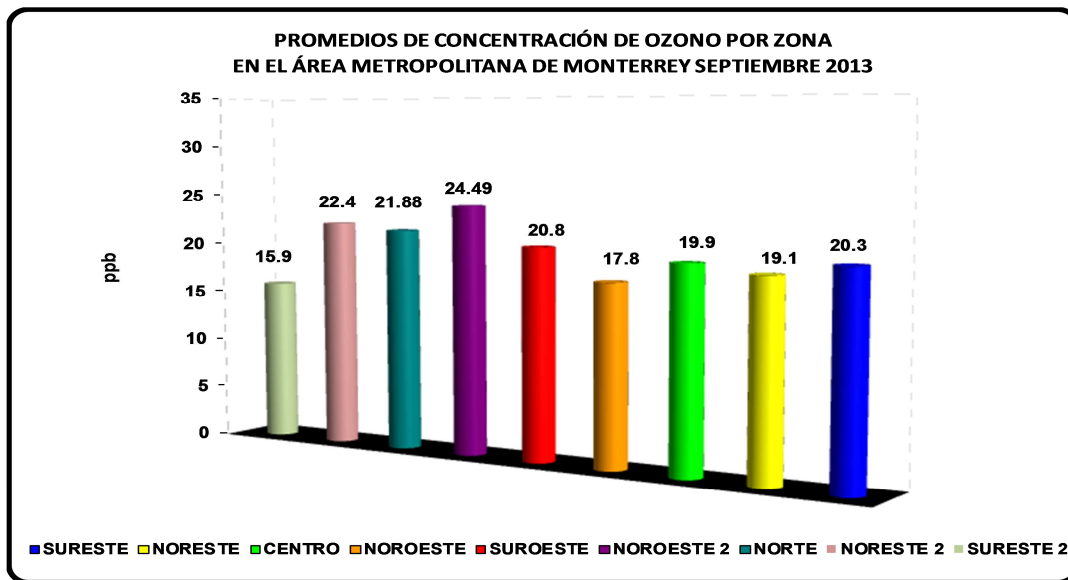
Figura 18: Promedio de concentración de Ozono por zona en el AMM
