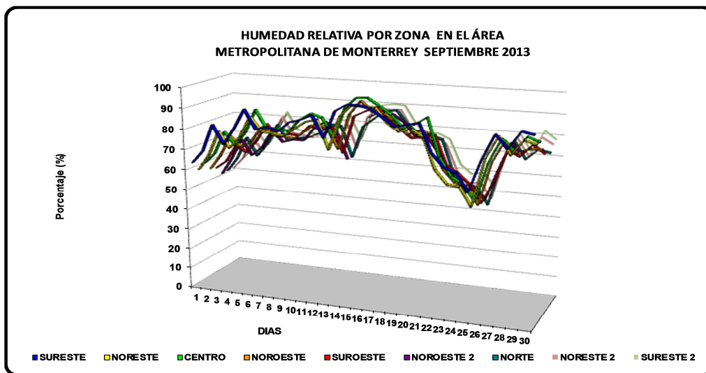
Figura 4: Humedad relativa por zona en el AMM
