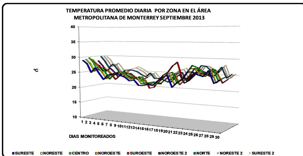
Figura 1: Temperatura Promedio Diaria por zona en el AMM
