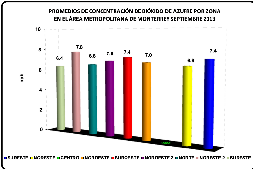
Figura 14: Promedio de concentración de Bióxido de Azufre por zona en el AMM
