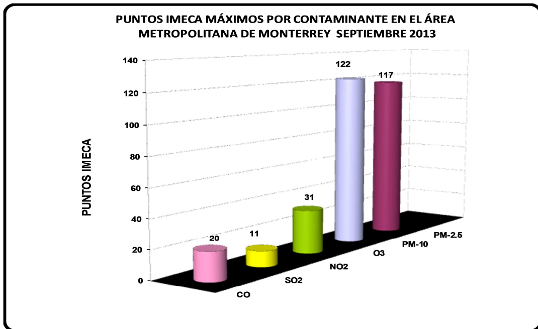
Figura 22: IMECA máximo por contaminante en el AMM
