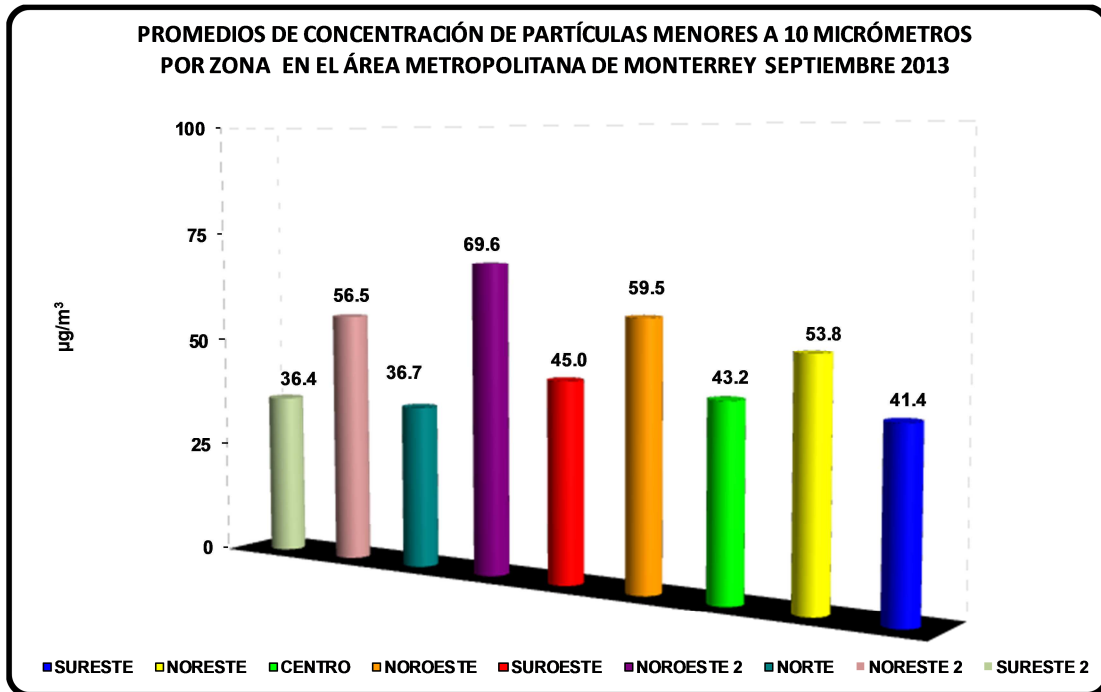
Figura 20: Promedio de concentración de partículas menores a 10 micrómetros por zona en el AMM
