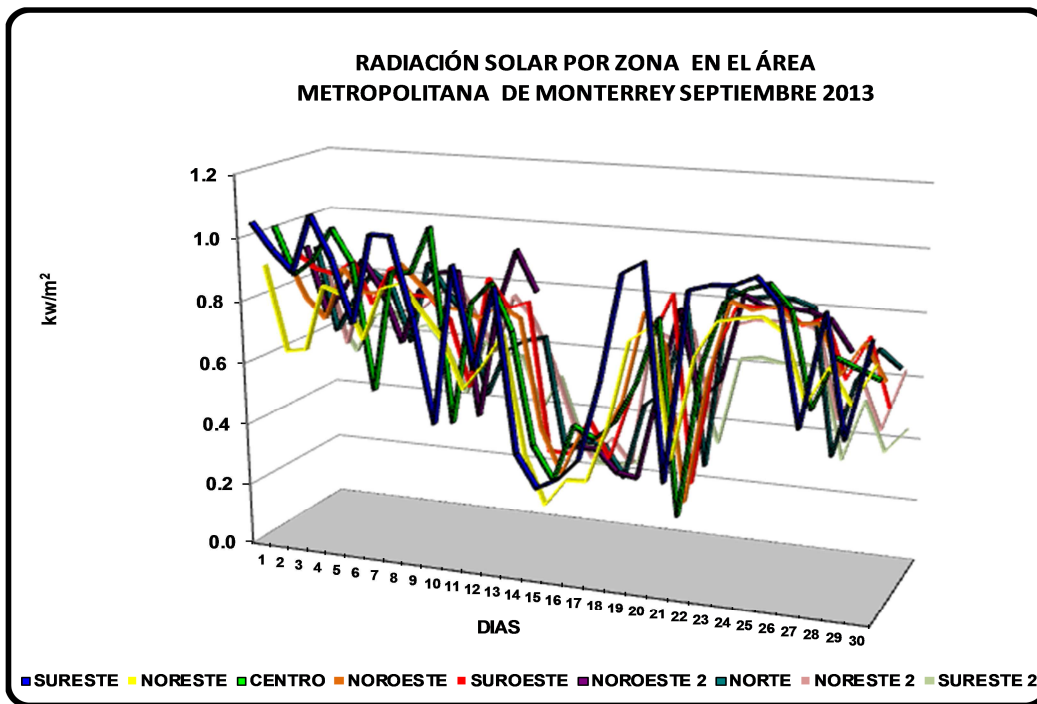
Figura 8: Radiación solar por zona en el AMM
