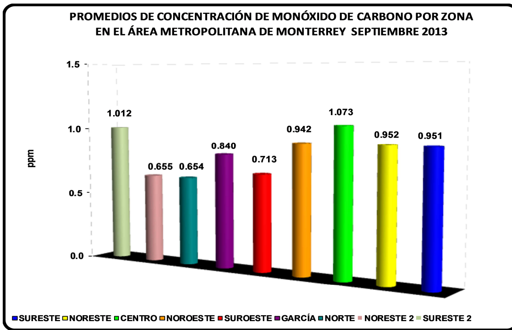
Figura 12: Promedios de concentración de Monóxido de Carbono por zona en el AMM
