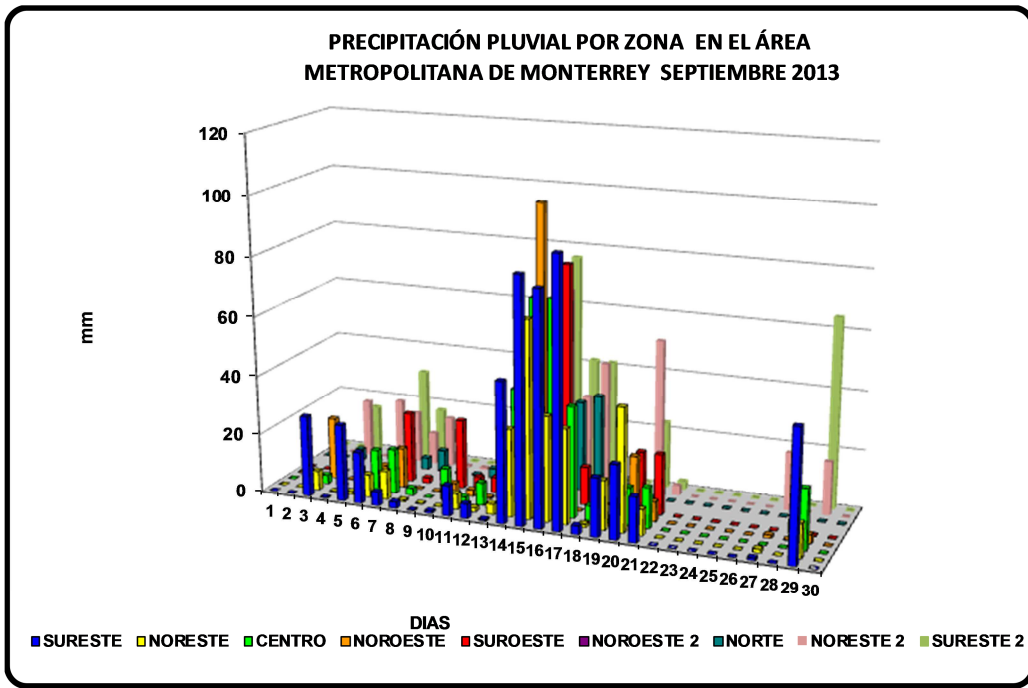
Figura 6: Precipitación pluvial por zona en el AMM
