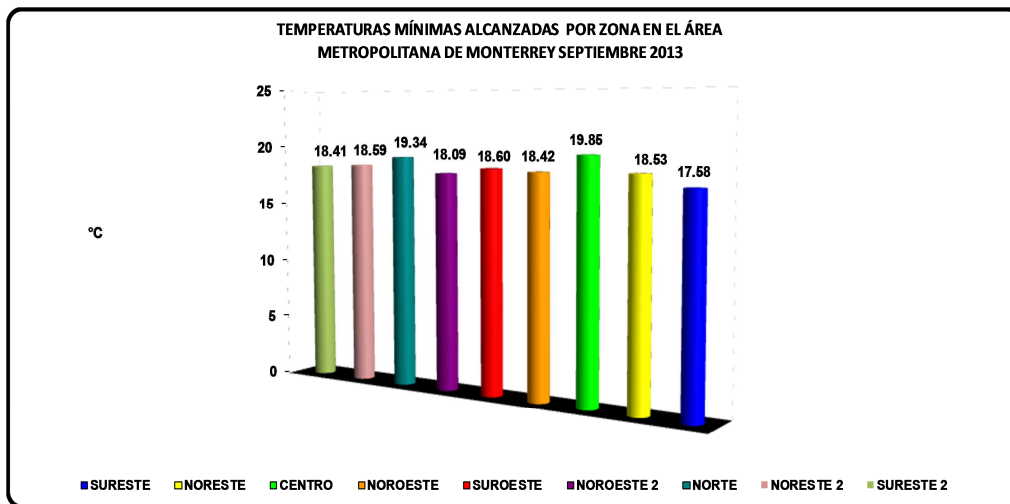
Figura 3: Temperatura Mínima por zona en el AMM
