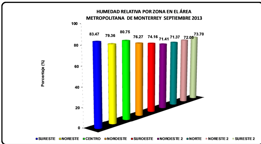
Figura 5: Humedad relativa promedio por zona en el AMM
