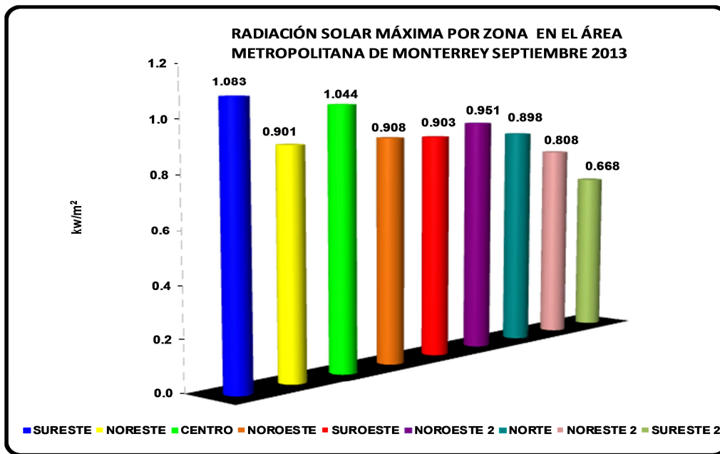
Figura 9: Radiación solar máxima por zona en el AMM
