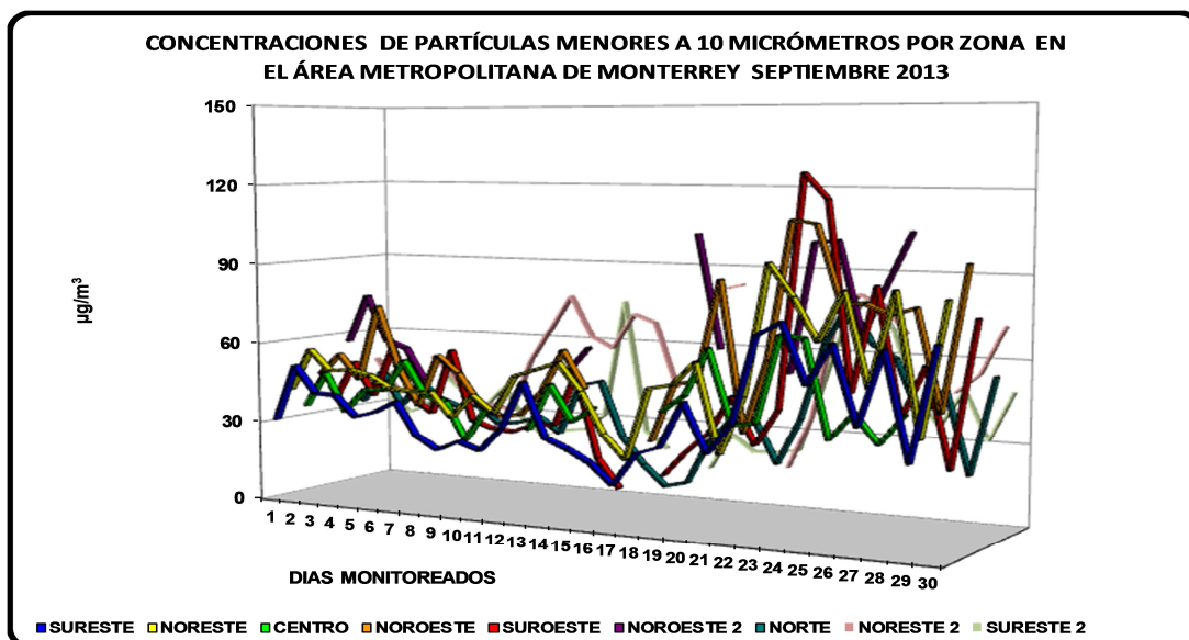
Figura 19: Promedio de concentración diaria de PM 10 por zona en el AMM
