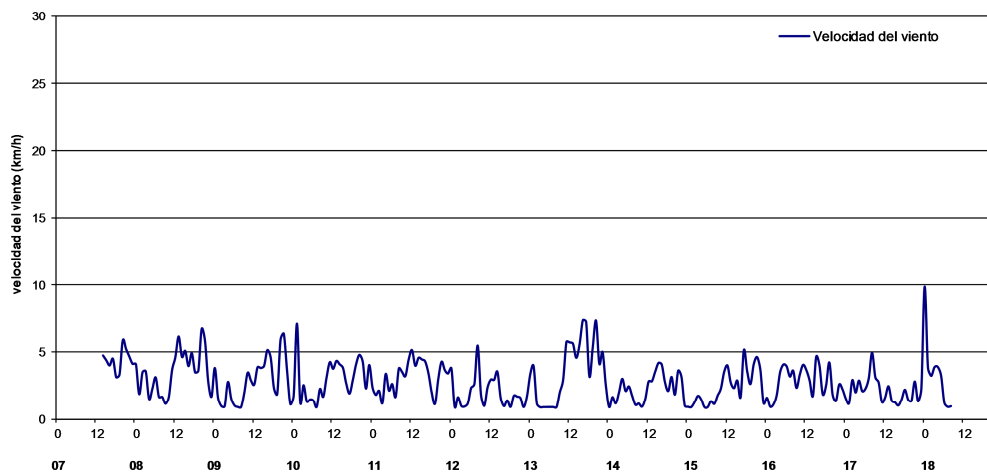
Figura 12. Velocidad del viento.
