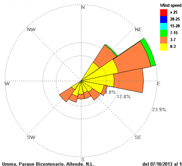
Figura 13. Rosa de vientos durante el monitoreo atmosférico realizado en el Parque Bicentenario en Allende, N.L.
