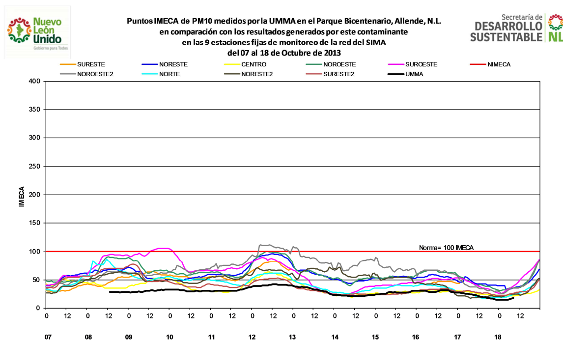
Figura 6. Puntos IMECA de Partículas menores a 10 micrómetros.
