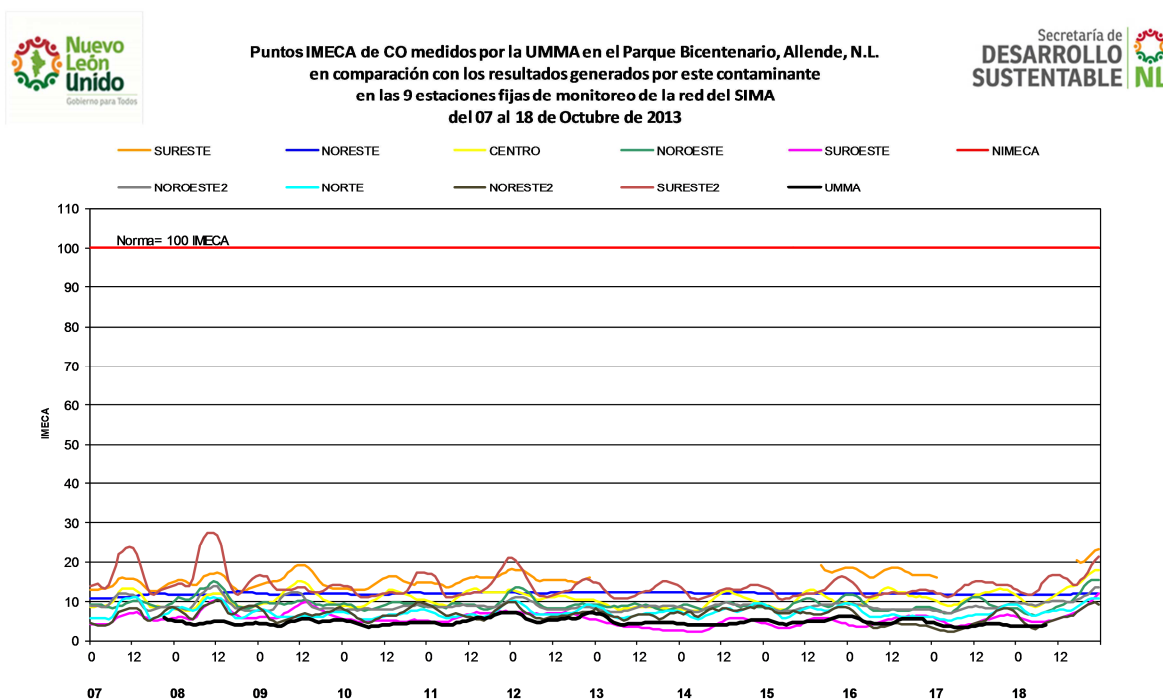
Figura 2. Puntos IMECA de Monóxido de Carbono.
