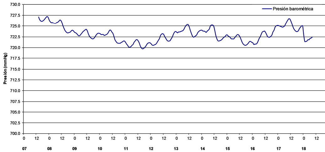
Figura 10. Presión barométrica.
