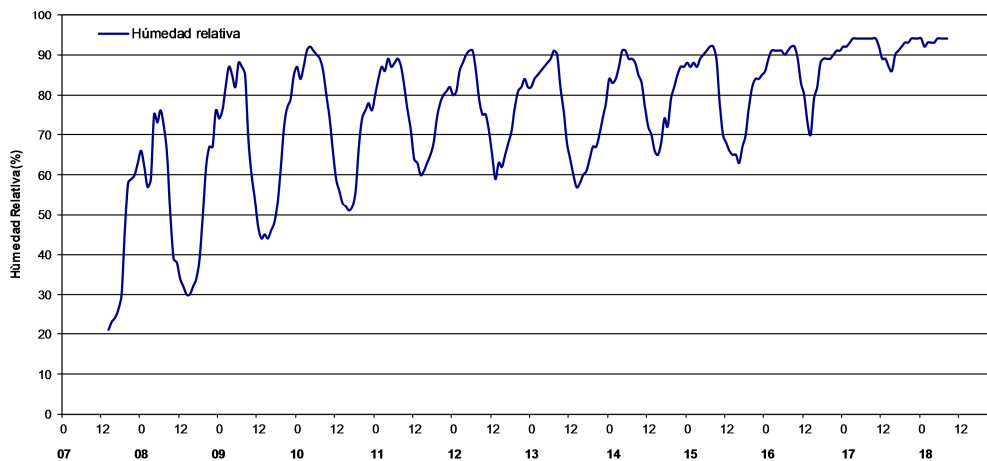
Figura 11. Humedad relativa.
