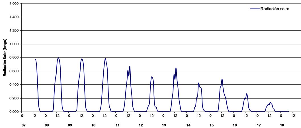
Figura 9. Radiación solar.
